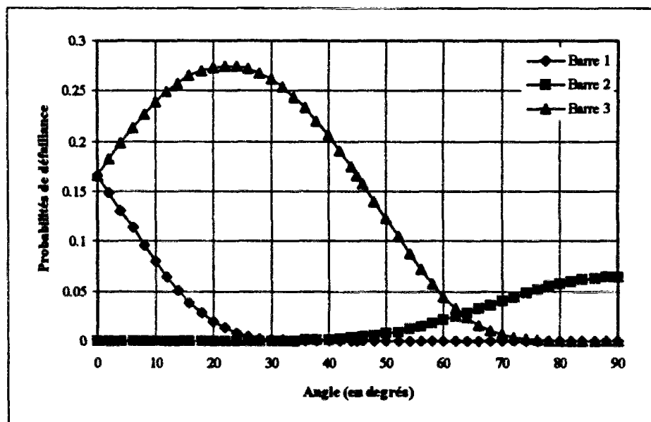
Figure V.4 : Evolution des probabilités de défaillance en fonction des angles de chargements
