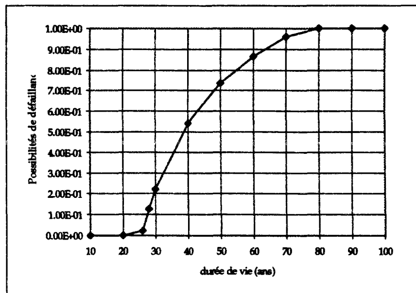
Figure VI.9 : Evolution des possibilités de défaillance en fonction du nombre d'années de service
