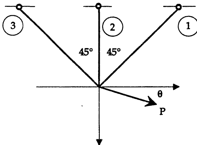
Figure.V.1 : Schéma descriptif de l'exemple de treillis à trois barres
