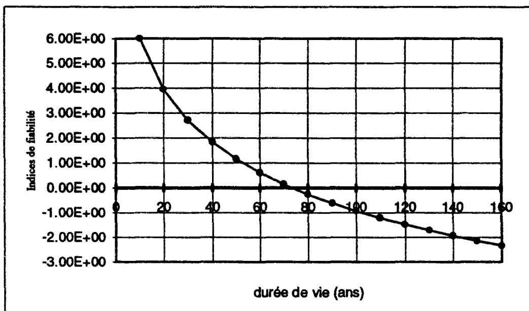
Figure VI.2 : Evolution de l'indice de fiabilité en fonction du nombre d'années de service
