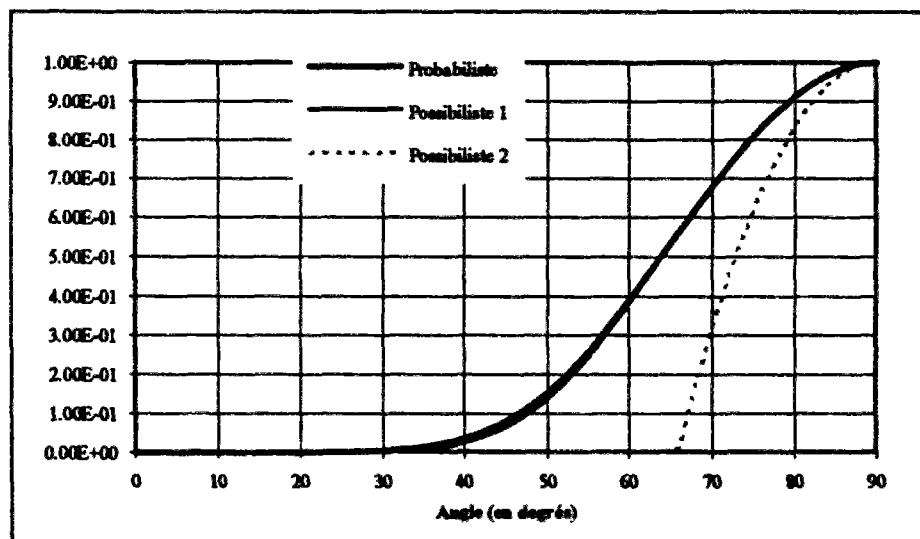
Figure V.11 : Evolution des probabilités et des possibilités de défaillance normalisées pour la barre 2
