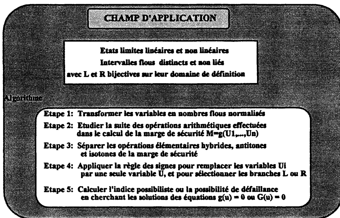
Figure 1.: Champ d'application et démarche générale de l'approche possibiliste de la fiabilité
