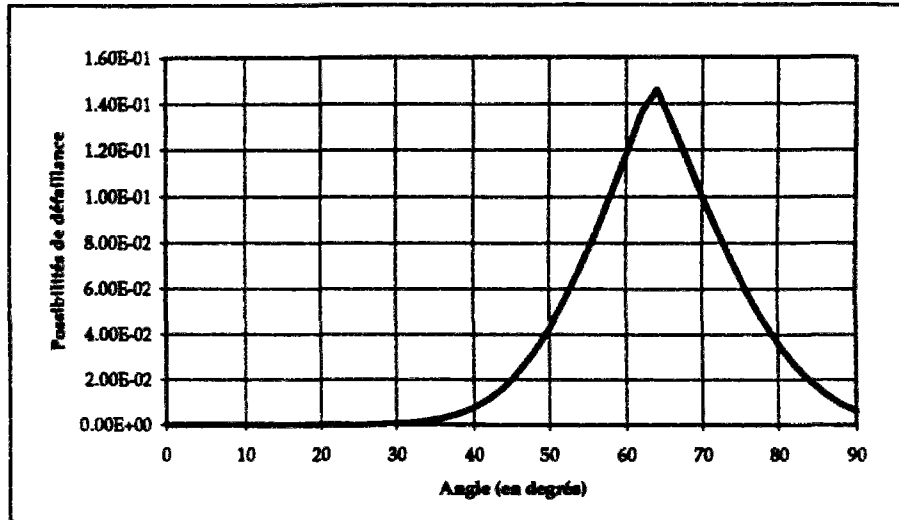
Figure V.18 : Evolutions des possibilités de défaillance du sous-système (2, 3/2) (nombres flous gaussiens)
