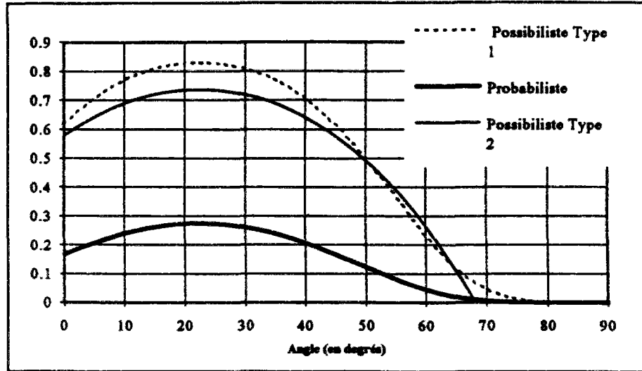
Figure V.9 : Comparaisons entre les possibilités et probabilités de défaillance en fonction des angles de chargements (Barre 3)
