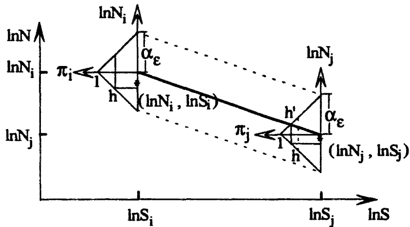
Figure VI.4 : Illustration de la méthode régression possibiliste
