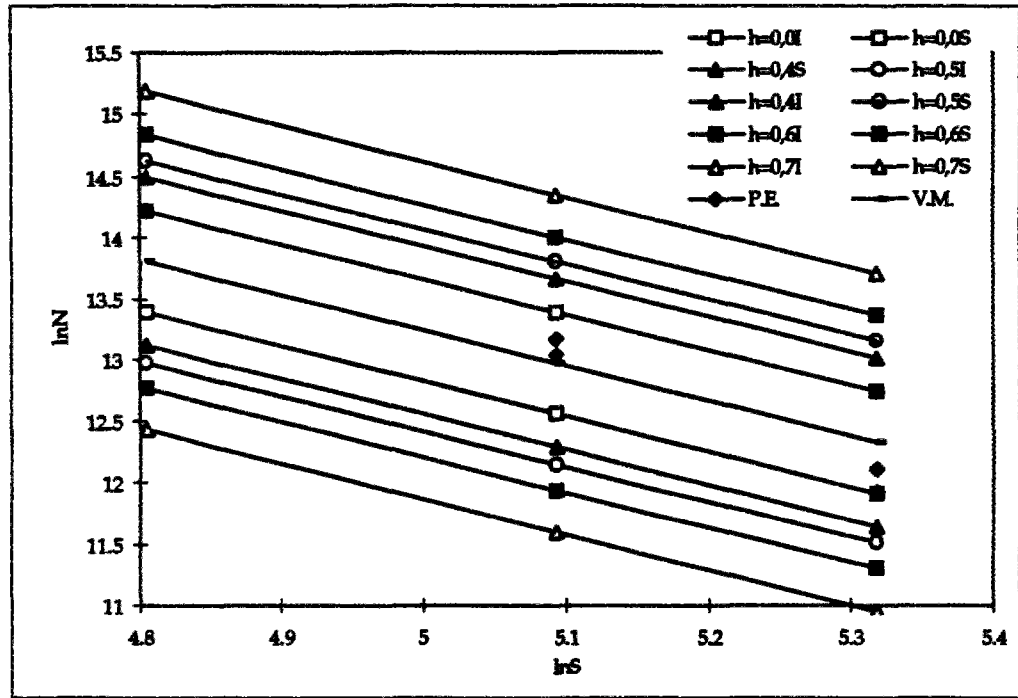
Figure VI.5 : Résultats de la régression possibiliste pour différentes valeurs de h
