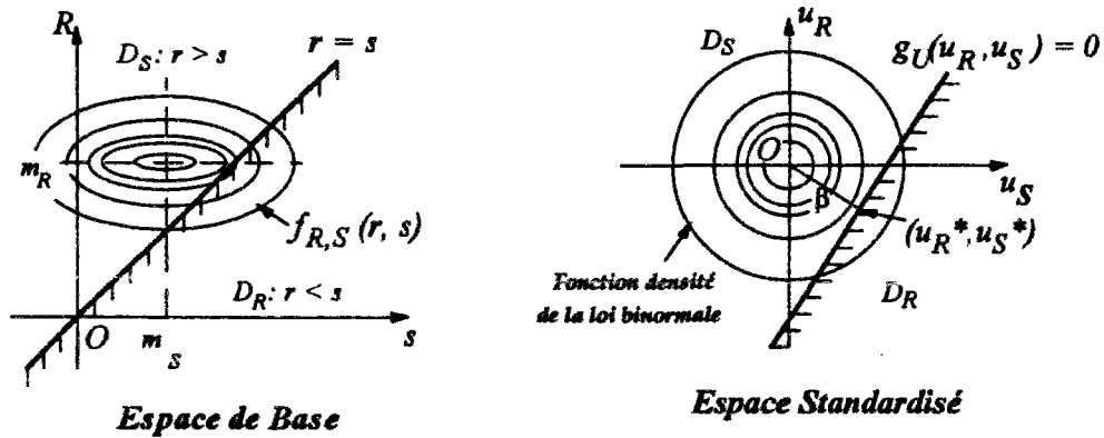
Figure III.1.: Représentations géométriques de l'état limite dans les espaces de base et standardisé et de l'indice de fiabilité \beta
