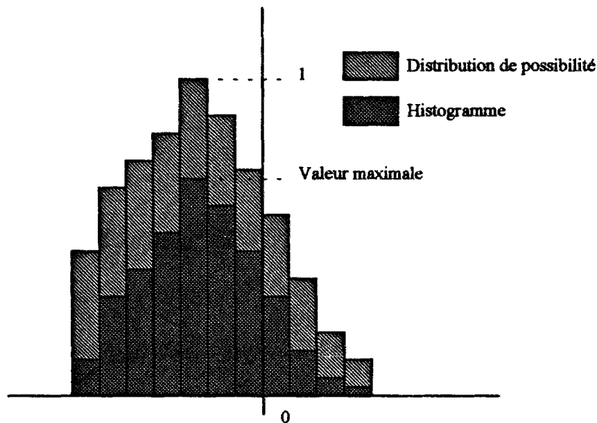
Figure II.1 : Première construction d'une distribution de possibilité à partir d'un histogramme
