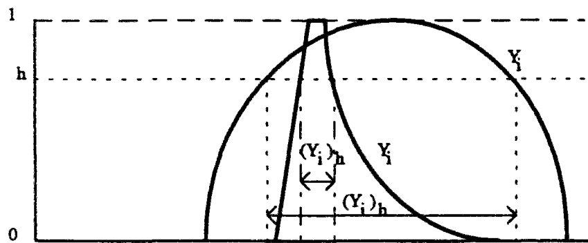
Figure A4.1.: Principe de la régression possibiliste
