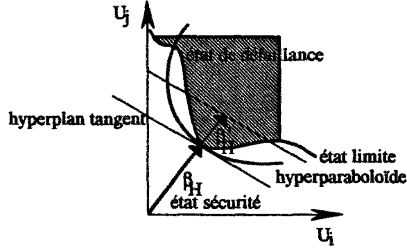
Figure III.3 : Hyperplan et hyperparaboloïde tangents - indice de fiabilité
