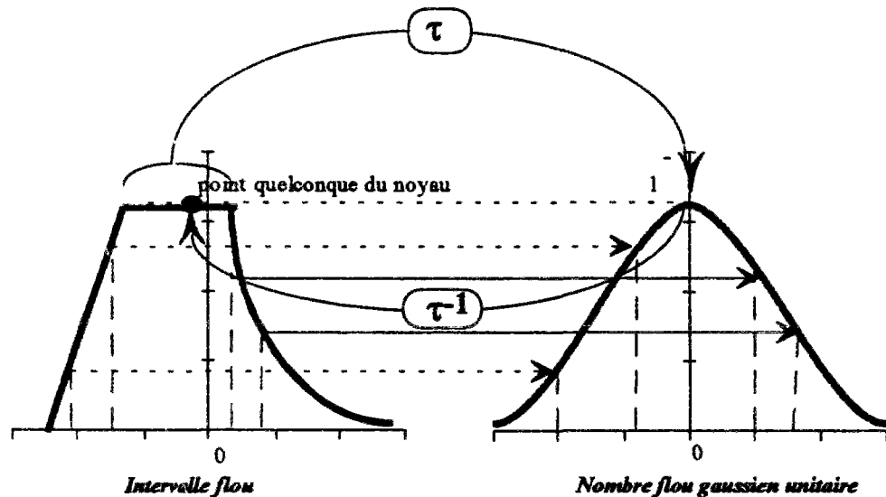
Figure IV.4 : Illustration de la transformée possibiliste
