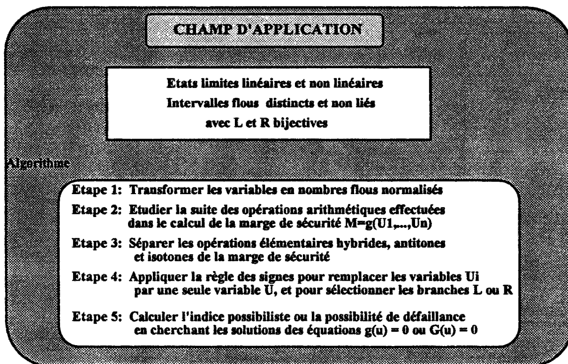
Figure IV.6 : Champ d'application et démarche générale de l'approche possibiliste de la fiabilité
