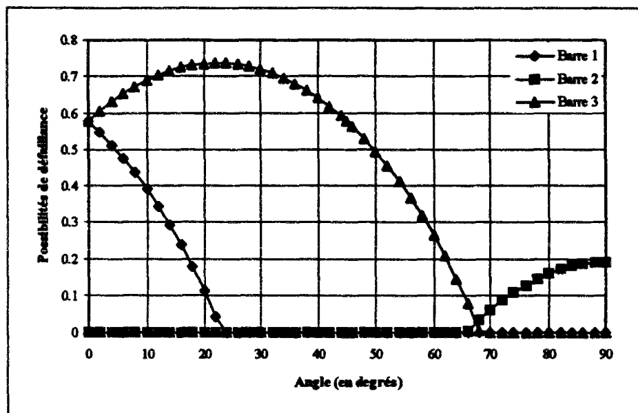
Figure V.8 : Evolution des possibilités de défaillance suivant divers angles de chargement
