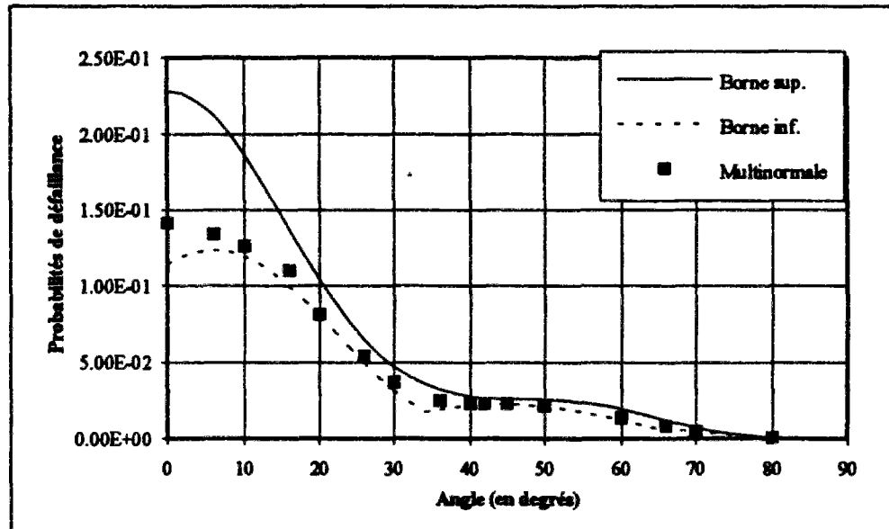
Figure V.20 : Evolution des probabilités de défaillance suivant divers angles de chargement
