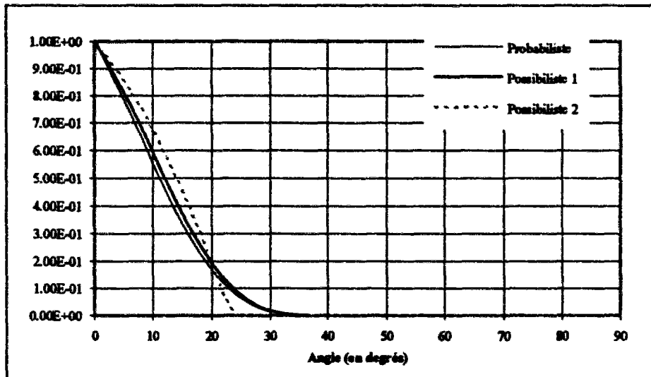
Figure V.10 : Evolution des probabilités et des possibilités de défaillance normalisées pour la barre 1
