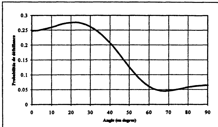
Figure V.13 : Evolution des probabilités de défaillance en fonction des angles de chargement (système en série)
