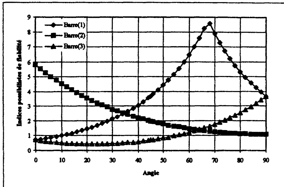
Figure V.5 : Evolution des indices de fiabilité en fonction des angles de chargements
