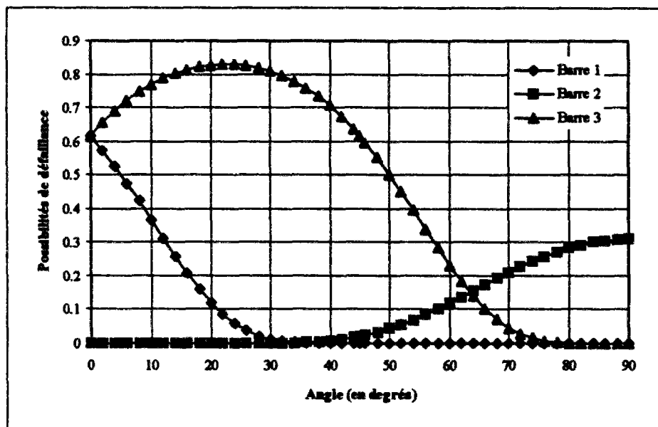
Figure V.6 : Evolution des possibilités de défaillance en fonction des angles de chargements
