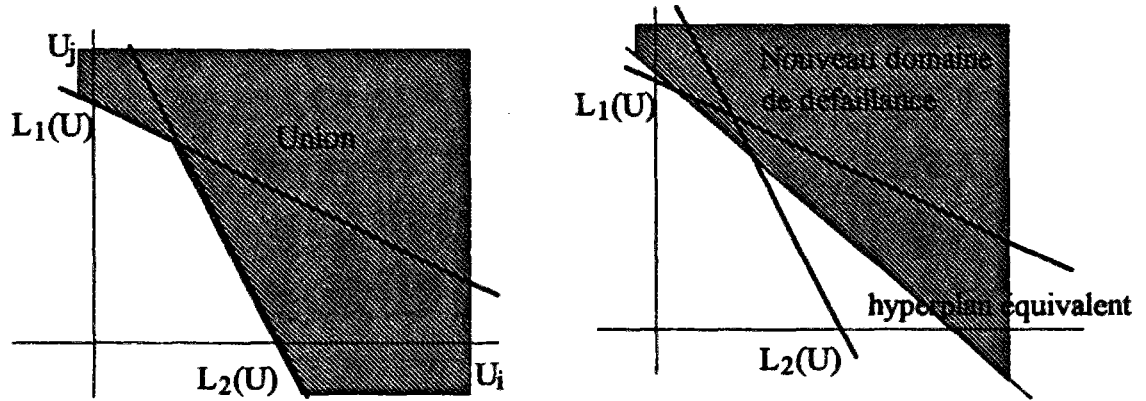
Figure III.4.: Hyperplan équivalent pour le calcul d'unions d'états limites
