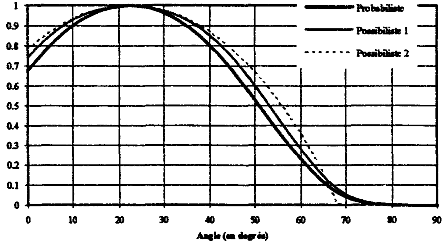
Figure V.12 : Evolution des probabilités et des possibilités de défaillance normalisées pour la barre 3
