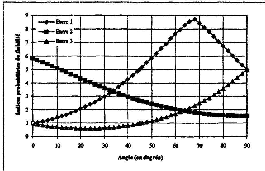
Figure V.3 : Evolution des indices probabilistes de fiabilité en fonction des angles de chargements
