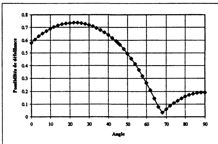
Figure V.15 : Evolution des possibilités de défaillance suivant divers angles de chargement (système en série, nombres flous triangulaires)
