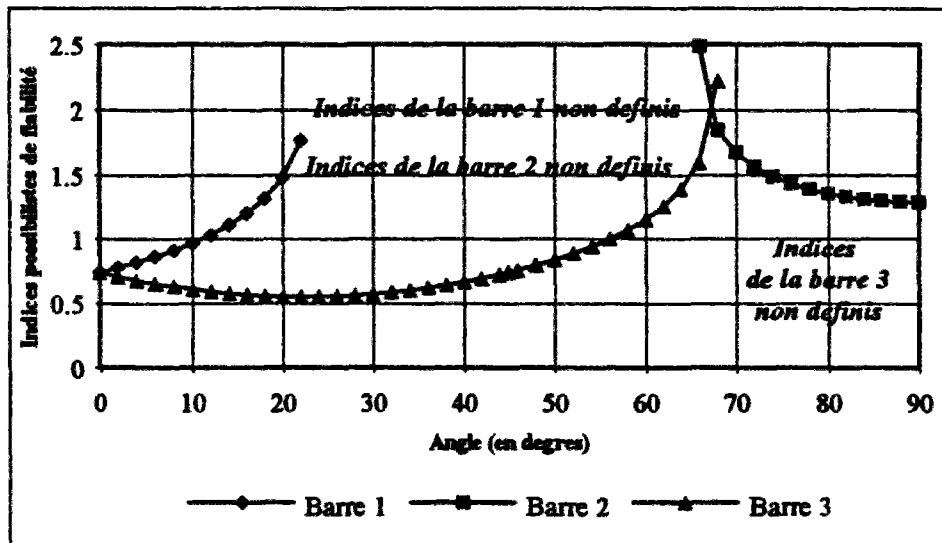
Figure V.7 : Evolution des indices possibilistes de fiabilité suivant divers angles de chargement
