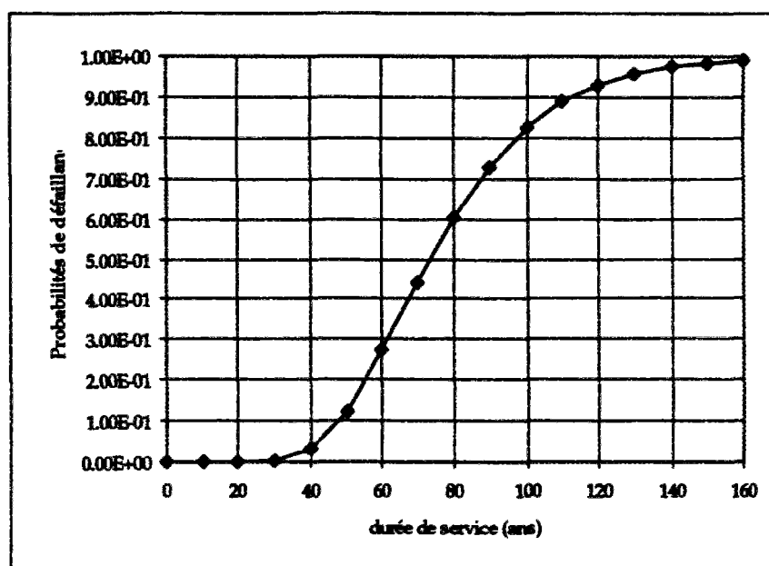
Figure VL3 : Evolution de la probabilité de défaillance en fonction du nombre d'années de service
