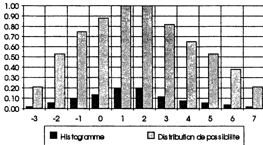
Figure II.2 : Exemple de construction d'une distribution de possibilité à partir d'un histogramme ordonné
