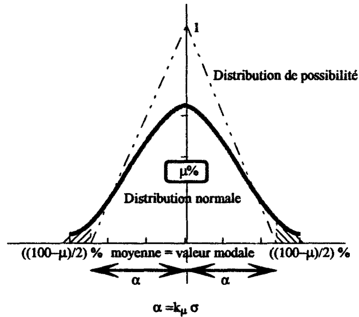
Figure II.3 : Distribution possibiliste triangulaire construite à partir d'une variable gaussienne
