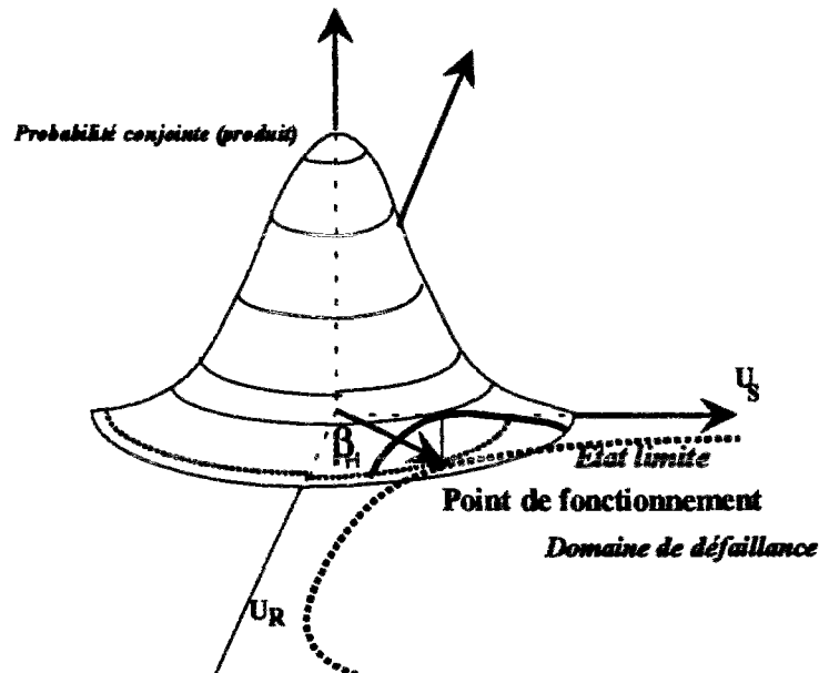
Figure III.2 : Représentation de l'indice de fiabilité
