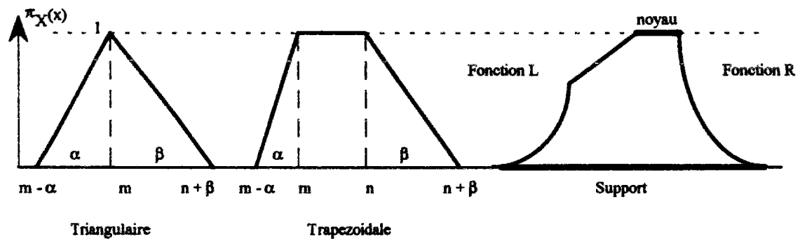
Figure IV.1 : Nombre flou - Intervalle flou - Quantité floue
