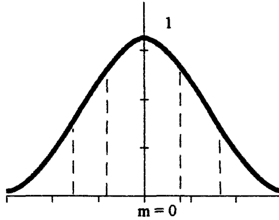
Figure IV.2 : Nombre flou gaussien
