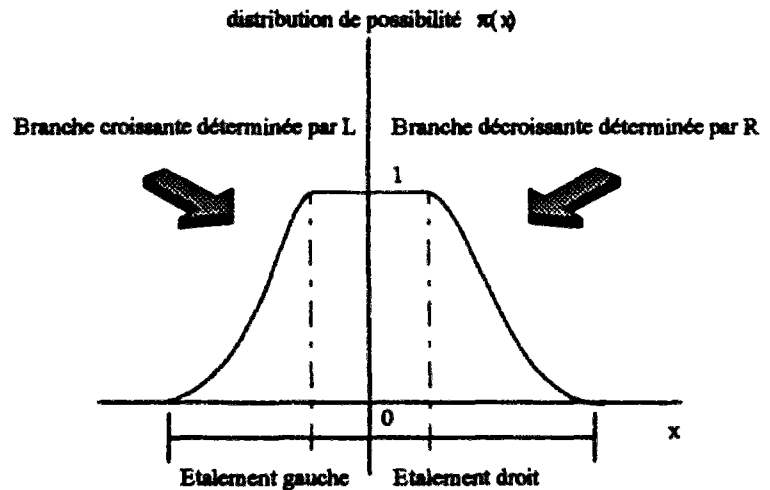
Figure 1: Fonctions de forme L et R
