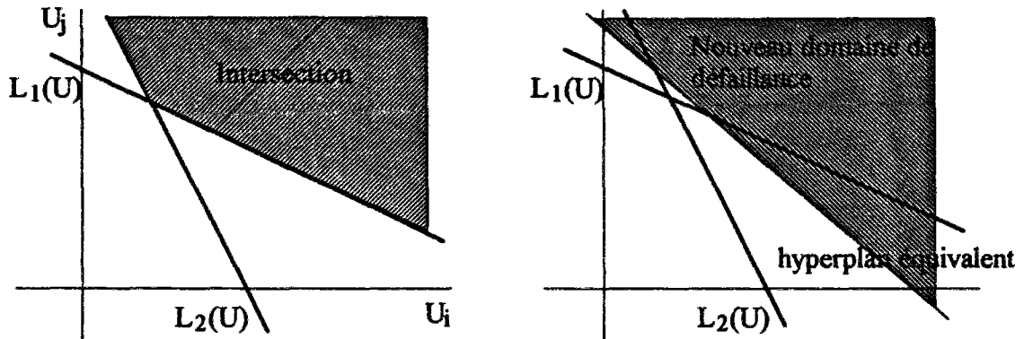
Figure III.5.: Hyperplan équivalent pour le calcul d'intersections d'états limites
