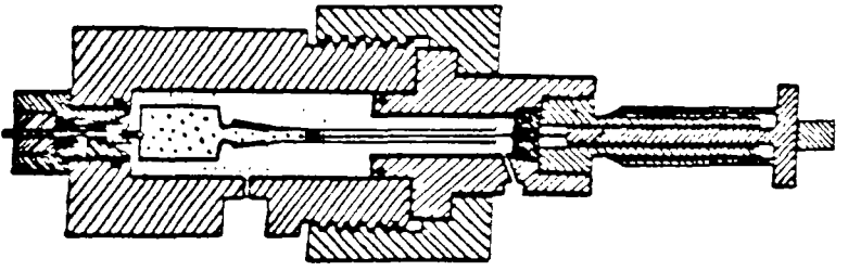
CONFIGURATION N°1 Dilato. 1 + Soude
