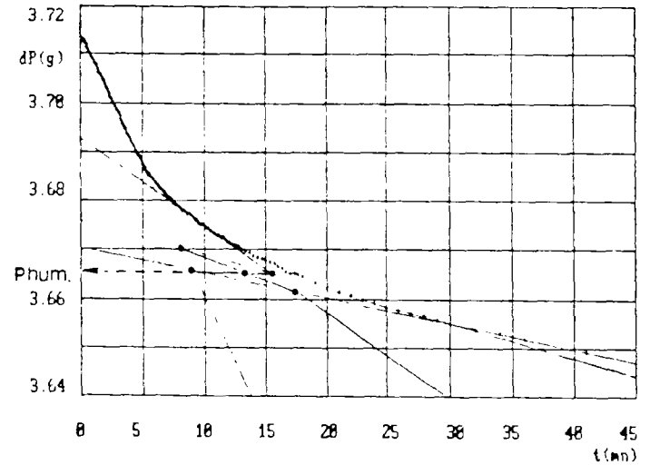
Courbe de séchage de l'échantillon 324.05 Epruvette de diamètre \phi = 10 mm et de hauteur H = 20 mm
