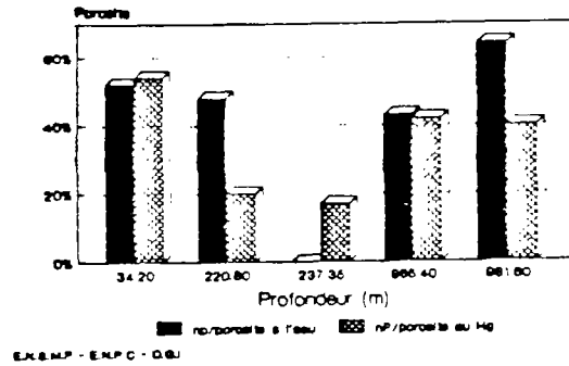
COMPARAISON DE LA POROSITE PIEGEE AVEC LA POROSITE DE PORES
