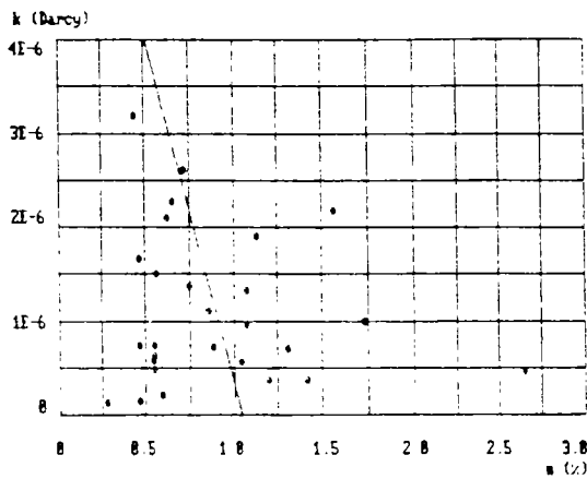
FIG.6.4 : relation entre la perméabilité k et la porosité totale à l'eau n .
