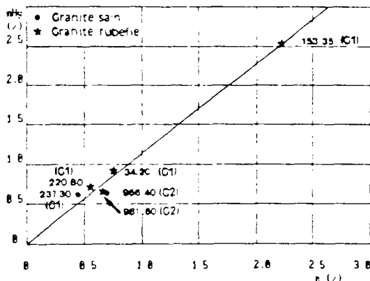
FIG.5.23 : relation entre la porosité totale à l'eau (n) et la porosité au mercure (nHg)
