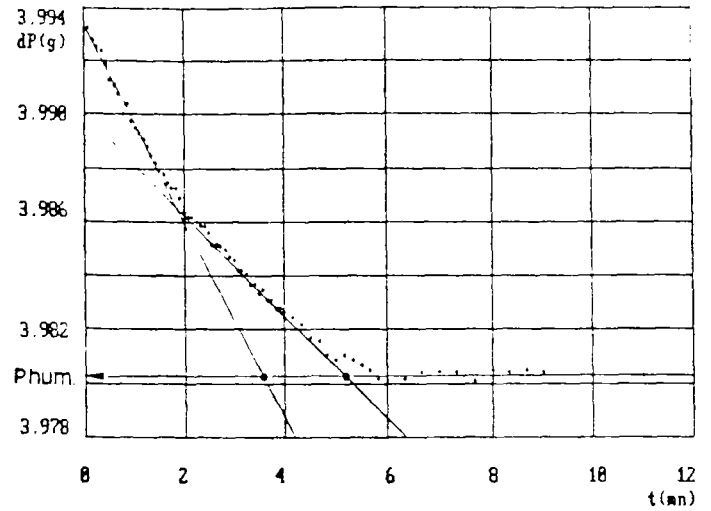
Courbe de séchage de l'échantillon 699.12 Epruvette de diamètre \phi = 10 mm et de hauteur H = 20 mm
