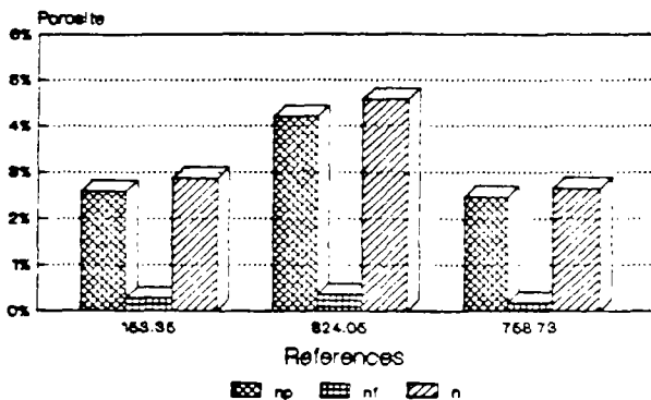
Granite rubefie a forte porosite ( n > 2 ) Decomposition de n en n_f et n_p a partir d' I_{qsec}
