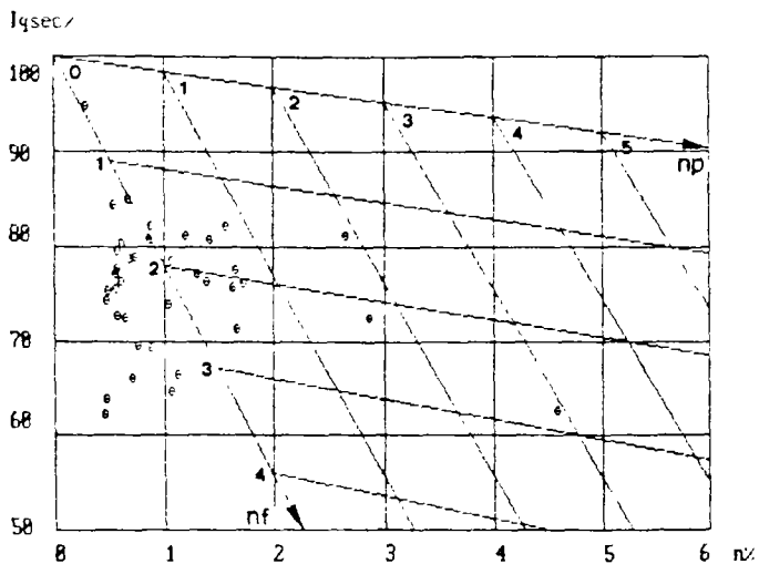
Décomposition de la porosité totale du granite d'Auriat, en porosité de pores et en porosité de fissures, d'après les coefficients déterminés par C.TOURENOQ, D.FOURMAINTRALUX, A.DENIS (1971).
