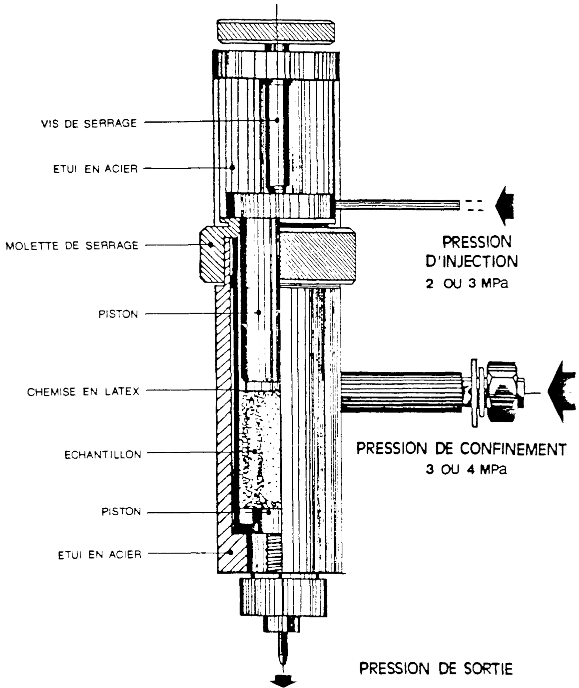
FIG.6.2: SCHEMA D'UNE CELLULE « HASSLER »
