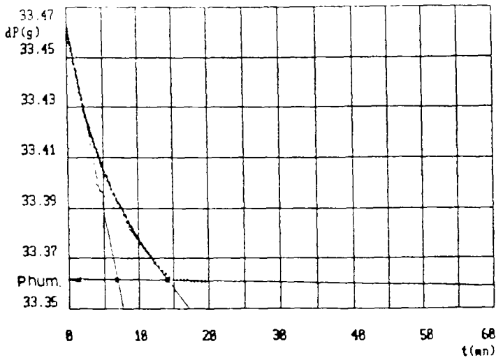
Courbe de séchage de l'échantillon 699.12 Eprouvette de diamètre \phi = 20 mm et de hauteur H = 40 mm
