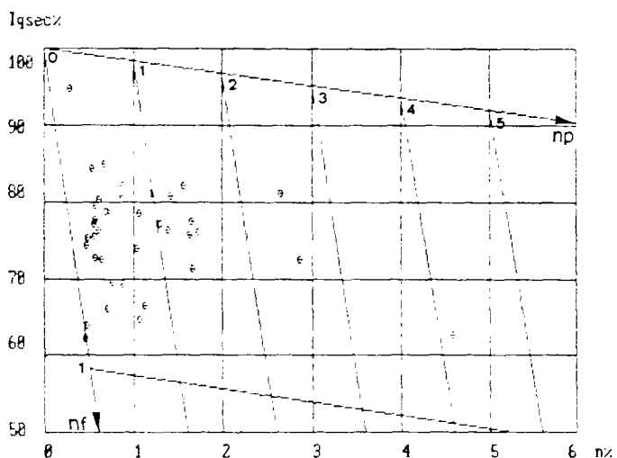
Décomposition de la porosité totale du granite d'Auriat, en porosité de pores et en porosité de fissures, d'après les coefficients déterminés à partir du sondage.
