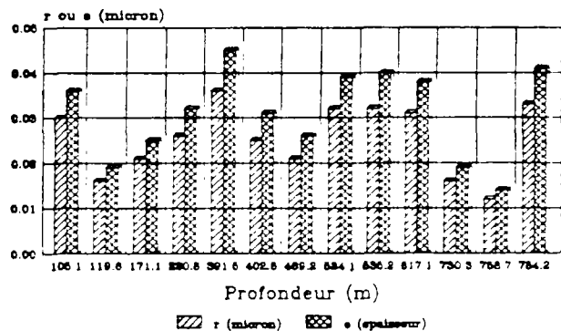
FIG.6.9 : relation entre les rayons moyens et d'accès aux pores, les épaisseurs moyennes des microfissures et les faciès d'altération.
