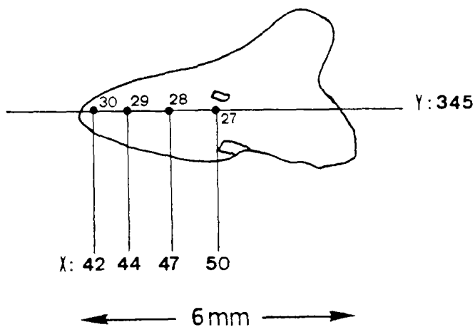
FIG. 2.16: ECH. 825.84. MINERAL B. LOCALISATION DES POINTS D'ANALYSE PRINCIPAUX RESULTATS. Granite très rubéfié
