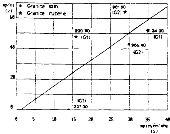
FIG.5.24 : relation entre la porosité de pore (np) et la porosité piégée (npiégée).
