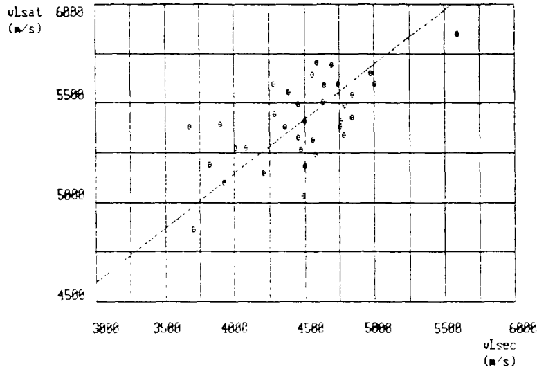
Relation entre v_{Lsec} et v_{Lsat}
