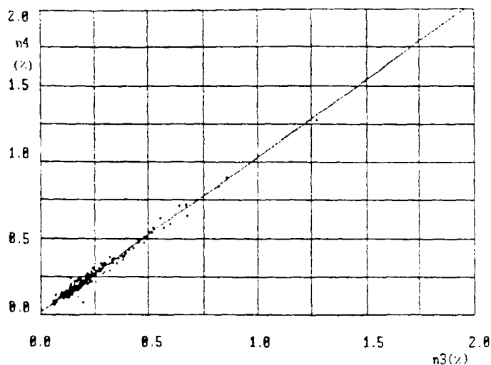
Relation entre les séries de mesure de porosité où le poids humide est déterminé après essuyage avec un papier absorbant sec. n3 : essuyage avec un papier hygiénique "doux". n4 : essuyage avec un papier hygiénique "dur". Eprouvettes de diamètre \phi = 10 mm et de hauteur H = 20 mm.
