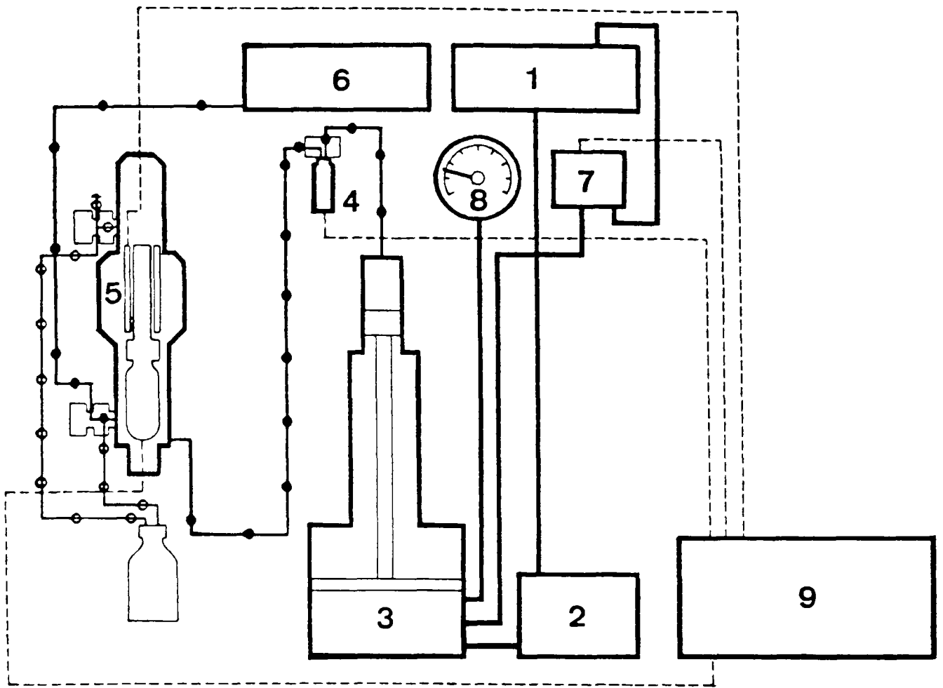
FIG.5.2: Schéma de principe du porosimètre CARLO.ERBA 2000 WS (1984)
