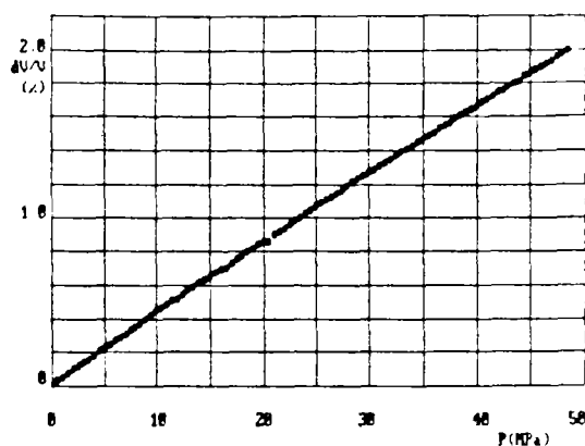
FIG 519 dV/V/P ABSOLU DE NaOH 10 -2 N
