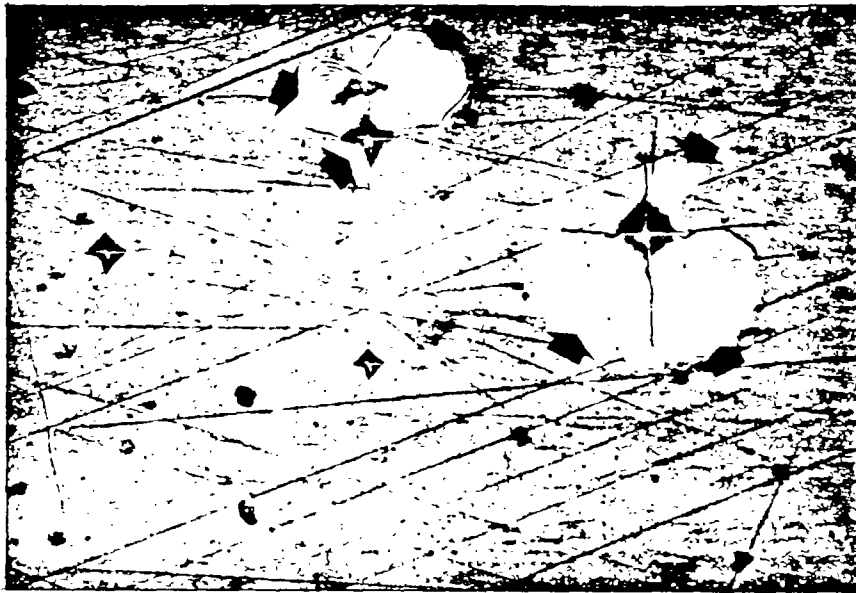
FIG.3.4 : Empreintes de Vickers sur une surface de verre. Ecailles à la surface pour les charges de 100 à 50 p (p : pond ; 1 pond \leftrightarrow 1 g), et petits éclats pour les charges plus faibles. Verre Schott SFS 1 (d'après notice LEITZ).
