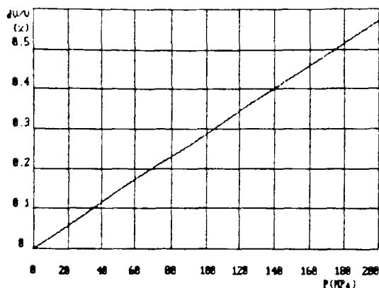
FIG 518 dV/V/P DU DILATOMÈTRE EN PYREX
