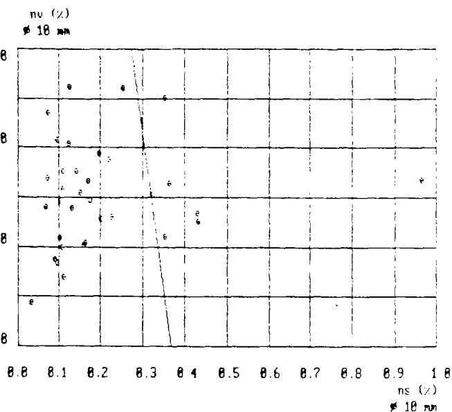
Relation entre les porosités calculées à partir de VL et déterminées à partir des courbes de séchage (éprouvettes \phi = 10 \text{ mm} ; H = 20 \text{ mm} )
