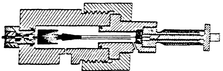
CONFIGURATION N°4 Dilato. 3 + Mercure
