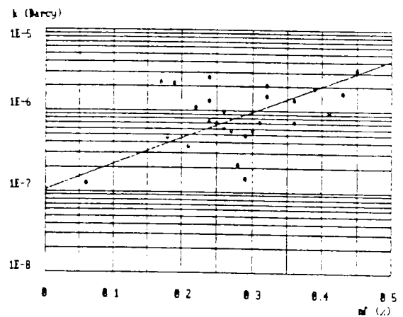
FIG.6.5 : relation entre la perméabilité k et la porosité de fissure n_f
