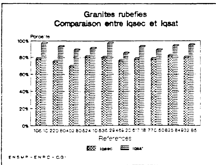
Comparaison des indices de qualité I_{qsec} et I_{qat} . Cas du granite rubéfié.
