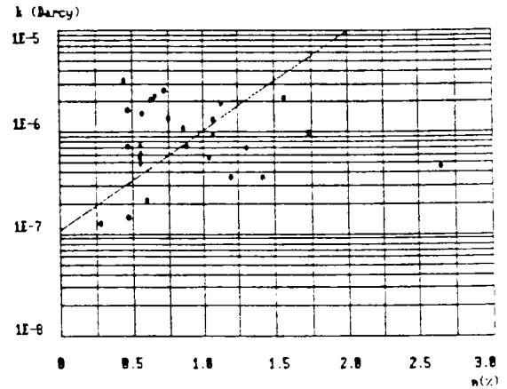
FIG.6.4 : relation entre la perméabilité k et la porosité totale à l'eau n .
