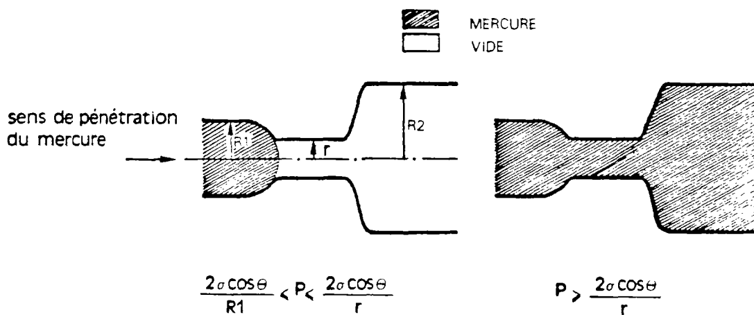
FIG.5.1. Notion schématique de rayon d'accès d'un pore (d'après P.BOUSQUIE, 1979)
