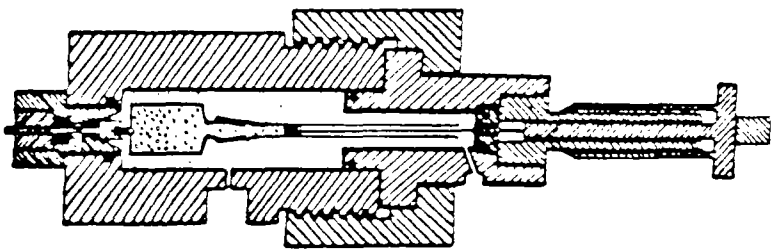
CONFIGURATION N°2b Dilato. 2 + Soude + Billes de verre
