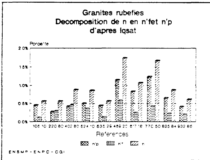
Décomposition de la porosité totale du granite d'Auriat, en porosité de pores et en porosité de fissures, à partir de l'indice de qualité I_{qsat} . Cas du granite rubéfié.
