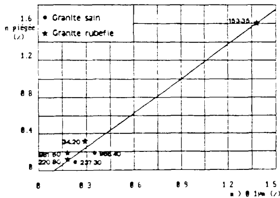
FIG.5.25 : relation entre la macroporosité (n>0.1µm) et la porosité piégée (npiégée)
