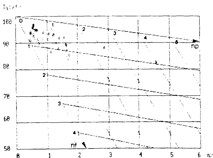
Décomposition de la porosité totale du granite d'Auriat, en porosité de pores et en porosité de fissures, à partir de l'indice de qualité Iq cat
