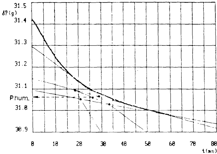
Courbe de séchage de l'échantillon 324.05 Epruvette de diamètre \phi = 20 mm et de hauteur H = 40 mm
