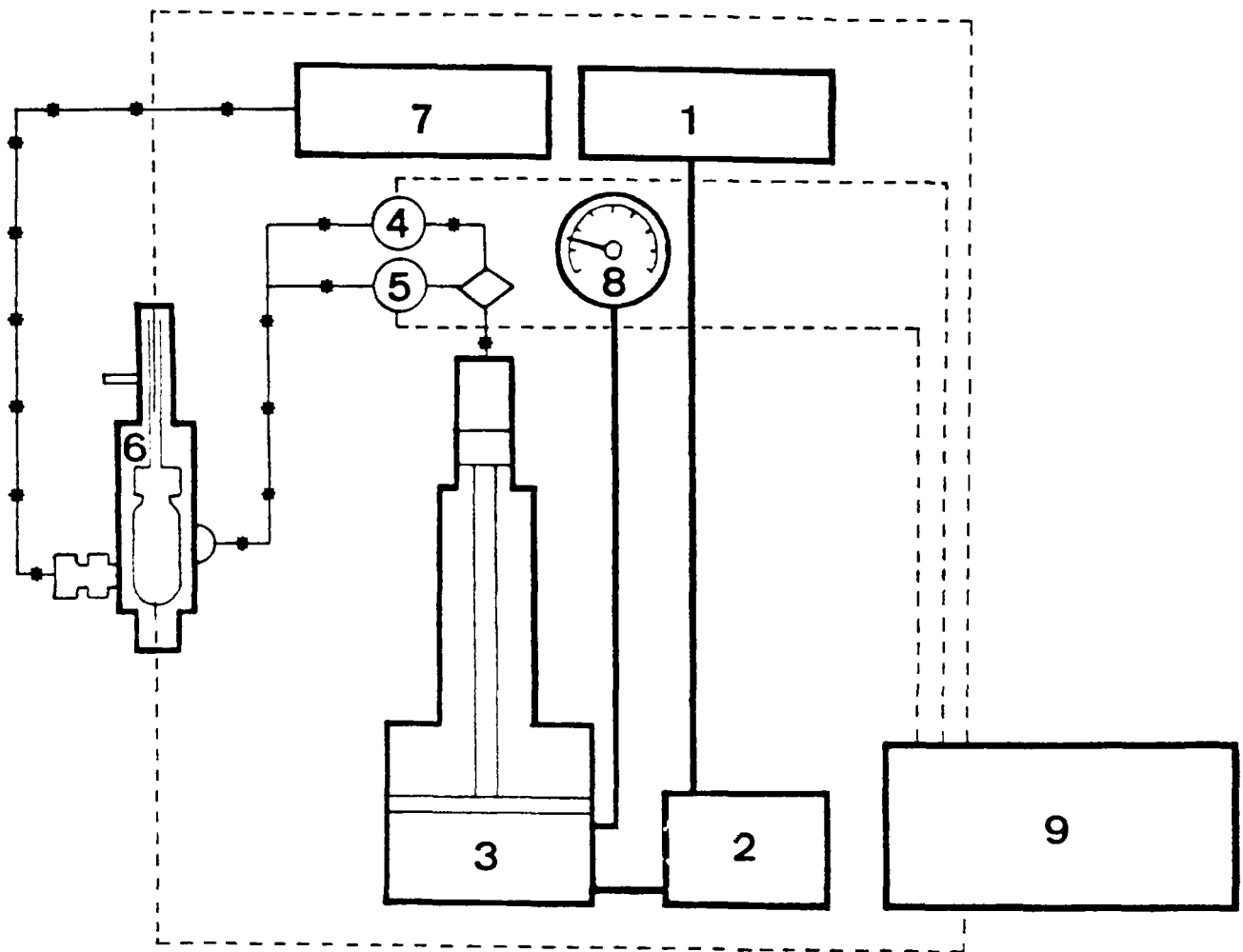
FIG.5.14: Schéma de principe du porosimètre CARLO.ERBA 1500 (1974)
