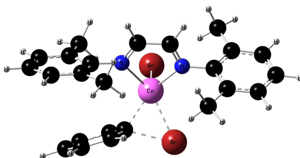
Schéma 72 : état de transition 1.IbTSlIb en triplet
