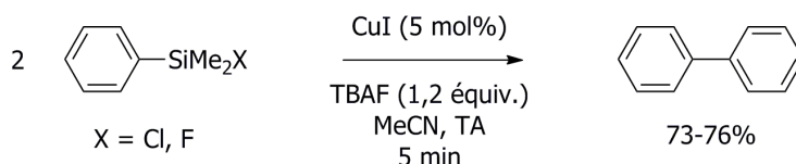
Schéma 15 : dimérisation de dérivés siliciés par catalyse au cuivre
