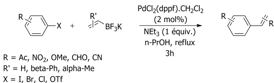
Schéma 123 : vinylation de composés aromatiques par des trifluoroborates (G. Molander)
