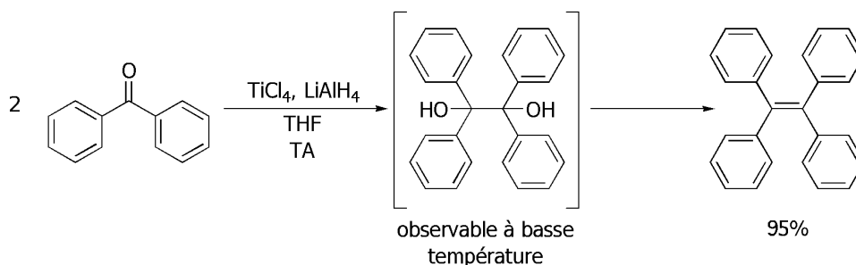
Schéma 104 : principe de la réaction de McMurry
