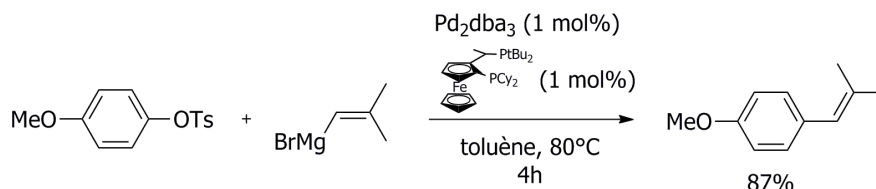
Schéma 122 : vinylation de tosylates aromatiques par des organomagnésiens vinyliques
