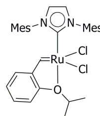
catalyseur de Hoveyda-Grubbs seconde génération
