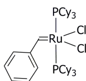
catalyseur de Grubbs première génération
