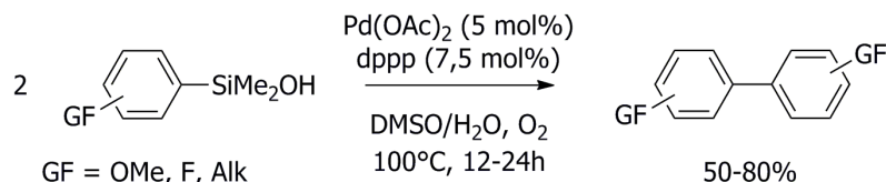
Schéma 30 : dimérisation d'organosiliciés par catalyse au palladium
