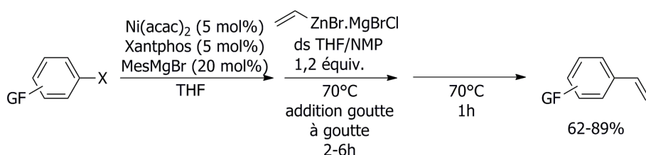
Schéma 130 : Coupplages de vinylzinciques avec des halogénures aromatiques
