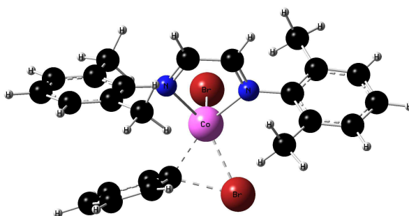
Schéma 72 : état de transition 1.IbT5Iib en triplet
