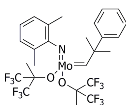
catalyseur de Schrock
