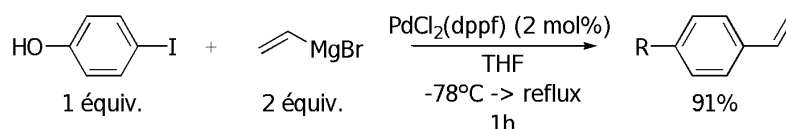
Schéma 121 : vinylation d'iodures aromatiques par des organomagnésiens vinyliques
