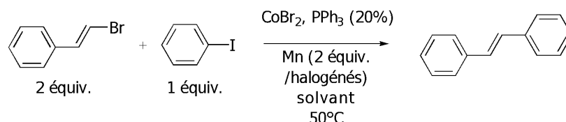
Schéma 149 : étude de l'influence du solvant sur la réaction de vinylation
