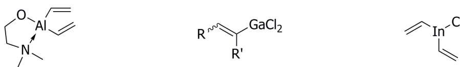
Schéma 128 : exemples d'organométalliques vinyliques couplés par du palladium
