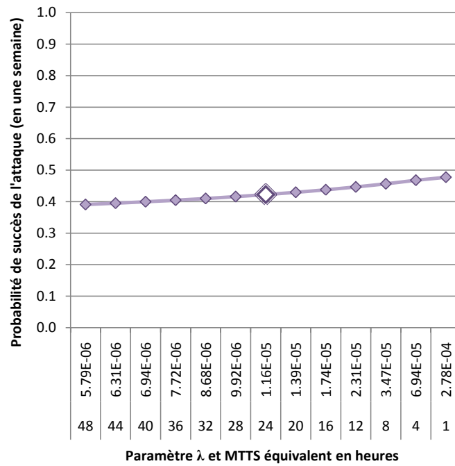
FIGURE III.21 – Incidence du paramétrage de la feuille Reconnaissance générique sur P_s
