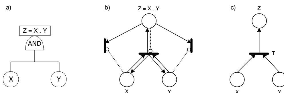
FIGURE III.28 – Modélisation comparée d'un ET logique en BDMP et en réseau de Petri
