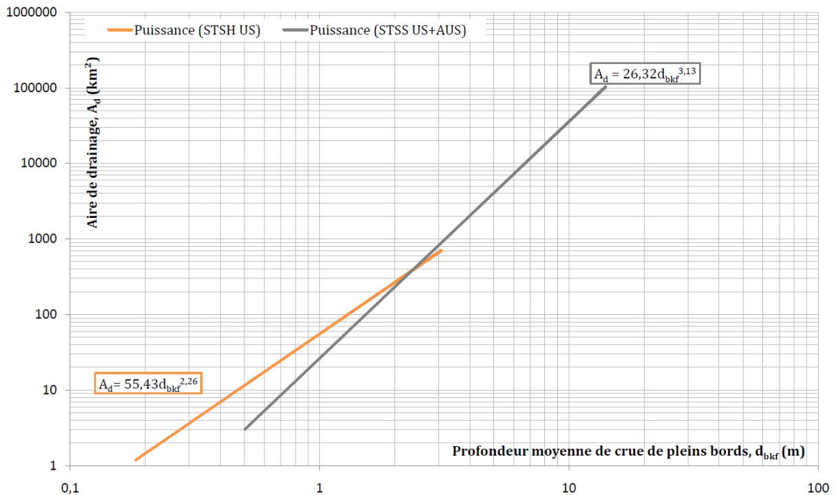
Figure 5-24 : Comparaisons des relations Aire de drainage / Profondeur des domaines subtropicaux semi-humides (STSH) et à saisons sèches (STSS).
