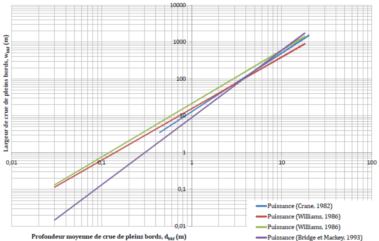
Figure 5-5 : Largeur de crue de pleins bords en fonction de la profondeur moyenne de crue de pleins bords exprimée en fonction des équations présentées dans le Tableau 5-1.
