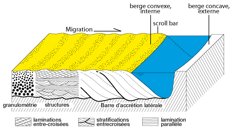
Figure 1-17 : Schéma illustrant l'architecture, les structures sédimentaires et l'évolution granulométrique d'une barre de méandre (d'après Allen, 1985).
