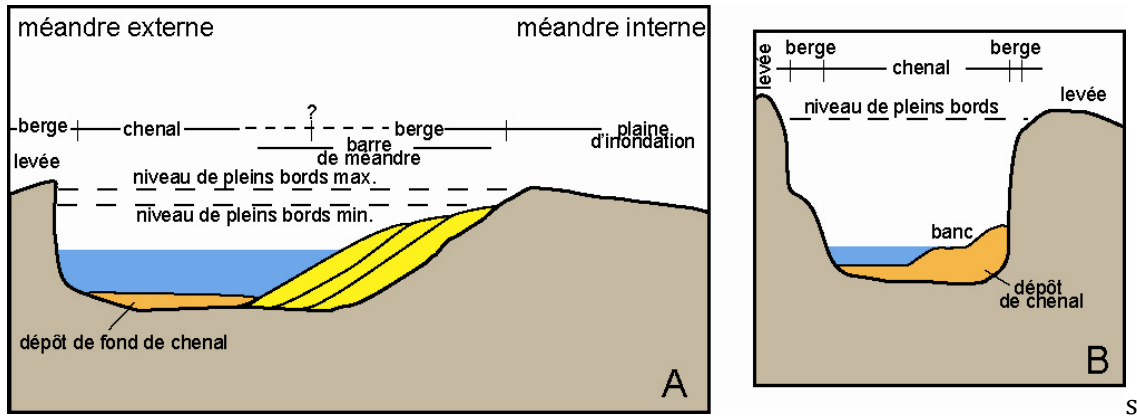
Figure 1-10 : Représentation schématique des géométries mesurées. A : section à l'apex d'un méandre et B : section dans une portion droite. La largeur de pleins bords peut être déterminée à partir des ruptures de pente des berges. Des mesures de l'élévation du lit du chenal berge à berge, permet de définir une aire de section, à partir de laquelle est définie a posteriori une profondeur moyenne de crue de pleins bords (d'après Fitzpatrick et al. , 1998).
