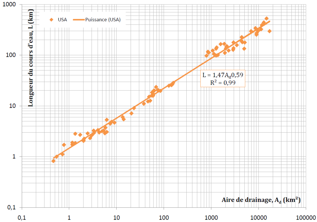
Figure 5-28 : Longueur de chenal ( L ) exprimée en fonction de l'aire de drainage ( A_d ) pour des données de rivières issues du domaine climatique subtropical semi-humide.
