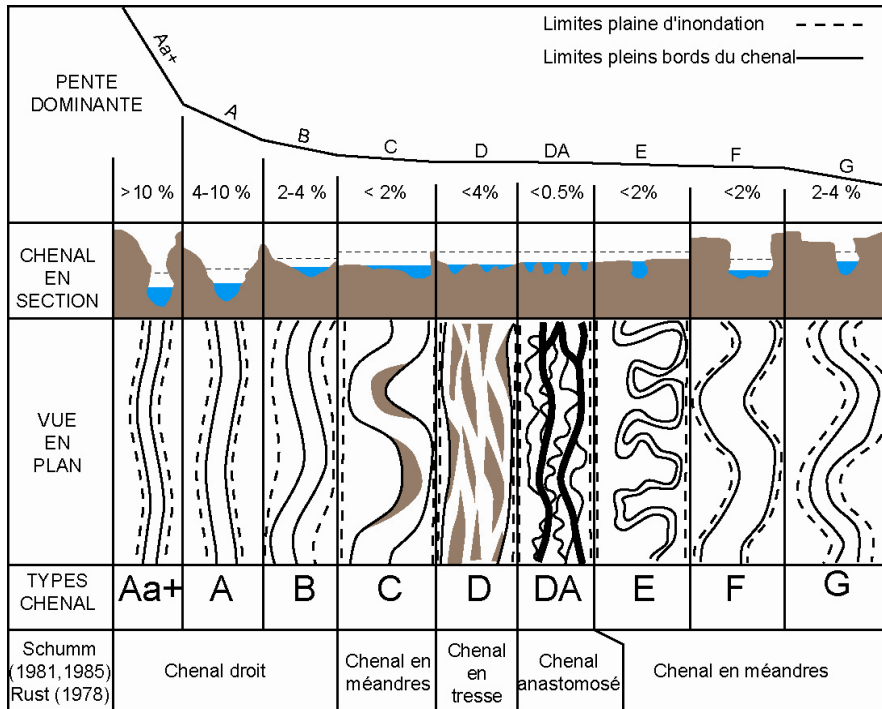
Figure 1-4 : Classification des cours d'eau selon Rosgen (1994) basée sur la section transversale du chenal et la vue en plan reportée à la pente du transect considéré. Cette classification prend en compte les modifications enregistrées par la rivière tout au long de son trajet.
