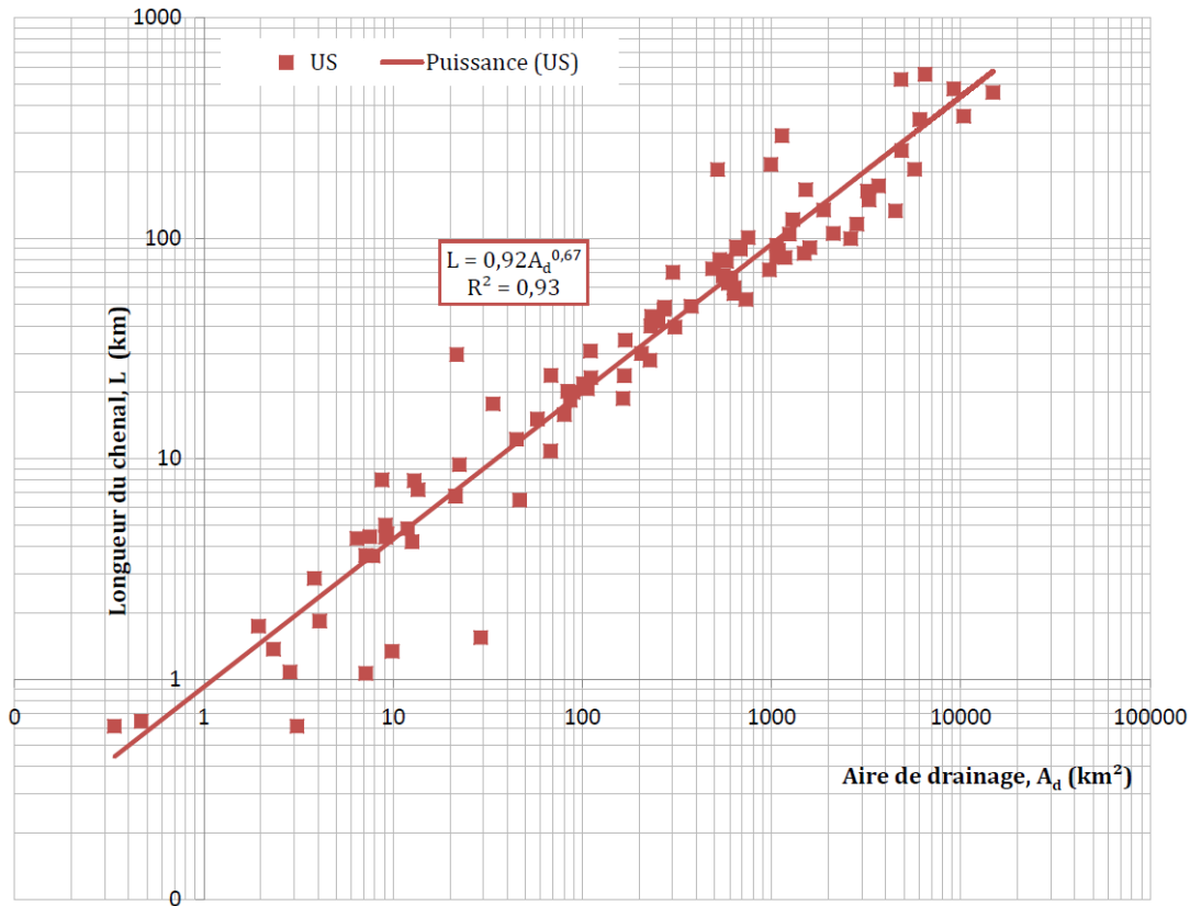
Figure 5-29 : Longueur de chenal ( L ) exprimée en fonction de l'aire de drainage ( A_d ) pour des données de rivières issues du domaine climatique subtropical à saisons sèches.
