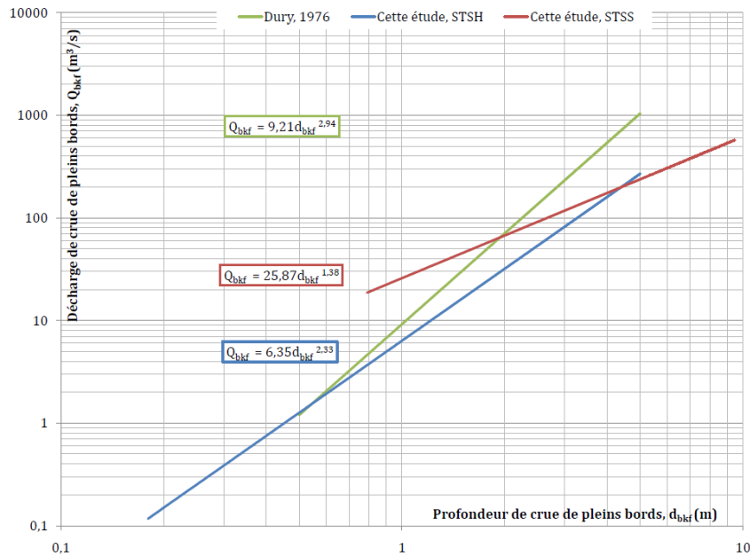
Figure 5-33 : Comparaison des lois entre profondeur de crue de pleins bords et décharge de crue de pleins bords. STSH : Subtropical Semi-Humide et STSS : Subtropical à Saisons Sèches.
