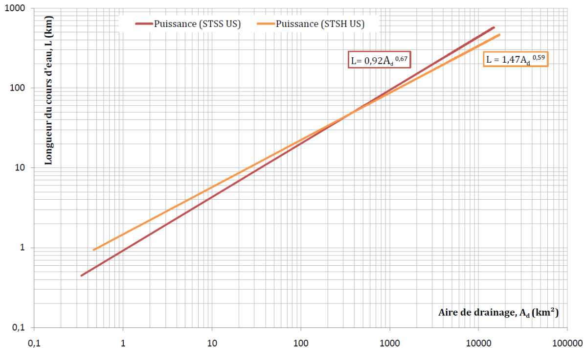
Figure 5-30 : Comparaison des lois entre Longueur de cours d'eau et Aire de bassin versant des domaines subtropicaux semi-humides (STSH) et à saisons sèches (STSS).
