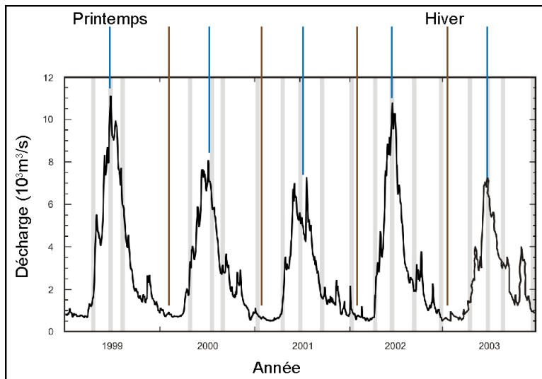
Figure 2-3 : Variations de décharge enregistrées par la rivière Fraser (Canada). Les valeurs maximales pouvant atteindre 1000\text{m}^3/\text{s} sont enregistrées au printemps (traits bleus) et les valeurs minimales pouvant descendre à 300\text{m}^3/\text{s} correspondent aux hivers (traits marron ; www.dfo-mpo.gc.ca ).
