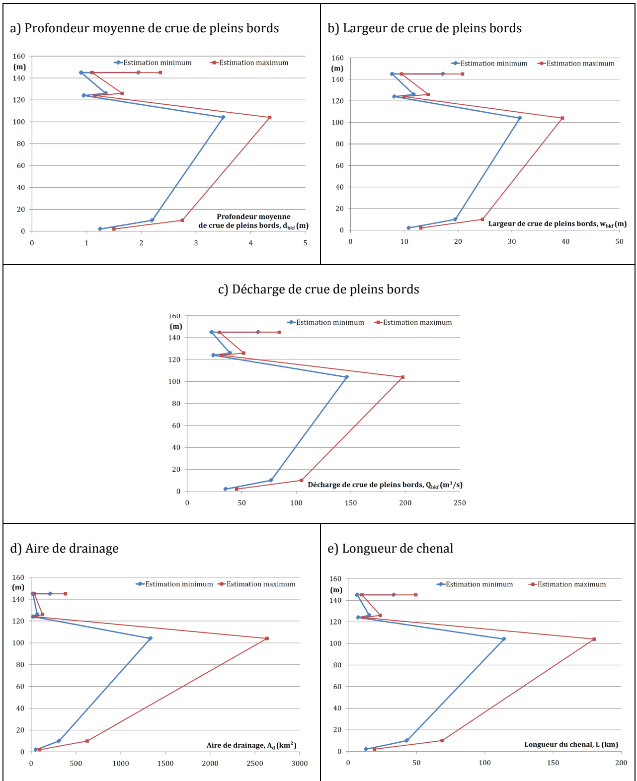
Figure 6-5 : Évolution stratigraphique des paramètres paléohydrologiques calculés pour les barres de méandre de la série du Fan de Tórtola, coupe de Canales (Données chiffrées fournies en Annexe VI d).
