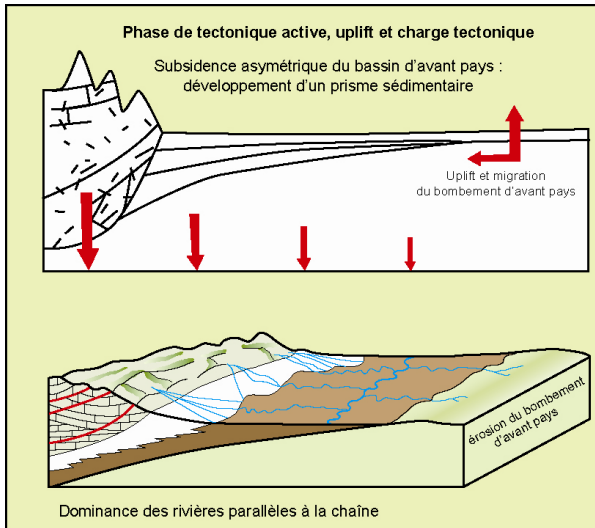
Figure 2-11 : Phase de tectonique active d'un bassin d'avant-pays. Le prisme entraîne la subsidence de l'arrière du bassin et le soulèvement de la partie frontale du chevauchement, dont la migration est orientée vers les zones internes. En réponse, se développent des systèmes fluviaux longitudinaux (d'après Burbank, 1992).
