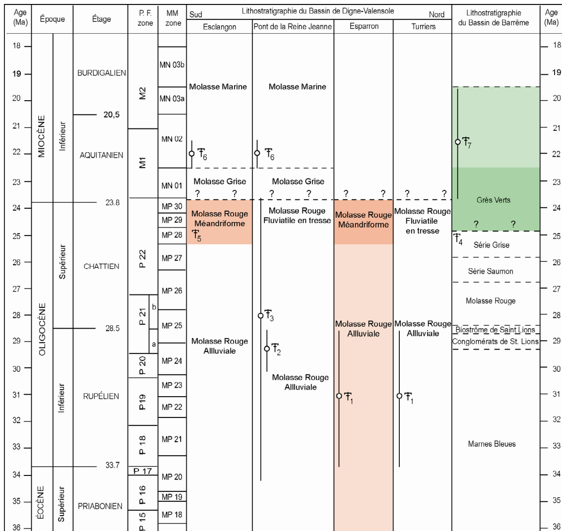
Figure 3-11 : Chronostratigraphie des bassins de Barrême et de Digne du Rupélien supérieur au Burdigalien inférieur. Les séries étudiées sont représentées en vert pour la série des Grès Verts de Barrême et en rouge pour la série de la Molasse Rouge de Digne. Les gisements de micromammifères connus sont indiqués selon l'extension de leur biozone. T 1 : Gisement d'Esparron; T 2 : Gisement du Roucas Blanc ; T 3 : Gisement de Saint-Geniez ; T 4 : Gisements de la Rouvière, la Tuilière et les Blachettes ; T 5 : Gisement du Rousset; T 6 : Gisement de Barles et Lambert ; T 7 : Gisement du Gipas.
