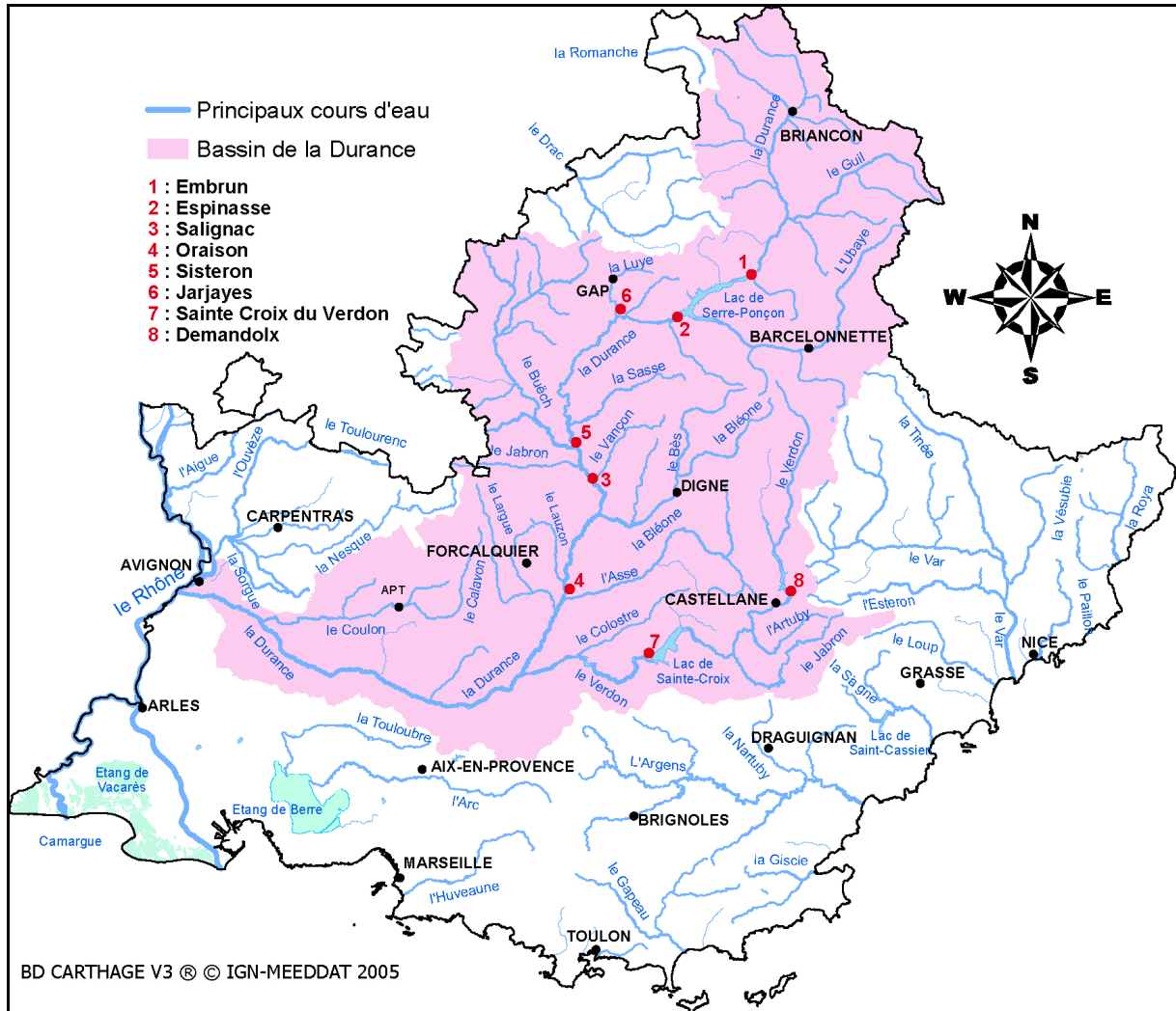
Figure 6-9 : Bassin Versant de la Durance (d'après la base de données de CARTHAGE).
