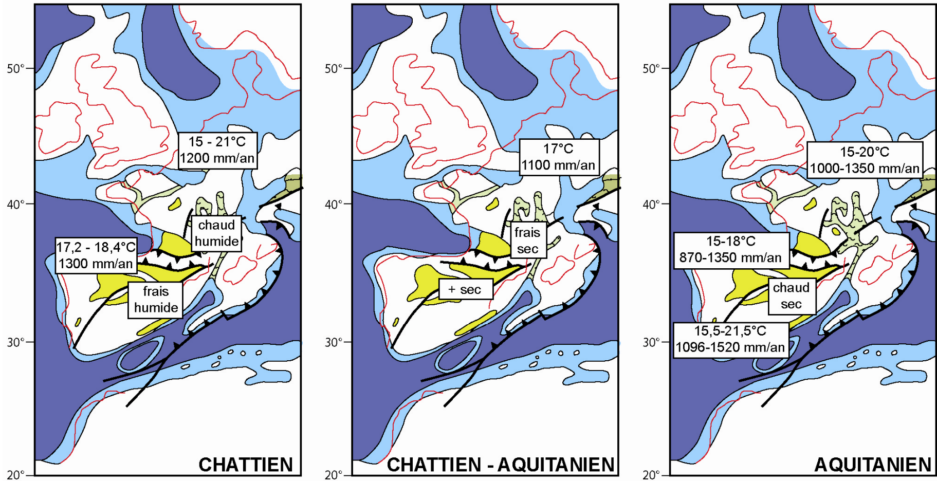
Figure 3-10 : Synthèse des conditions climatiques d'Europe occidentale du Chattien à l'Aquitaniien (basées sur les travaux présentés dans les paragraphes précédents). Pour les légendes des cartes se référer à la Figure 3-1 .
