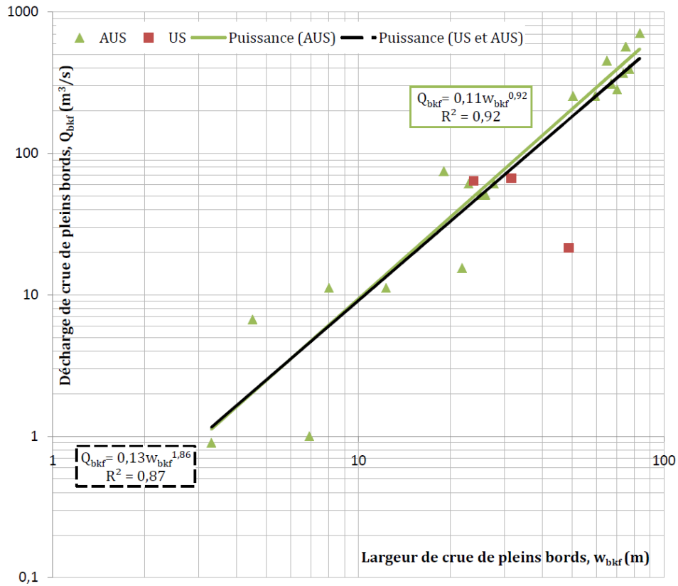
Figure 5-20 : Décharge de crue de pleins bords ( Q_{bkf} ) exprimée en fonction de la largeur de crue de pleins bords ( w_{bkf} ) pour des données de rivières issues du domaine climatique subtropical à saisons sèches.
