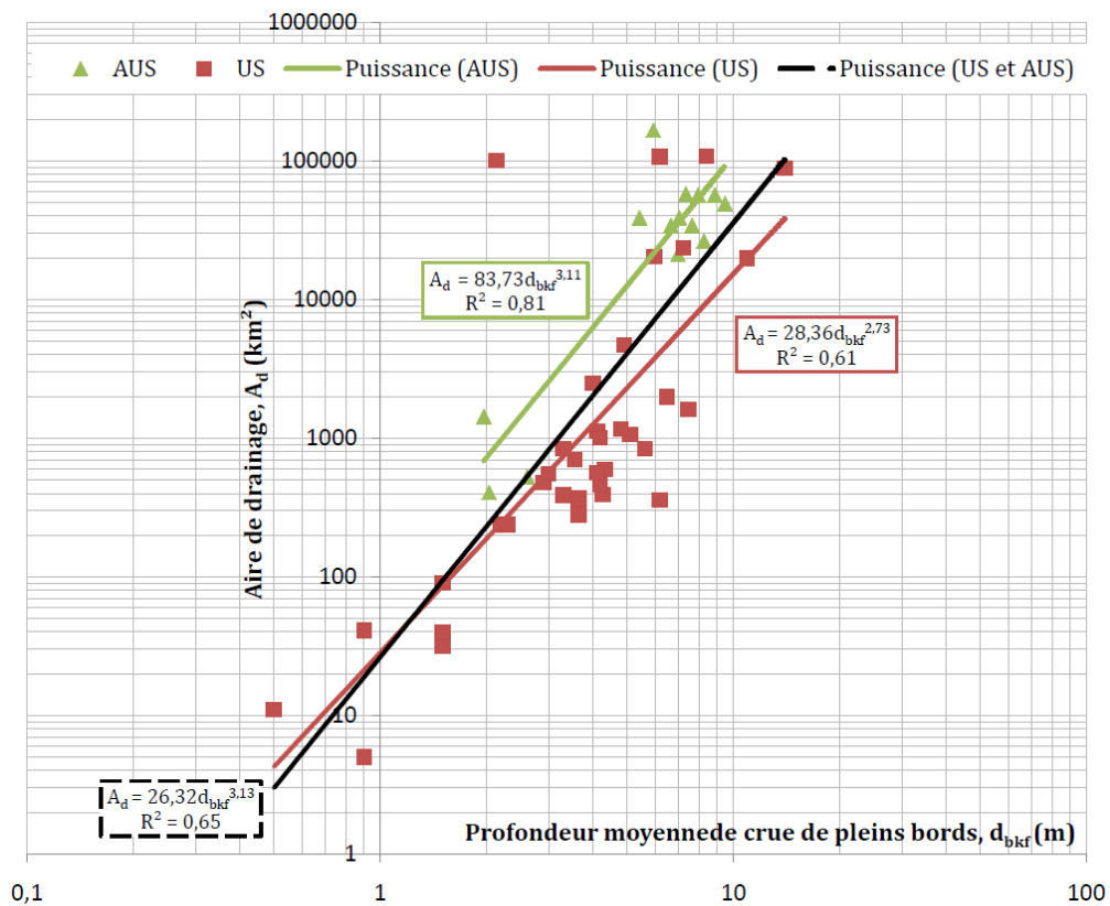
Figure 5-23 : Aire de drainage ( A_d ) exprimée en fonction de la profondeur moyenne de crue de pleins bords ( d_{bkf} ) pour des données de rivières issues du domaine climatique subtropical semi-aride.
