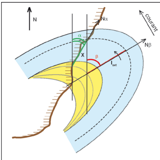
Figure 4-30 : Représentation en plan des géométries mesurées. L'affleurement est représenté en marron. En vert, le segment X correspond à l'extension horizontale du set mesurée au télémètre ou au GPS. En rouge, le segment l_{set} correspond à la largeur du set que nous cherchons à estimer (à l'apex du méandre). L'angle vert \alpha correspond à la direction de la visée ou du pointé GPS et l'angle rouge \beta correspond à la direction de migration du set. La flèche noire indique la direction du courant au point où la mesure est effectuée
