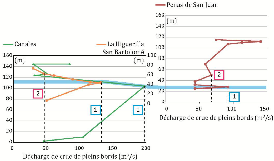
Figure 6-25 : Variations des décharges de crues de pleins bords des chenaux mesurés dans la série du Fan de Tórtola (Paléobordure ouest : Canales La Higuera et San Bartolomé. Paléobordure Est : Peñas de San Juan).
