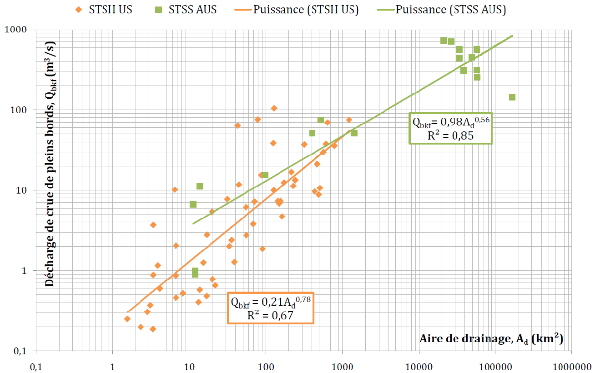
Figure 5-31 : Comparaison des lois entre Décharge de crue de pleins bords et Aire de bassin versant des domaines subtropicaux semi-humides (STSH) et à saisons sèches (STSS).
