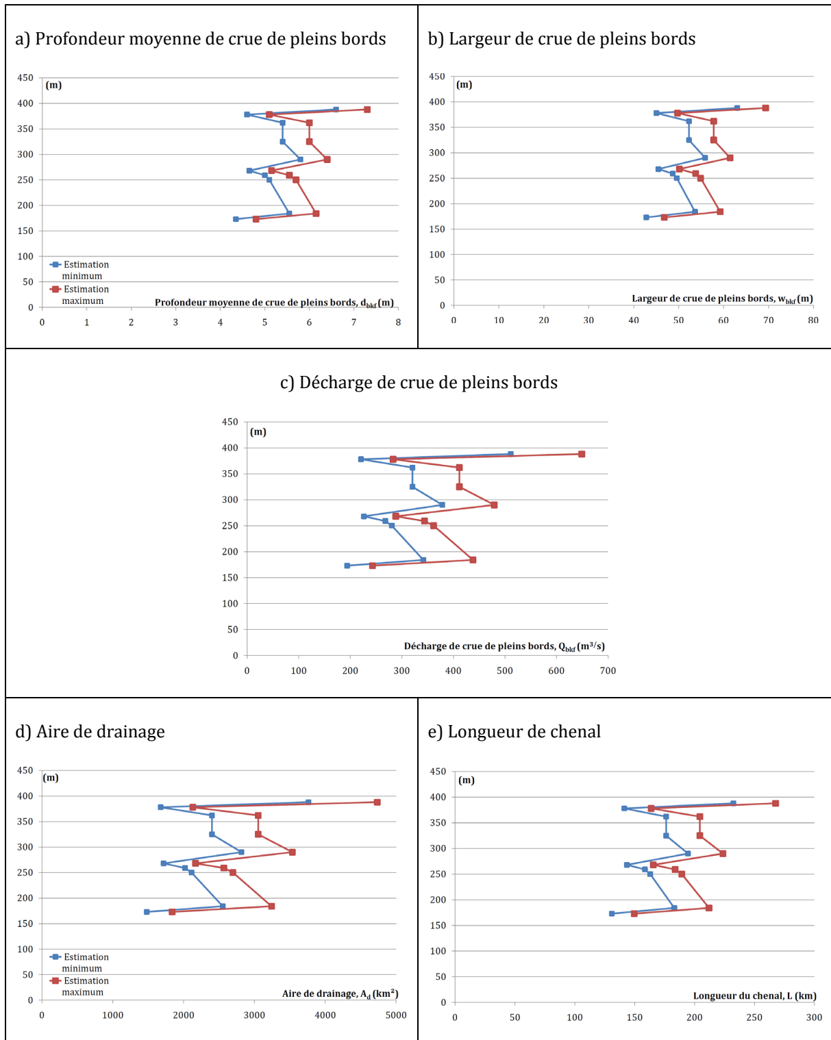
Figure 6-3 : Évolution stratigraphique des paramètres paléohydrologiques calculés pour les chenaux de la Molasse Rouge d'Esclagon (données chiffrées fournies en Annexe VI b).
