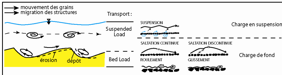
Figure 1-11 : Représentation schématique des phénomènes d'érosion et de dépôt associés à la formation des dunes. Illustration des différents modes de transport de la charge de fond et de la charge en suspension (modifié d'après Knighton, 1998).
