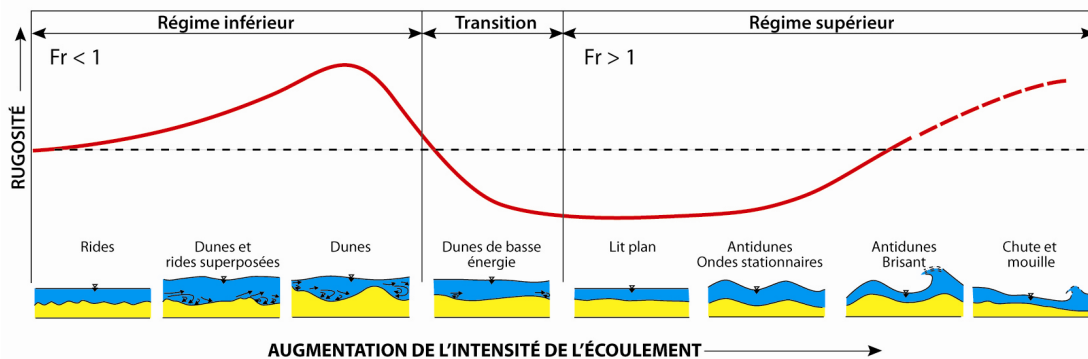
Figure 1-13 : Schéma illustrant l'impact de la rugosité sur la formation des structures sédimentaires au sein d'un système fluvial sableux. La ligne rouge représente les variations de résistance de l'écoulement associées à une augmentation de son intensité. Sont également dessinées les structures sédimentaires issues de ces différents régimes d'écoulement (d'après Knighton, 1998).
