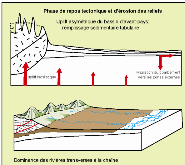
Figure 2-12 : Phase de relâche tectonique. L'érosion du prisme entraîne un rebond isostatique. La perte d'espace d'accommodation qui en résulte couplée aux importants apports sédimentaires liés à l'érosion des reliefs favorisent le développement de systèmes transverses progradants (d'après Burbank, 1992)
