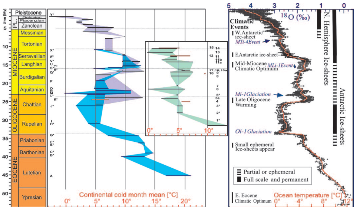
Figure 3-7 : Températures continentales des mois les plus froids d'Europe Centrale depuis 45 Ma (estimées à partir des données de flores germaniques). Ces données sont comparées aux températures océaniques moyennes estimées par Zachos et al. (2001) à partir des données isotopiques de l'oxygène (extrait de Mosbrugger et al. , 2005).
