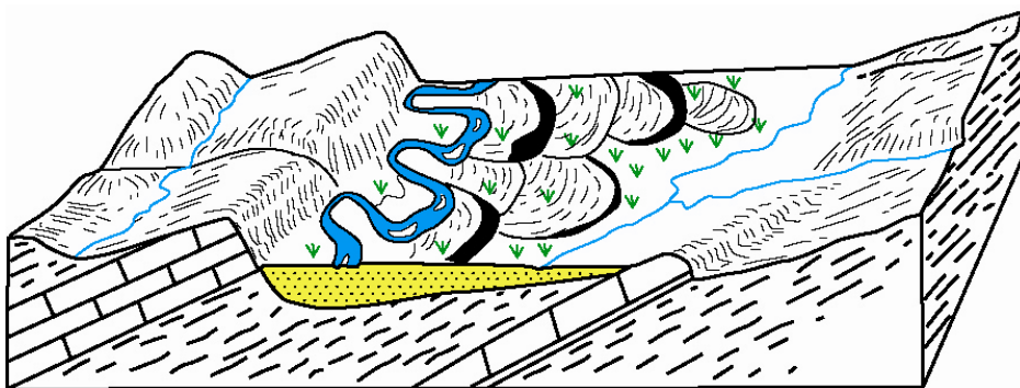
Figure 2-13 : Système méandrique développé dans une zone de basculement montrant l'asymétrie de la position de la rivière au sein de sa plaine, et l'asymétrie des dépôts de méandre plus importants sur la partie surélevée. On note également l'augmentation de la proportion de sable au niveau de l'axe du bassin et la conservation préférentielle des sols sur la partie surélevée (Holbrook et Schumm, 1999).
