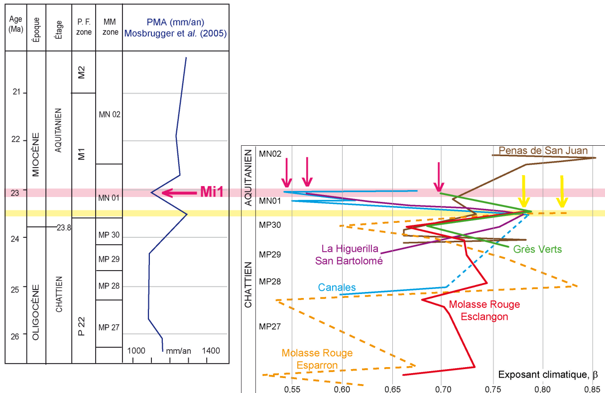
Figure 6-20 : Corrélations climatiques entre Europe septentrionale et Europe méridionale et occidentale. Les données présentées dans le graphique de gauche correspondent aux données climatiques issues de macroflore nord-germaniques (Mosbrugger et al., 2005).
