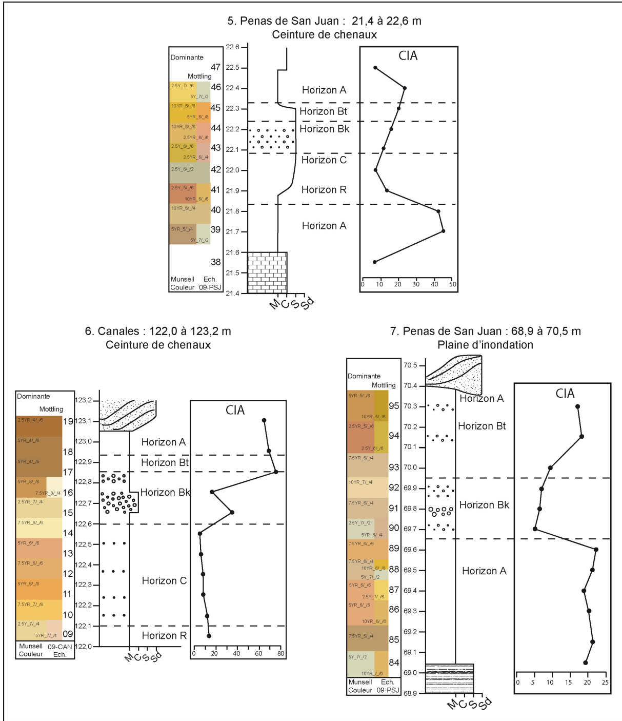
Figure 6-17 : Profil et indice d'altération calculés à partir des analyses isotopiques des paléosols de la série du Fan de Tórtola. Les sols sont numérotés de 5 à 7 par ordre stratigraphique. Les couleurs des colonnes de gauche font référence à la charte de Munsell (1909).
