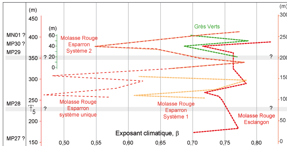
Figure 6-14 : Corrélation des signaux paléoclimatiques des Grès Verts et de la Molasse Rouge. La base des séries est estimée MP28, Chattien supérieur ( \approx 25\text{Ma} ).
