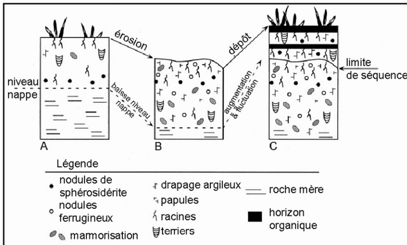
Figure 2-17: Impact des variations du niveau de base sur l'évolution d'un paléosol d'interfluve. A) Sidérite et sol gris, peu drainé. B) chute du niveau de base (nappe phréatique), la plaine est érodée des drapages argileux et des nodules ferrugineux se forment grâce à un meilleur drainage. C) remontée du niveau de base, nouveau dépôt de plaine et développement de sols hydromorphes (Kraus, 1999)
