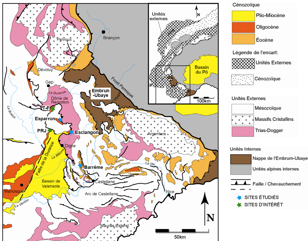
Figure 3-2 : Carte géologique synthétique du Sud-est de la France (d'après Ford et al., 1999). Les trois systèmes étudiés sont indiqués par des étoiles bleues. Les étoiles vertes indiquent les sites d'intérêt du Pont de la Reine Jeanne (PRJ) et Turriers – Faucon du Caire (T-F).
