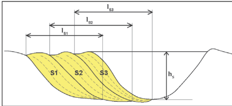
Figure 5-2 : Section en coupe d'une barre d'accrétion latérale à l'apex d'un méandre illustrant les géométries des objets sableux. S1 à S3 sets successifs déposés par accrétion latérale. La lettre l correspond à la largeur des sets et h_s à la hauteur (d'après Allen, 1965 ; Moody-Stuart, 1966).
