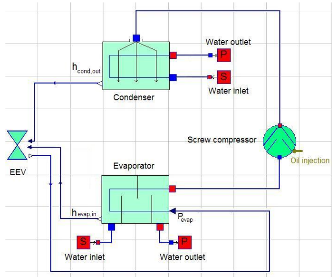
Figure 4.8 : Modèle global de la PAC assemblée dans l'environnement graphique (GUI) de Dymola™
