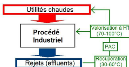
Figure 1.14 : Schéma du principe de valorisation de la chaleur fatale par PAC
