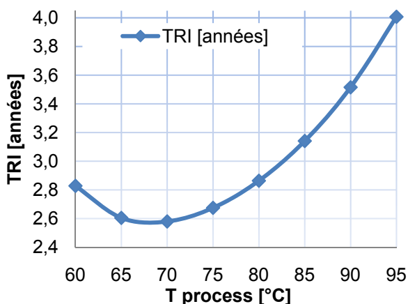
Figure 1.39 : TRI en fonction de T process
