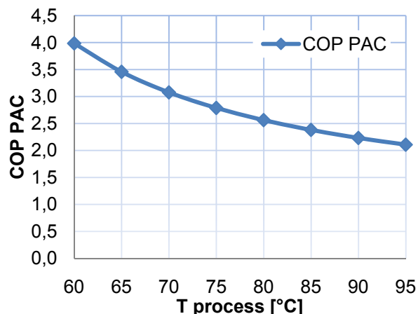
Figure 1.36 : Variation du COP de la PAC en fonction du niveau T_{process} fourni
