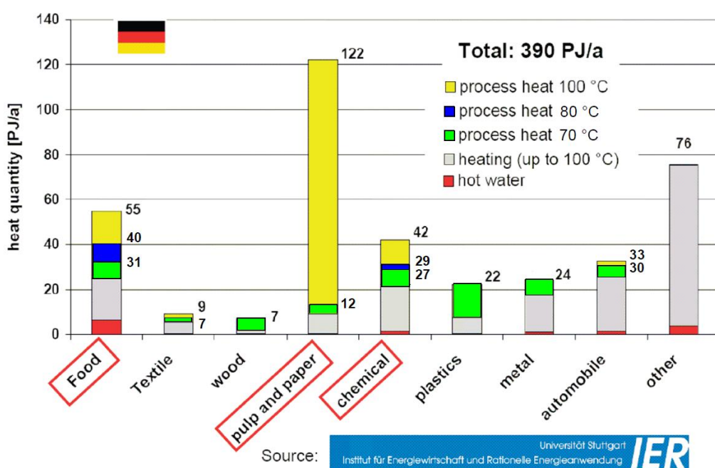
Figure 1.12: Distribution du besoin de chaleur par secteur industriel en Allemagne pour trois niveaux de température process (70 °C, 80 °C et 100 °C)
