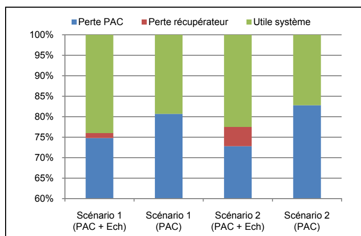
Figure 2.23 : Répartition des utilisations exergetiques en % du système (PAC et échangeur récupérateur) dans chaque configuration selon le scénario ( \eta_{ex} compresseur corrigé et T_0 = 300\text{ K} )
