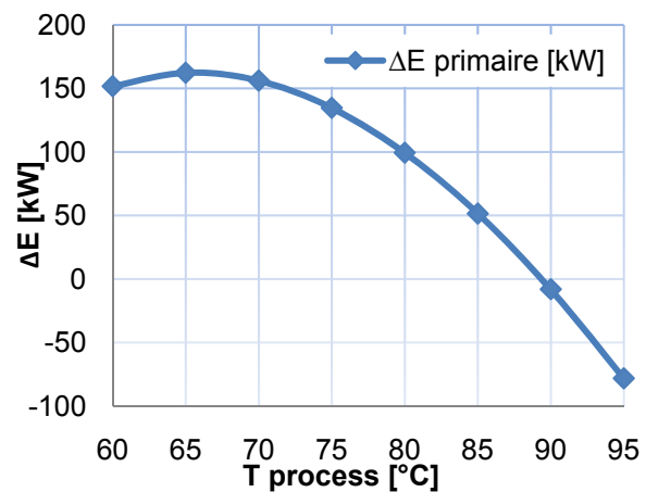
Figure 1.37 : Gain en énergie primaire en fonction de T_{process}
