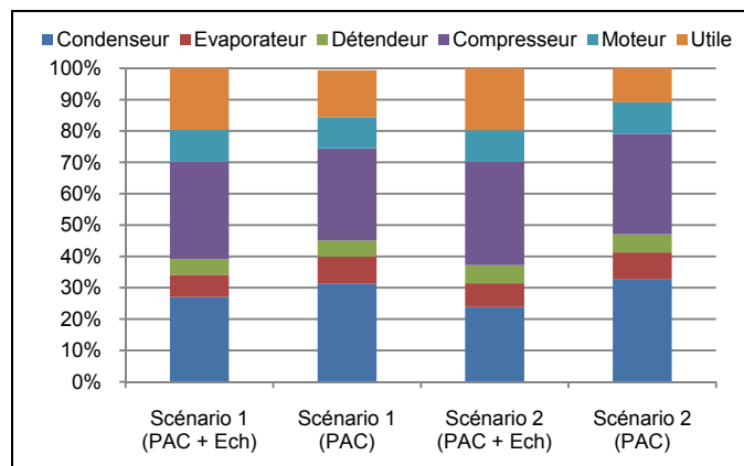
Figure 2.22 : Répartition des utilisations exergetiques de la PAC dans les différentes configurations en % ( T_0 = 300\text{ K} )
