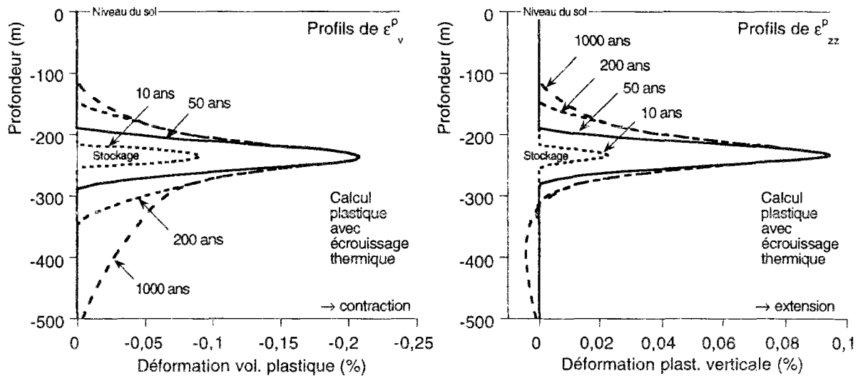
Figure 11 : Profils de déformation plastique pour le calcul plastique avec écrouissage thermique (drainage en surface).
