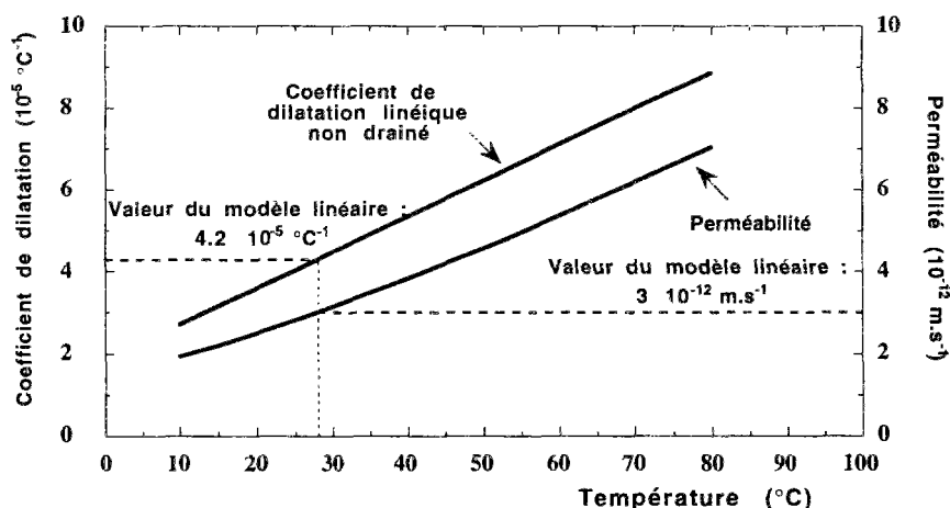
Figure A9.1 : Variations en température des caractéristiques de l'argile dans l'étude non linéaire.
