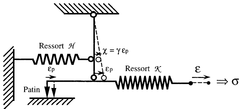
Figure 13 : Système rhéologique plastique écrouissable avec une liaison linéaire entre les allongements du patin et du ressort d'écrouissage.
