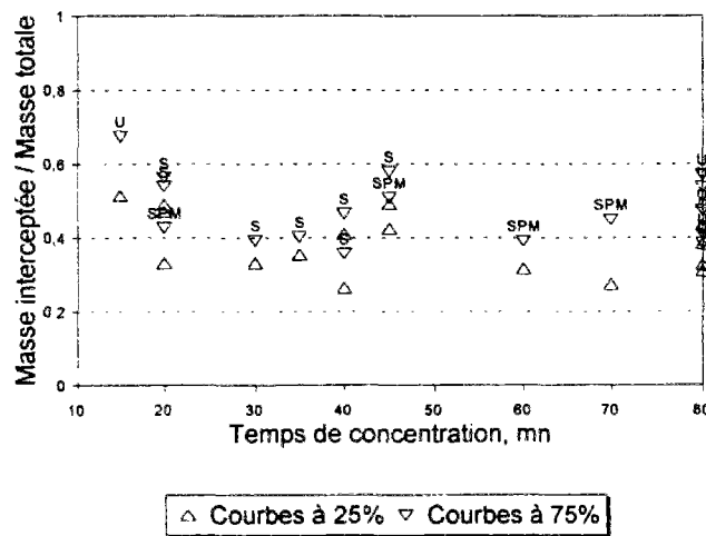
Figure 6.24 Masse de DCO interceptée à long terme par 20m 3 /ha act en fonction du temps de concentration
