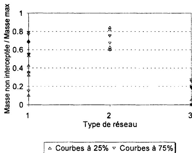
Figure 6.36 Masse de MES la plus grande non interceptée pendant un événement par 200 \text{ m}^3/\text{ha act} , en fonction du type de réseau
