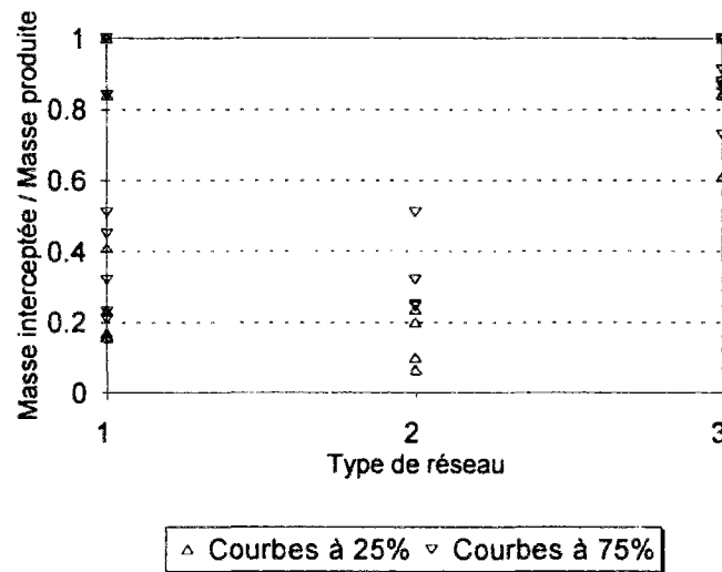
Figure 6.31 Masse de MES interceptée par 100 m 3 /ha act, pour l'événement dont la masse produite est la plus grande, en fonction du type de réseau
