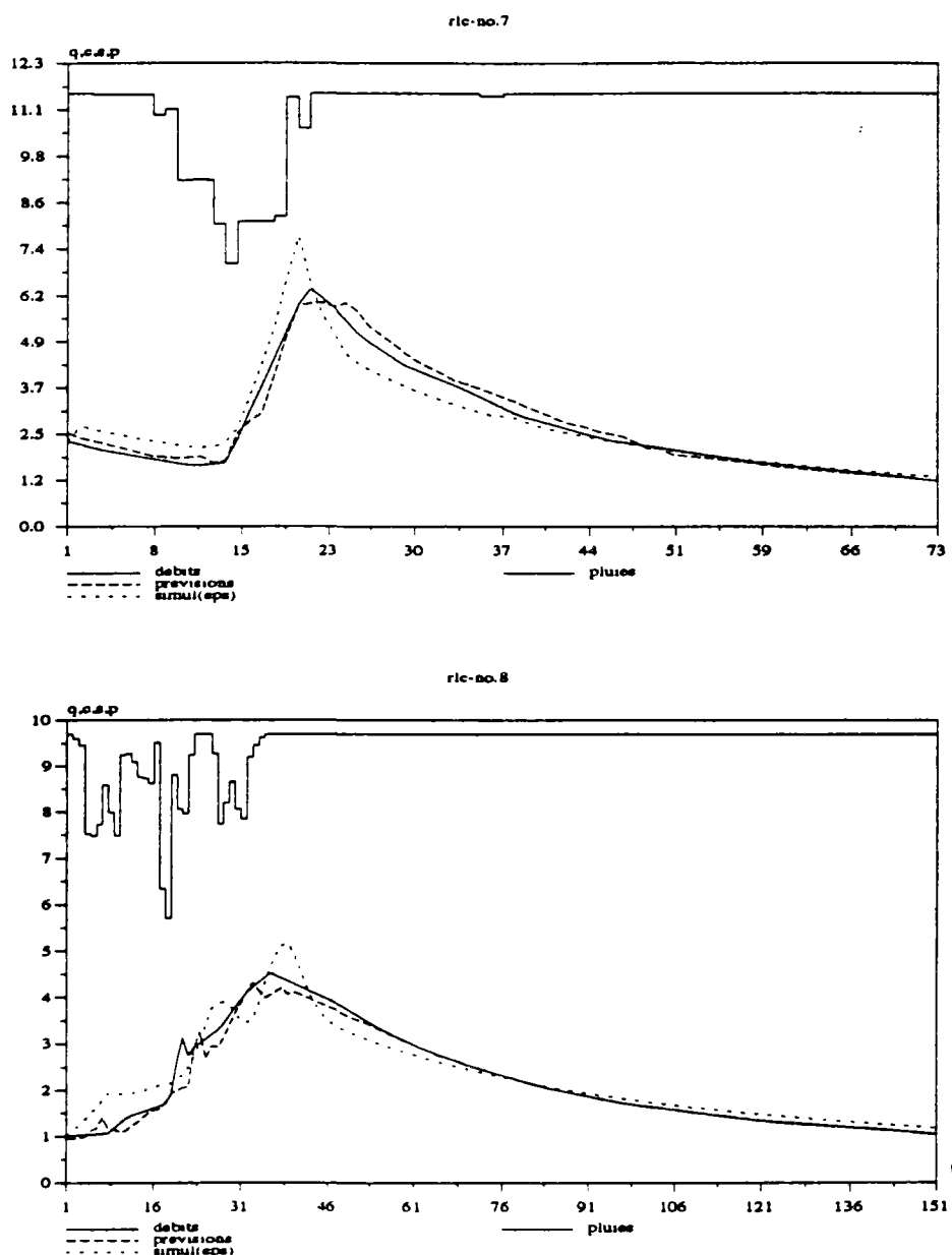
Figure 7-9 Prédiction sous condition de pluie connue (le Réal Collobrier) ——— débits mesurés ou pluies mesurées - - - - - débits prévus ..... débits simulés par épisode
