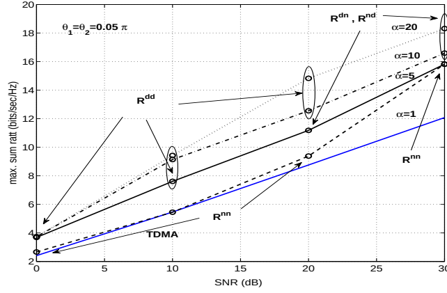
Figure 5: Somme moyenne des débits pour différentes structures de décodage comparées à TDMA dans un canal symétrique en fonction du SNR.
