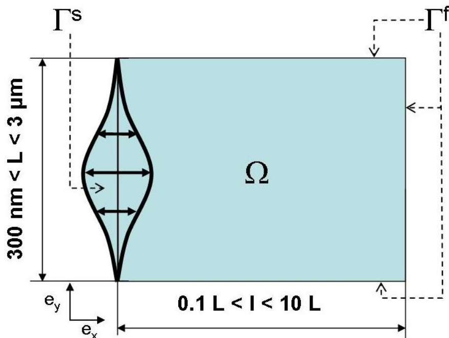
FIGURE III.3.1 – Géométrie rectangulaire
