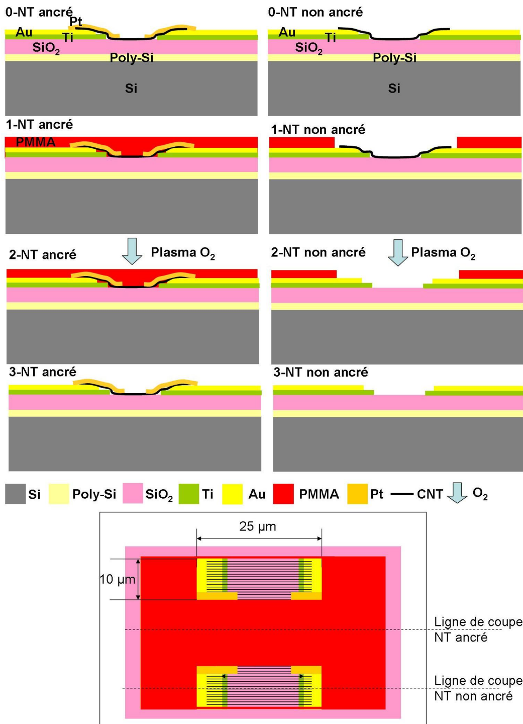
FIGURE IV.2.21 – Etapes de gravure des nanotubes hors de la zone d’ancrage. 0) Etat initial : nanotubes ancrés et non ancrés. 1) Mise en forme de la résine selon le motif dessiné dans l’encart en bas de la figure : les nanotubes hors de la zone d’ancrage ne sont pas masqués par la résine. 2) Gravure des nanotubes non masqués par du plasma O 2 . La résine est partiellement gravée. 3) Nettoyage de la résine résiduelle.
