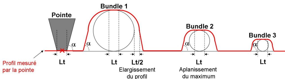
FIGURE IV.3.14 – Représentation schématique de l'effet sur les profils mesurés de la convolution du profil réel d'objets cylindriques par une pointe de largeur non négligeable devant la taille des objets : l'effet est un élargissement du profil et un aplatissement des maxima. L'effet est très prononcé pour les objets petits devant la taille de la pointe. La hauteur des maxima reste inchangée. L_t : largeur de la pointe. \alpha : angle d'attaque.
