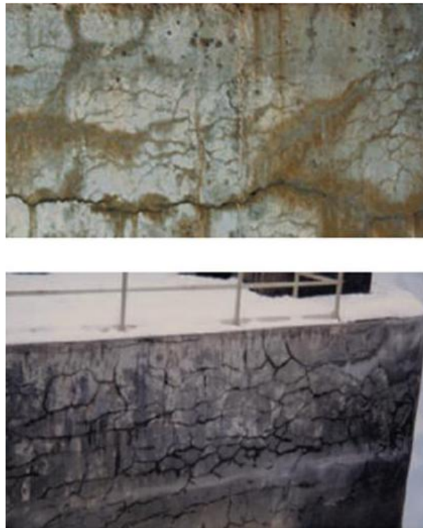
FIGURE I.3.1 – Exemples de dégradations d’ouvrages dues à l’alcali-réaction [Baroghel-Bouny 05a]
