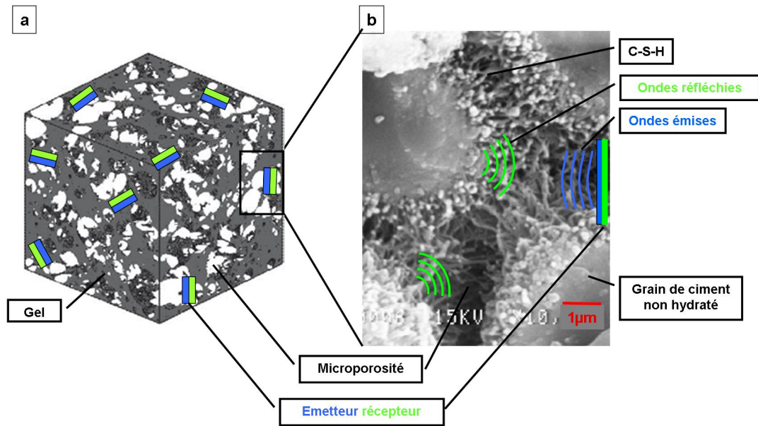
FIGURE II.2.1 – Instrumentation de la microporosité par des micro-transducteurs ultrasoniques immergés. a) Pâte de ciment avec capteurs dispersés (image : [Stroeven 10]) b) Zoom sur un micropore instrumenté par un micro-transducteur ultrasonique (image : [Damidot 05])
