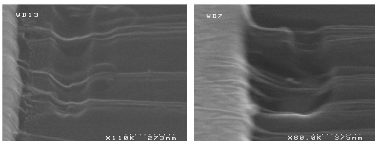
FIGURE IV.2.15 – Affaissement de nanotubes non ancrés dans une tranchée de SiO 2 créée par gravure HF.
