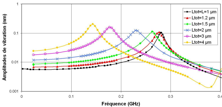
FIGURE III.5.15 – Amplitudes de vibration de la plaque en fonction de la fréquence pour des domaines de différentes largeurs L_{tot} , de profondeur l=1.3 \mu\text{m} et de largeur de plaques L=1 \mu\text{m} .
