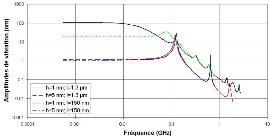
FIGURE III.5.1 – Amplitudes de vibration dans l'air de plaques de h=1 nm et h=5 nm d'épaisseur en fonction de la fréquence, pour deux domaines de largeur L=1 \mu\text{m} et de profondeurs l=0.150 \mu\text{m} et l=1.3 \mu\text{m} .
