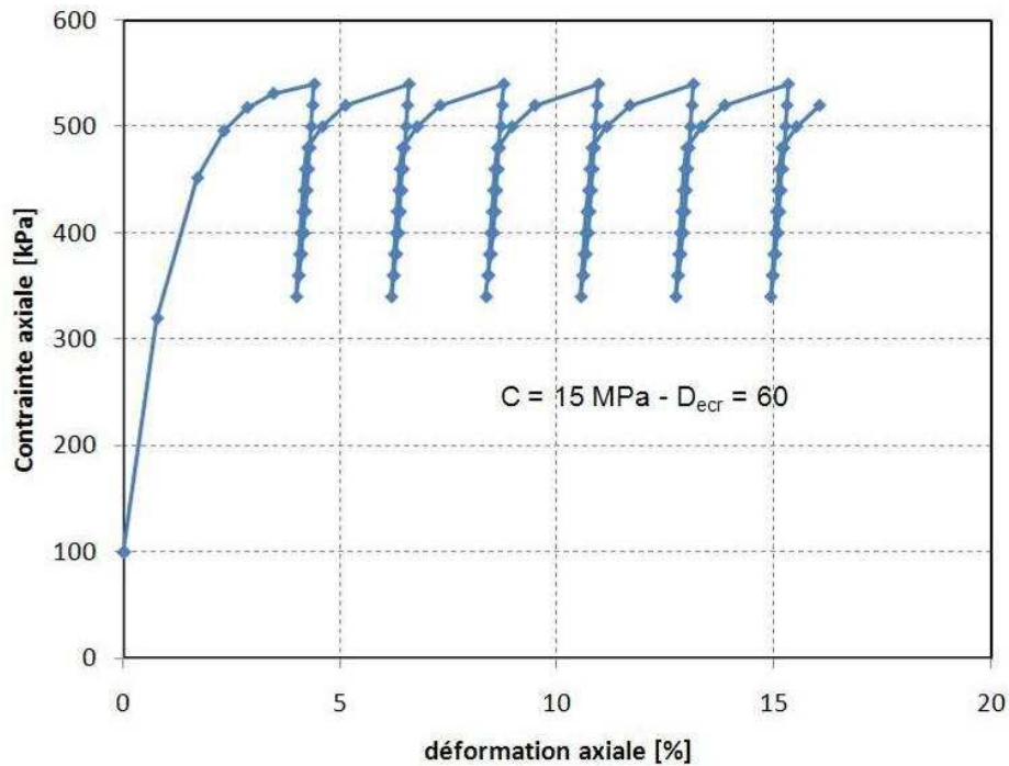
Figure 5-3 - Résultats d'une simulation d'un essai triaxial cyclique, C = 15 \text{ MPa} et D_{\text{ecr}} = 60
