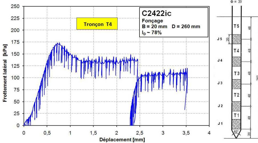
(a) frottement latéral pour le section T4
