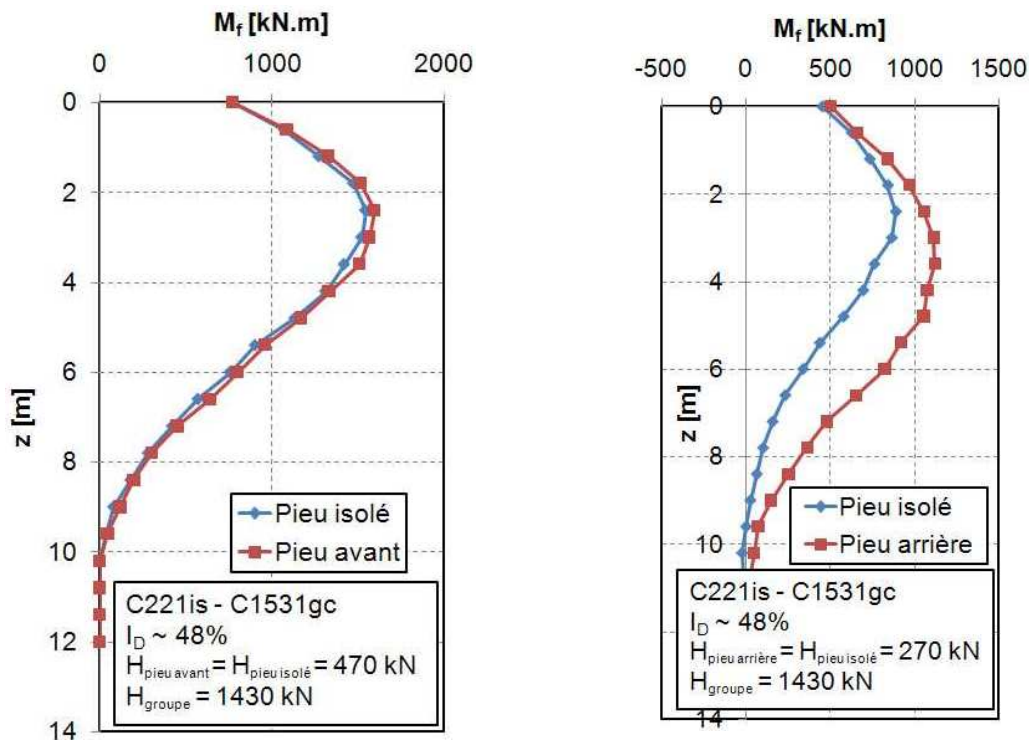
(a) – Pieu avant (dpc = 0,118B) et pieu isolé (dpc = 0,112B)
