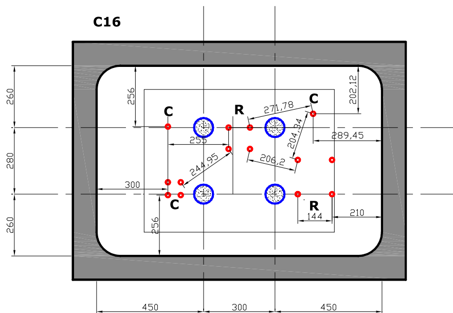
Figure 22 - Conteneur C16 ( I_D \sim 78\% ) - (M: Monotone, R: Essai à la rupture, C: Essai de chargement cyclique)
