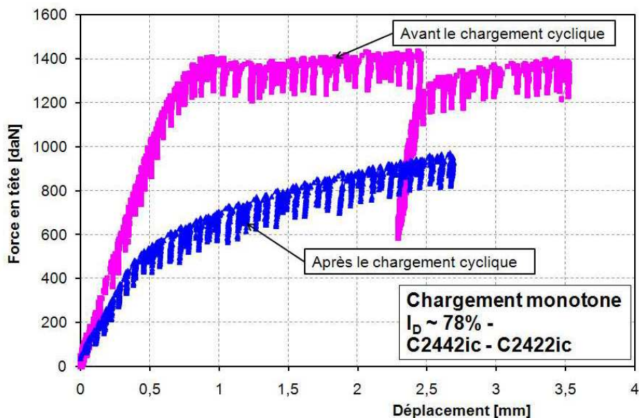
Figure 63 - Comportement du pieu avant et après le chargement cyclique
