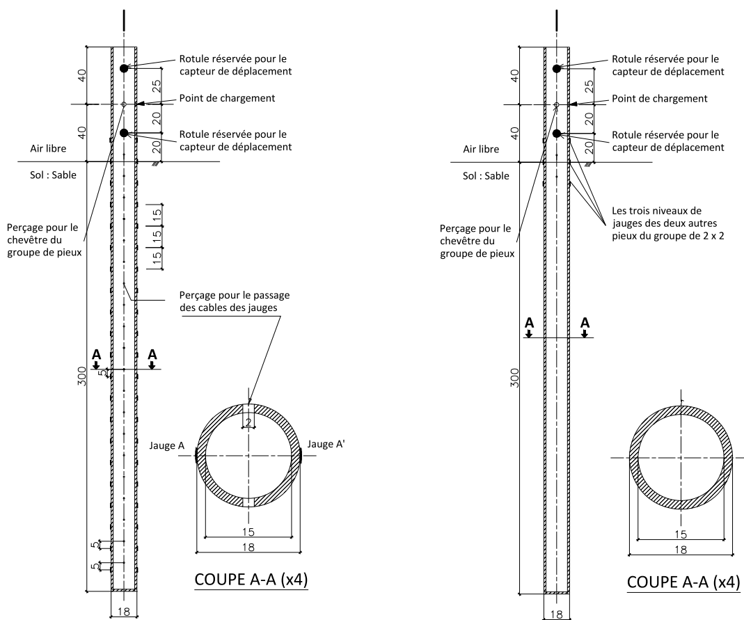
(a) Pieu instrumenté sur toute la fiche avec une jauge hors sol
