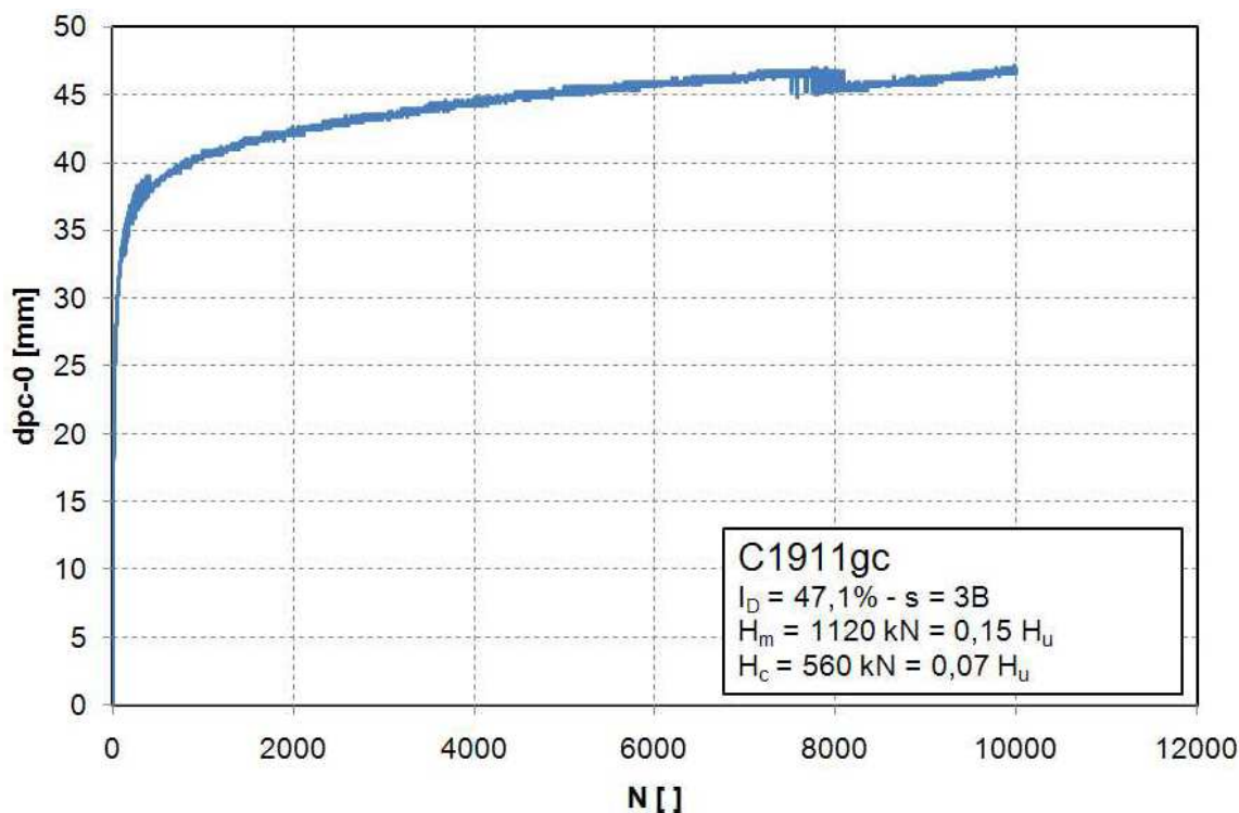
Figure 4-25 - Déplacements maximaux en tête du groupe en fonction du nombre de cycles
