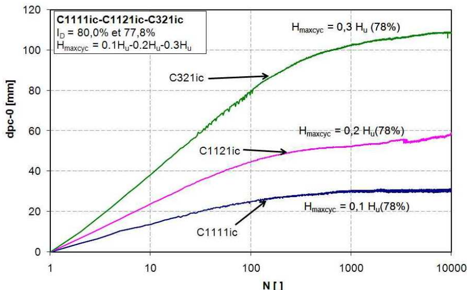
Figure 3-38 - Accumulation de déplacements cycliques en tête du pieu pour I_D \sim 78\%
