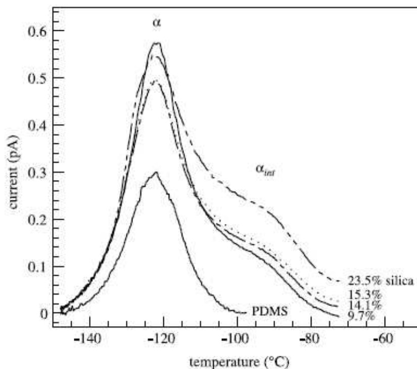
FIGURE 4.26 – Thermogrammes TSDC d'échantillons chargés SiO_2 "étain" polarisé à 20°C avec des vitesses de refroidissement et de chauffe de 10 °C/min et 3°C/min respectivement [12]
