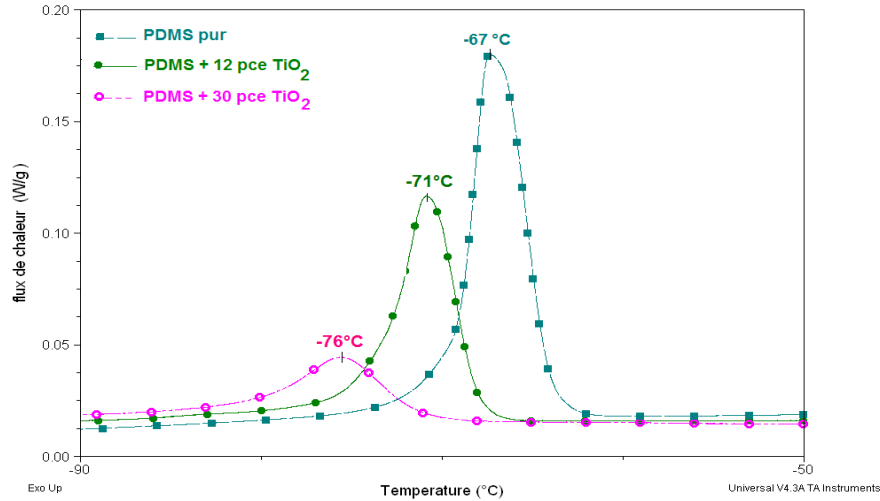
FIGURE 4.5 – Evolution du pic de cristallisation en fonction du taux de TiO_2 in situ “étain” (vitesse de refroidissement -1.5^\circ\text{C}/\text{min} )
