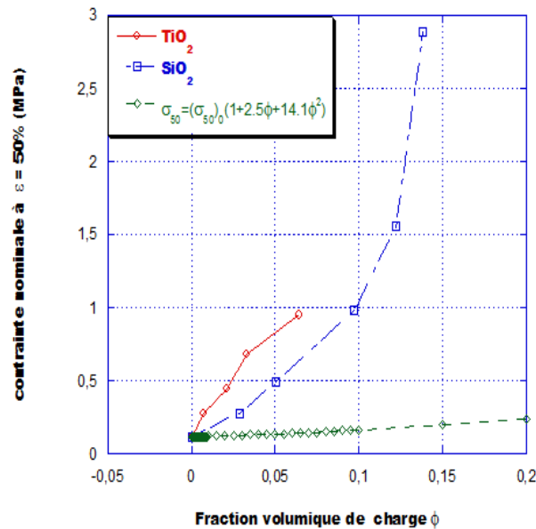
FIGURE 6.14 – Evolution des contraintes nominales atteintes à 50% de déformation pour les échantillons catalysés par un dérivé de l'étain
