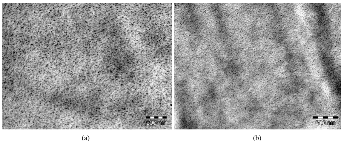
FIGURE 3.21 – Clichés MET d'un échantillon chargé de 10 pce de TiO_2 généré en présence d'ammoniaque
