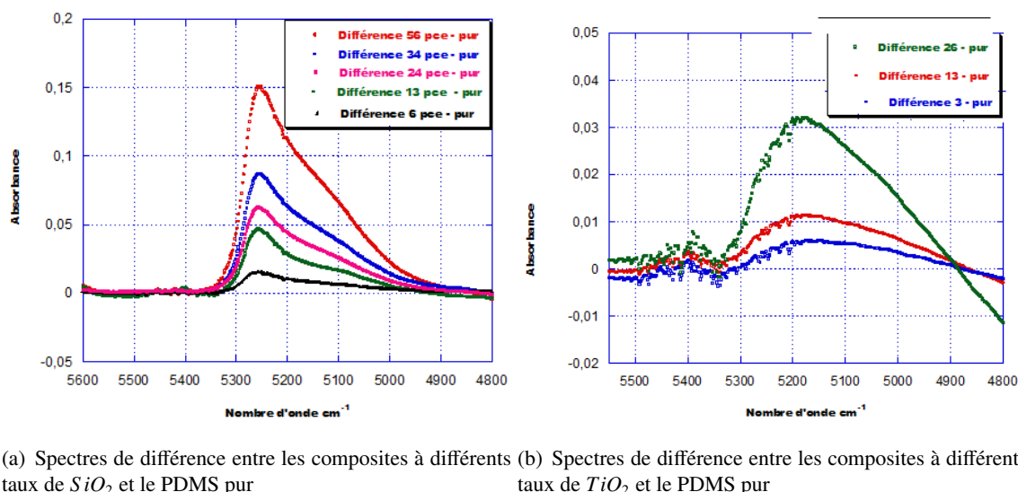
FIGURE 2.27 – Spectres de différences entre les composites à différents taux de charge et le PDMS non-chargé
