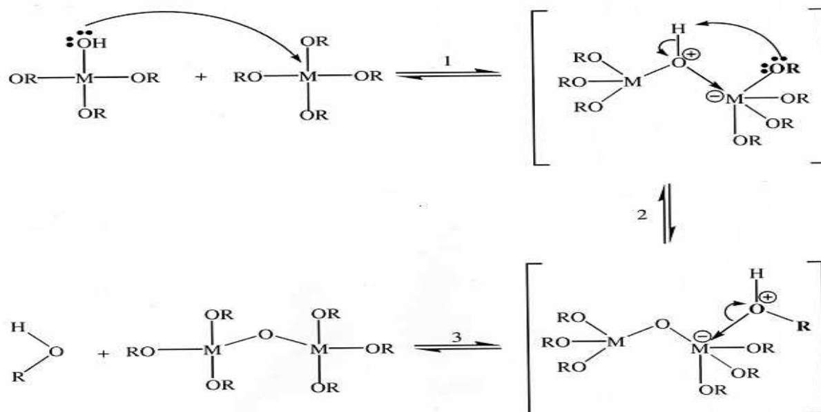
FIGURE 1.11 – Mécanisme d'alcoxolation des alcoxides M(\text{OR})_m
