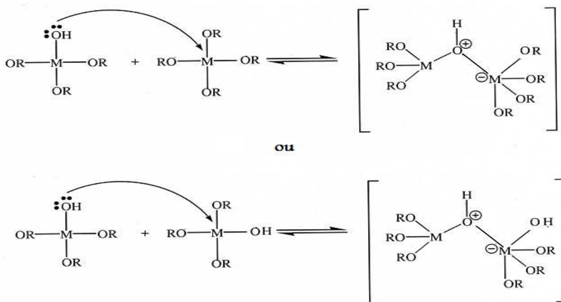
FIGURE 1.14 – Mécanisme d'olation des alcoxydes M(OR)_m
