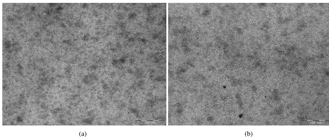
FIGURE 2.31 – MET de PDMS + 23 pce \text{TiO}_2 sur la croûte à différents endroits
