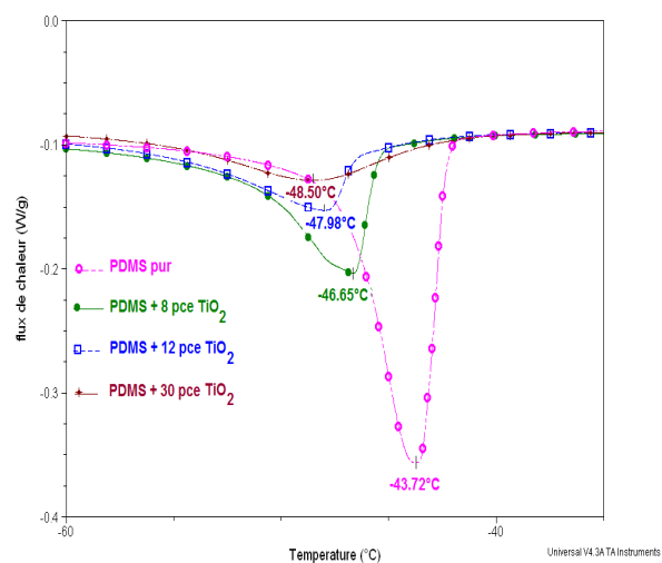
FIGURE 4.10 – Evolution du pic de fusion en fonction du taux de TiO_2 "étain" vitesse de chauffe 3^\circ C/min
