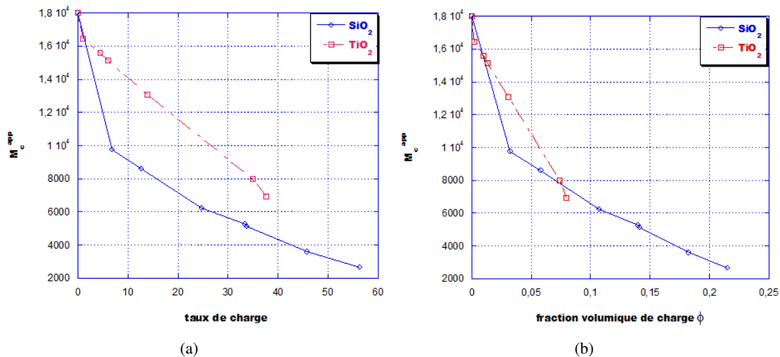
FIGURE 4.14 – Evolution de la masse molaire entre points de jonctions apparents : (a) en fonction du taux de charge (b) en fonction de la fraction volumique de charge
