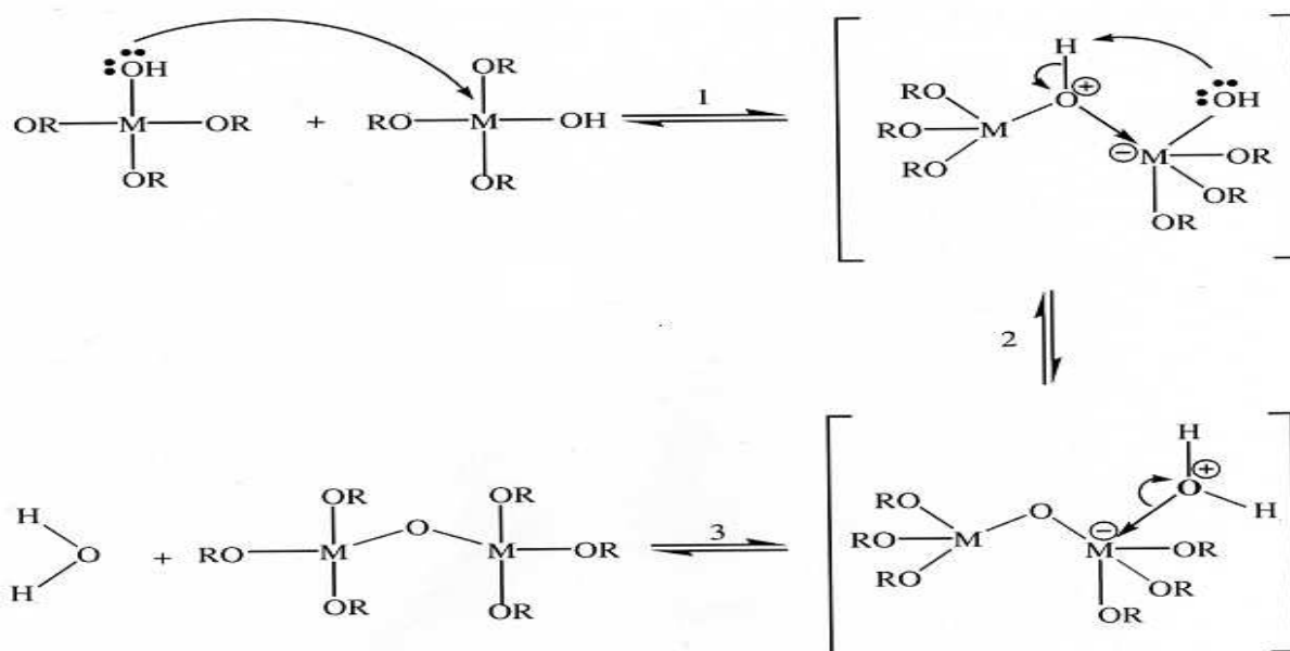
FIGURE 1.12 – Mécanisme d'oxolation des alcoxides M(\text{OR})_m
