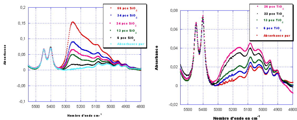
(a) Spectres proche-IR dans la gamme 4800 - 5600\text{cm}^{-1} de PDMS chargé à différents taux de \text{SiO}_2 (b) Spectres proche-IR dans la gamme 4800 - 5600\text{cm}^{-1} de PDMS chargé à différents taux de \text{TiO}_2
