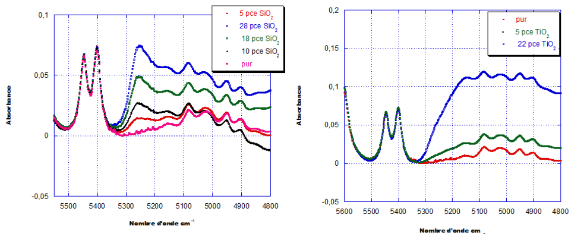
(a) Spectres proche-IR dans gamme 4800\text{--}5600\text{ cm}^{-1} de PDMS chargé à différents taux de \text{SiO}_2 (catalyseur DEA) (b) Spectres proche-IR dans gamme 4800\text{--}5600\text{ cm}^{-1} de PDMS chargé à différents taux de \text{TiO}_2 (catalyseur (ammoniaque))
