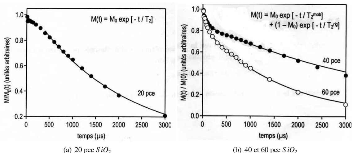
FIGURE 4.25 – Relaxation de l'aimantation pour une matrice de PDMS réticulé chargée avec 20 pce, 40 et 60 pce de silice de type "étain", à 30°C. Les courbes en trait plein correspondent aux meilleurs ajustements des points expérimentaux par une fonction exponentielle pour (a) et une somme de deux exponentielles pour (b).[2]
