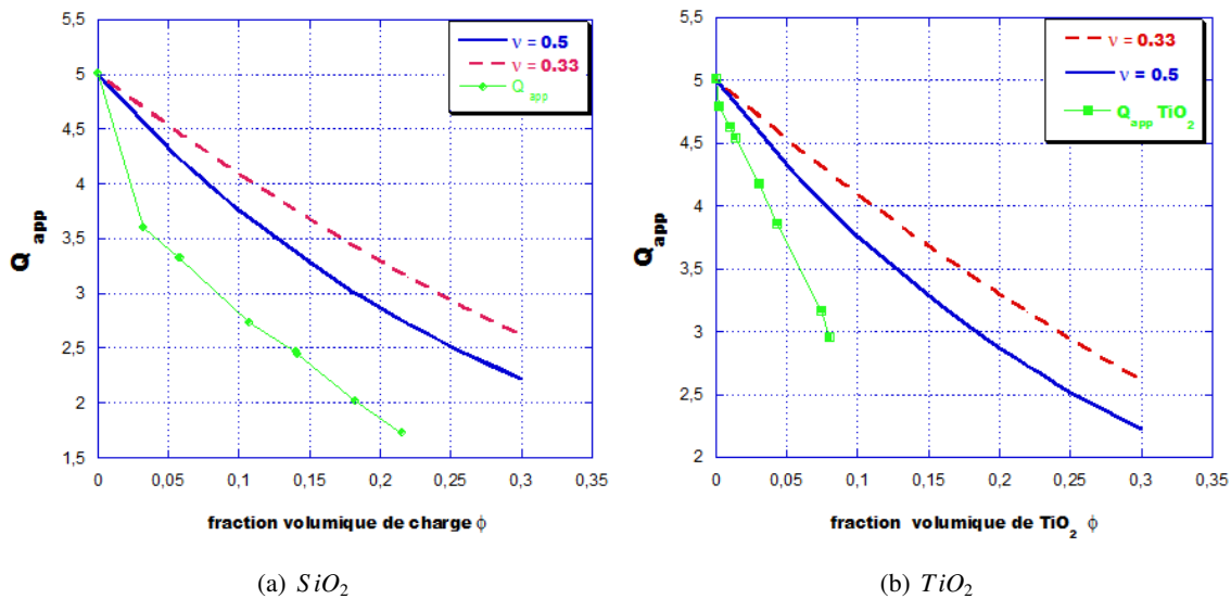
FIGURE 4.21 – Application du modèle de Lequeux au gonflement apparent des échantillons chargés
