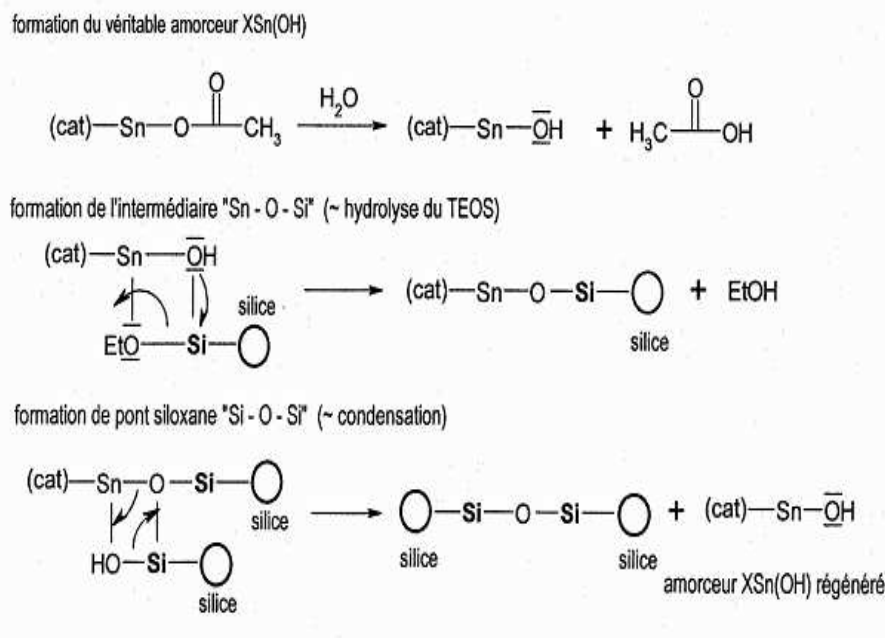
FIGURE 2.16 – Mécanisme d'intervention du diacétate de dibutyle d'étain comme catalyseur [10]
