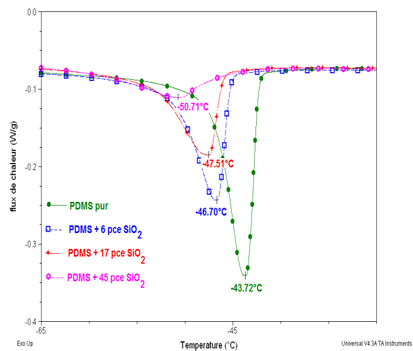
FIGURE 4.9 – Evolution du pic de fusion en fonction du taux de SiO_2 "étain" vitesse de chauffe 3^\circ C/min
