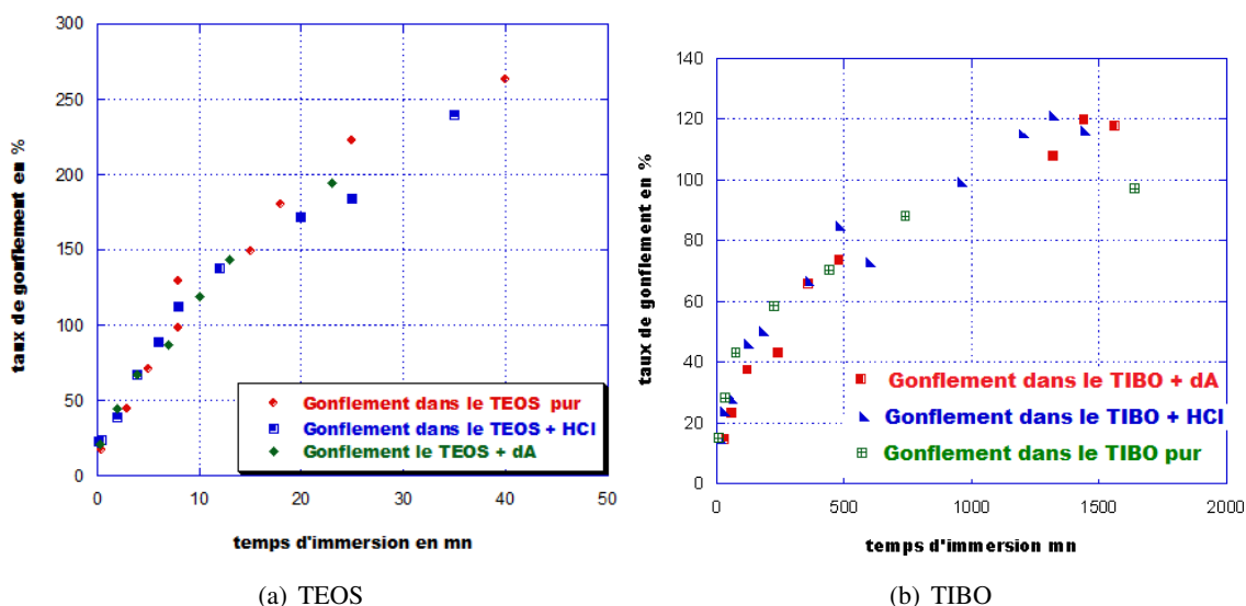
FIGURE 2.4 – Absorption des deux alcoxydes en fonction du temps
