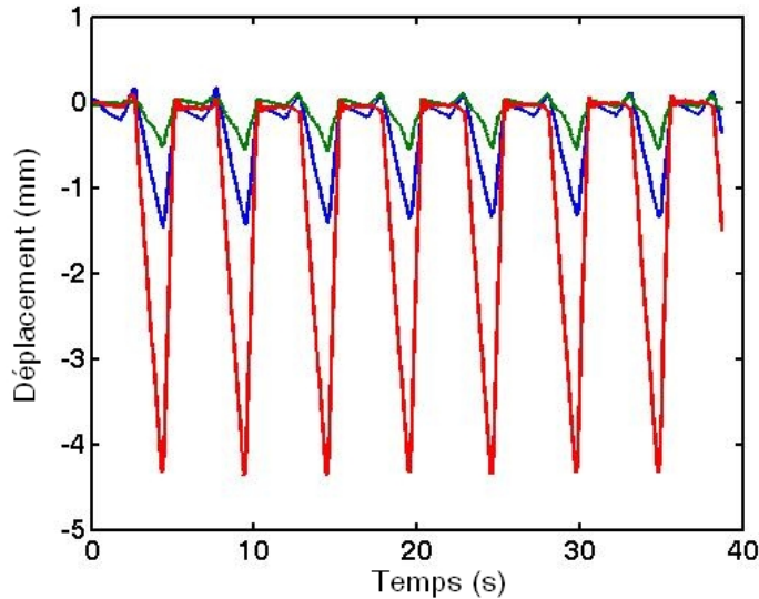
FIGURE 5.6 – Mouvement 3D estimé à travers les côtes par notre réseau de thérapie.
