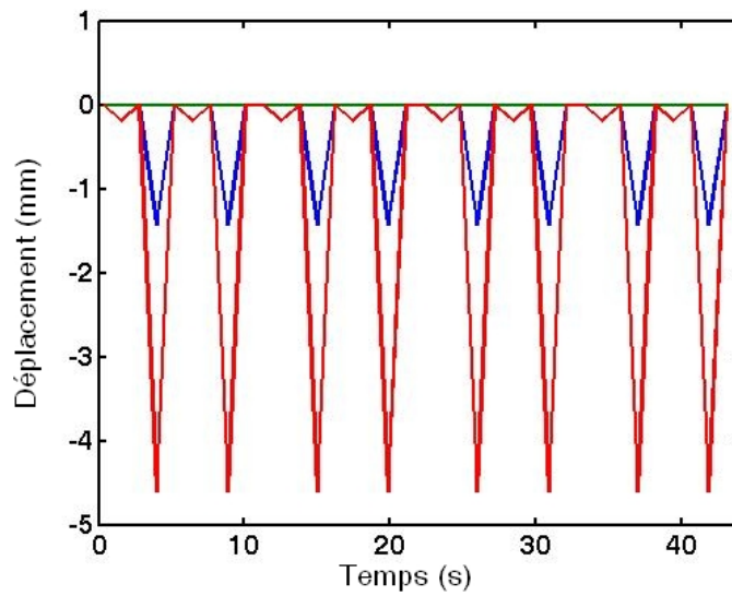
FIGURE 5.4 – Mouvement en 3D du moteur programmé. Ce mouvement est une approximation du mouvement estimé in-vivo lors des expérimentations sur des porcs anesthésiés et ventilés (cf 4.2.2).
