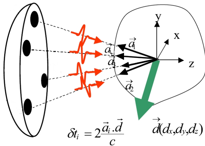
FIGURE 4.6 – Système de suivi du mouvement
