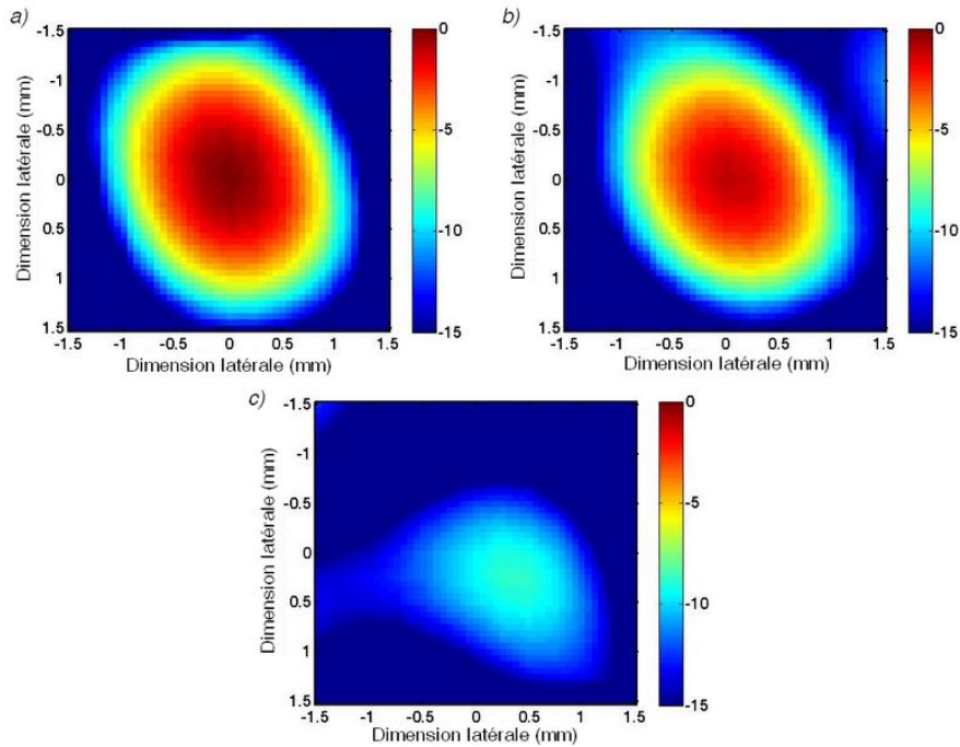
FIGURE 2.13 – C-Scans montrant le dépôt d'énergie (échelle logarithmique) dans le plan focal en utilisant le retournement temporel classique (a), le retournement temporel non-invasif (b) et une loi sphérique (c).
