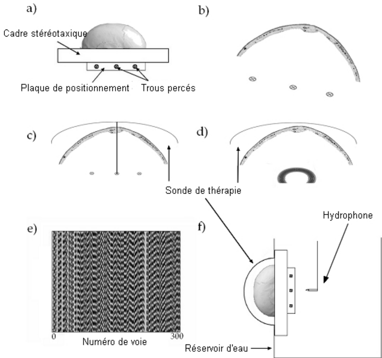
FIGURE 2.7 – Protocole non-invasif de focalisation transcrânienne
