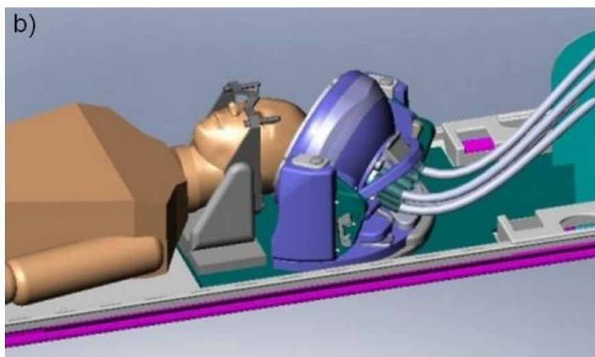
FIGURE 3.17 – a) Nouveau prototype clinique développé par SSI. Les émetteurs sont répartis selon 8 spirales. b) Positionnement du patient dans l'IRM sous contrôle stéréotaxique.
