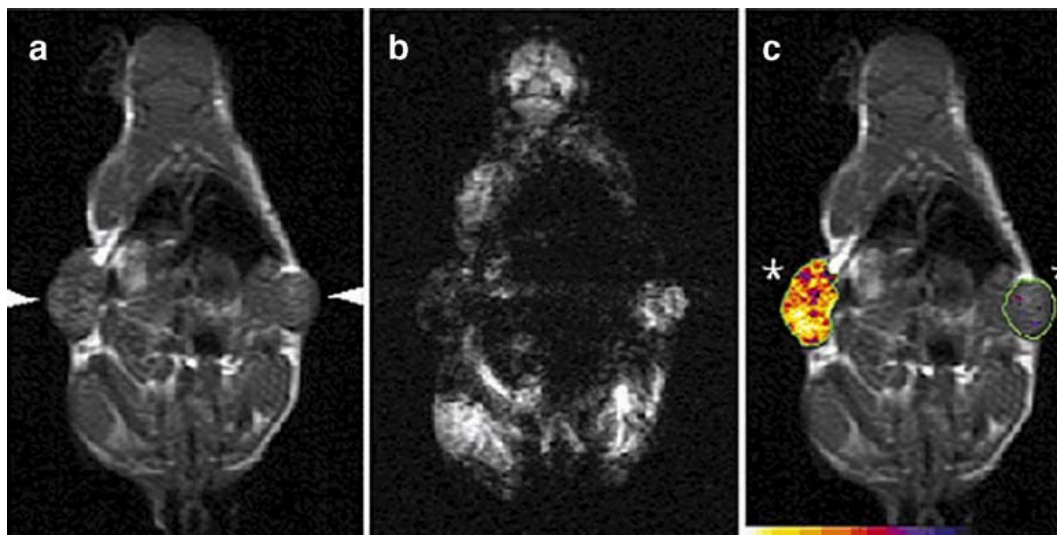
FIGURE 1.5 – a) Image contrastée en T_1 de tumeurs avec le récepteur ETR (flèche gauche) et sans le récepteur (flèche droite). b) Image écho de gradient contrastée en T_2 du même animal après l'injection de la sonde Tf-MION, l'accumulation dans les cellules de la sonde superparamagnétique diminue l'intensité du signal. c) Image composée d'une image écho de spin contrastée T_1 avec en surimposition une image représentant le changement en T_2^* entre avant et après administration de la sonde superparamagnétique [49].
