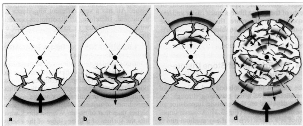
FIGURE 1.6 – Différentes phases de la désagrégation d'un calcul par lithotripsie [54]
