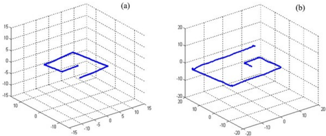
FIGURE 4.10 – Estimation du déplacement (mm), (a) V \approx 1 \text{ cm.s}^{-1} , (b) V \approx 1,7 \text{ cm.s}^{-1} .
