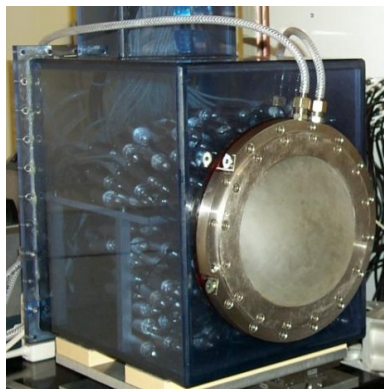
FIGURE 3.4 – Photographie du réseau de thérapie muni de sa membrane en latex.
