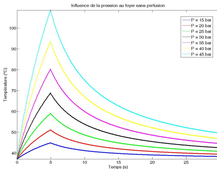
FIGURE 3.13 – Influence de la pression sur la diffusion thermique.
