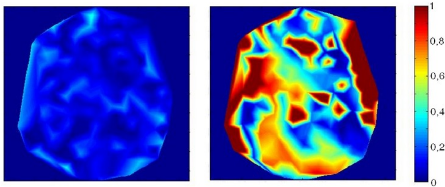
FIGURE 2.17 – Distribution spatiale de l'erreur de phase sur la surface du crâne : a) en utilisant le retournement temporel guidé par rayons X, b) sans aucune correction. L'échelle des couleurs est en nombre de longueur d'onde.
