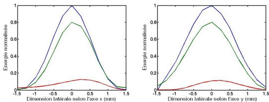
FIGURE 2.14 – Projections de la répartition d'énergie sur les deux axes du plan focal (échelle linéaire) - en bleu le retournement temporel classique, en vert le retournement temporel simulé et en rouge la loi sphérique.
