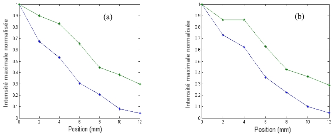
FIGURE 4.4 – Perte d'énergie avec l'angulation, bleu angulation par la dll, vert angulation par retournement temporel. (a) axe (Ox). (b) axe (Oy).
