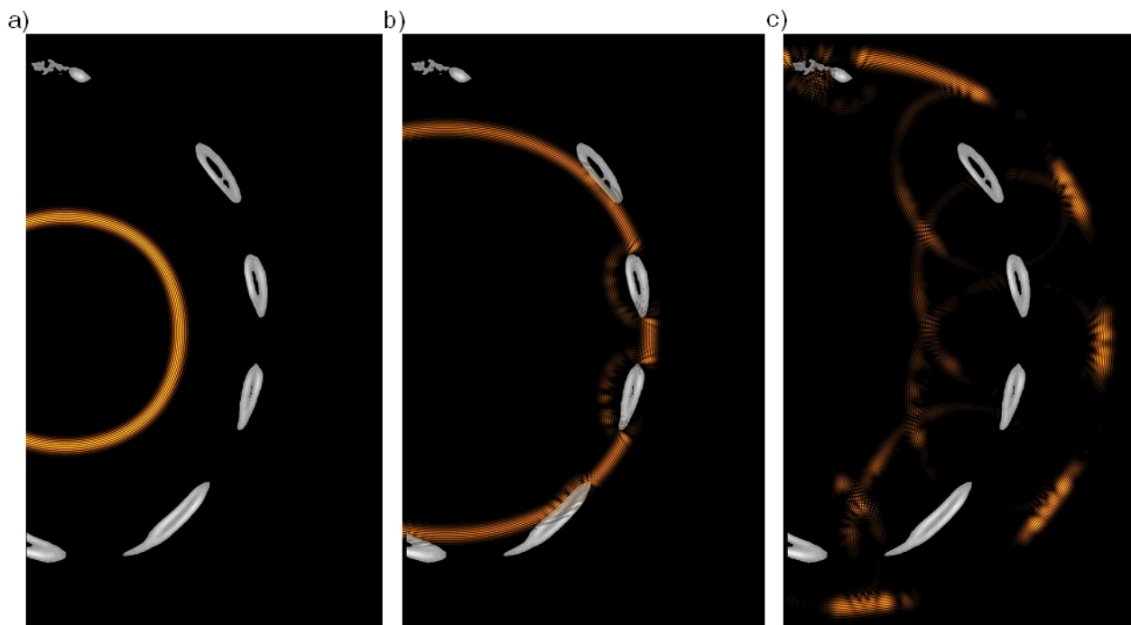
FIGURE 4.18 – Images provenant de la simulation : une source émettant une impulsion est placée au centre géométrique du réseau.
