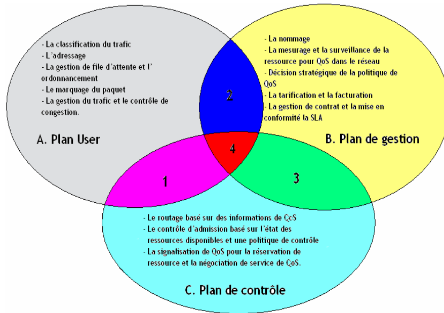
Figure 37 : La convergence des trois plans
