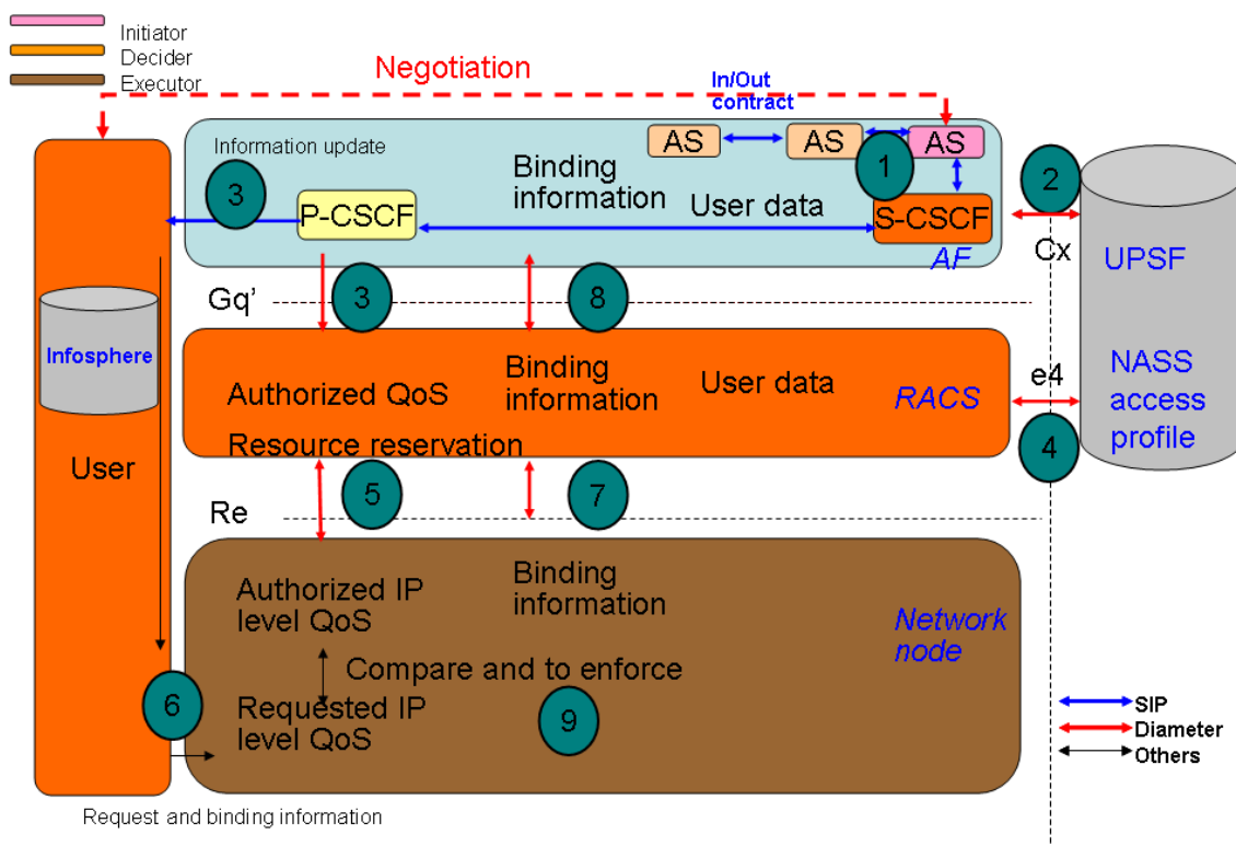
Figure 49: La négociation et binding initié par SE
