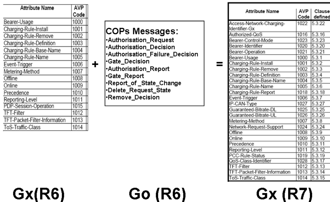
Figure 29 : Les AVPs dans l'interface Gx+
