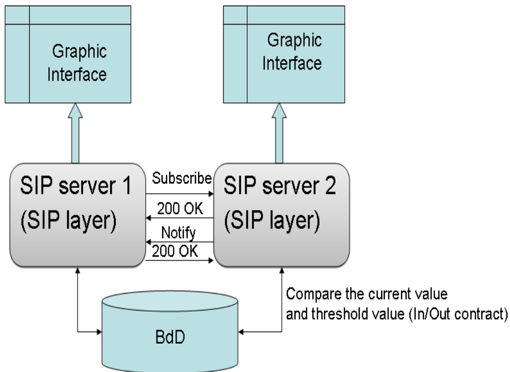
Figure 67 : Architecture global de l'implémentation
