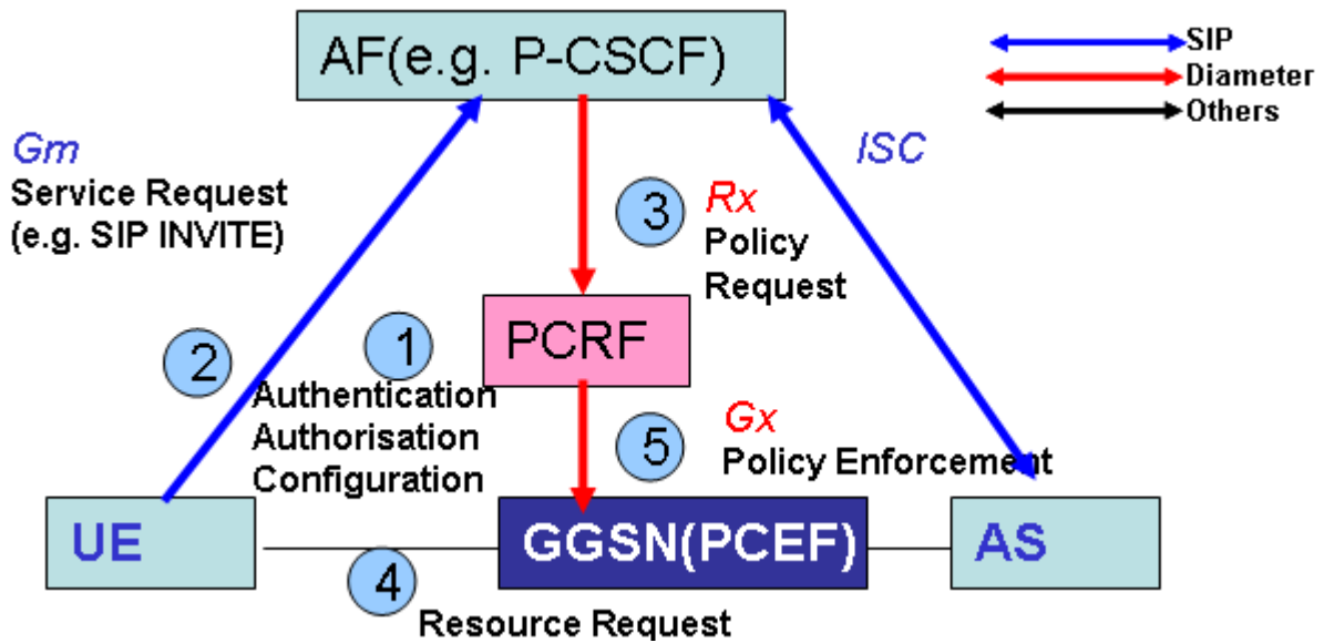
Figure 16: QoS contrôle dans le 3GPP
