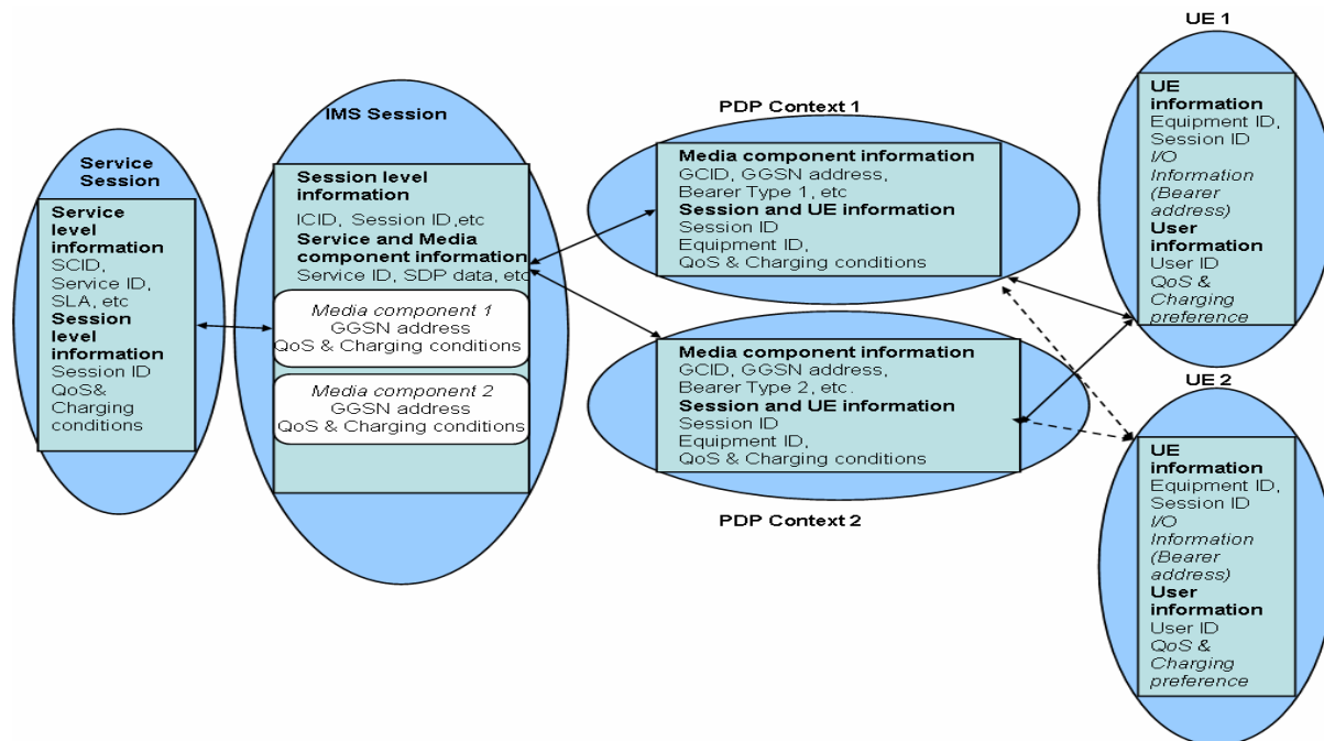
Figure 48 : La cohérence des informations par le binding E2E de la session
