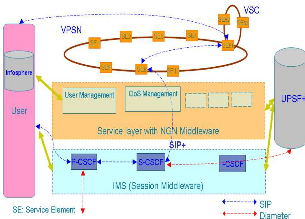
Figure 39 : Vision globale de SIP+
