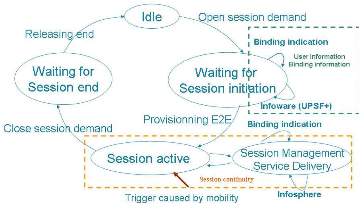
Figure 46 : Automate du binding de la session E2E
