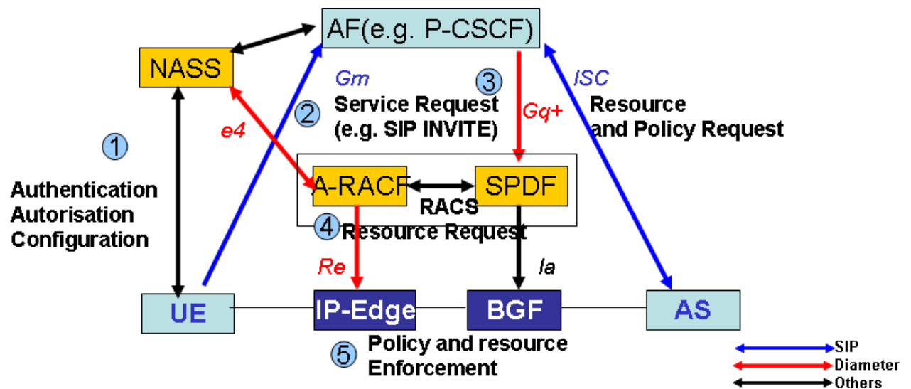
Figure 18: QoS contrôle d'ETSI TISPAN
