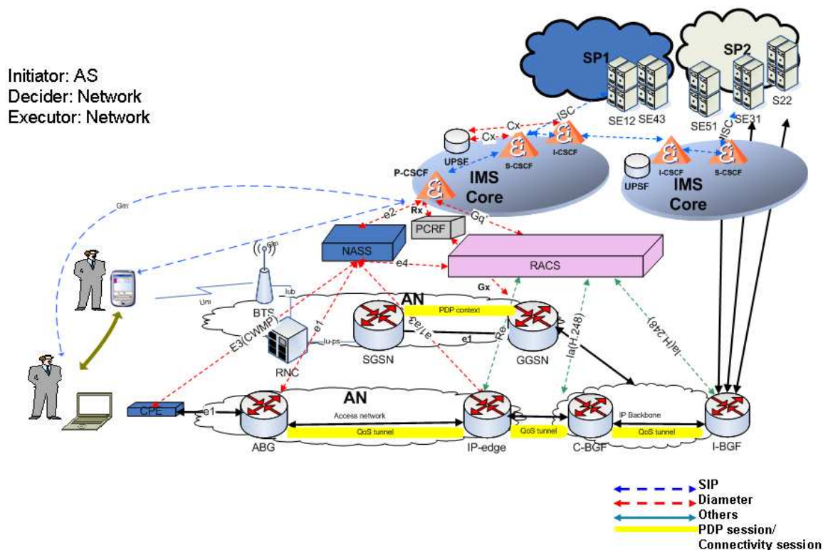
Figure 34: Scénario de la mobilité de l'utilisateur
