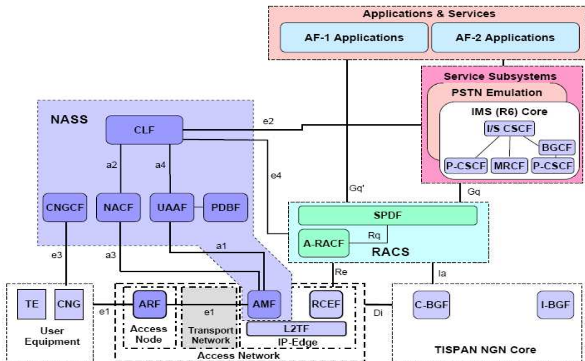
Figure 17 : L'architecture NGN de TISPAN
