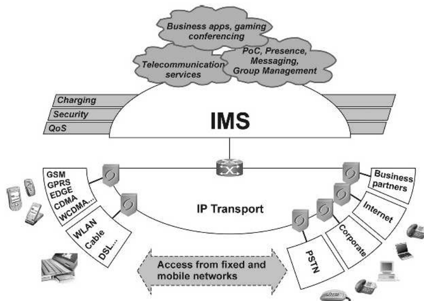
Figure 5 : L'architecture globale de l'IMS
