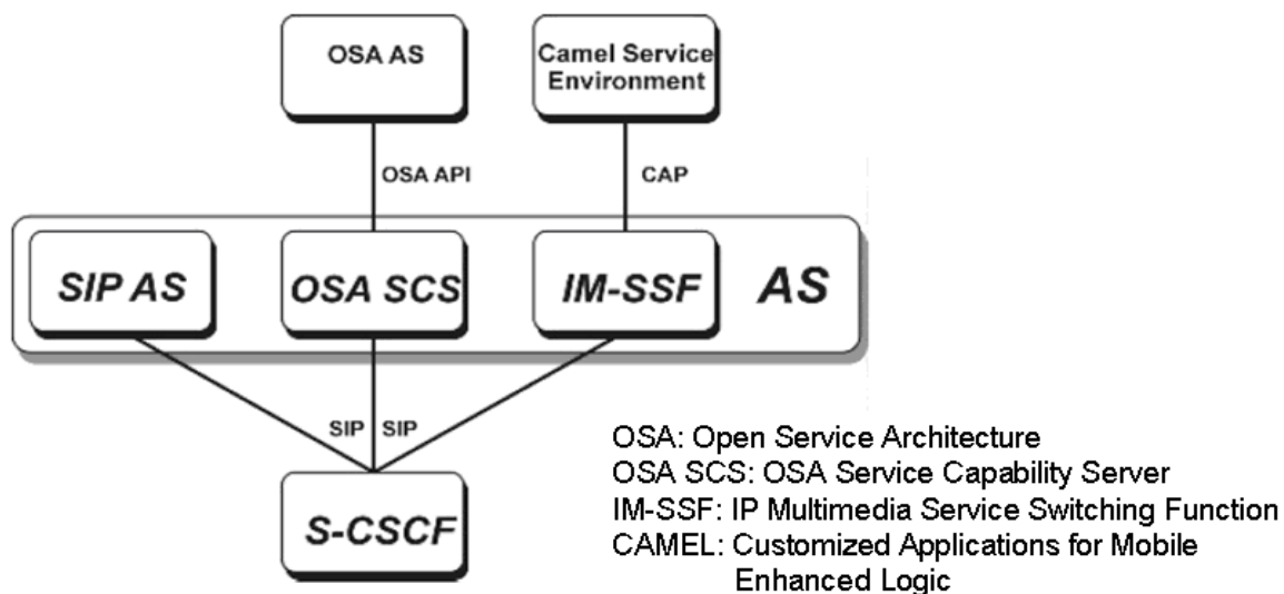
Figure 11 : Différents types d’AS
