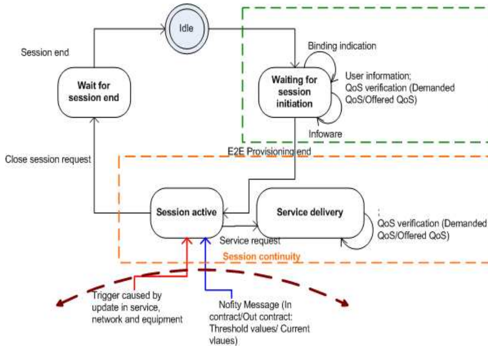
Figure 43 : Automate du contrôle de QoS
