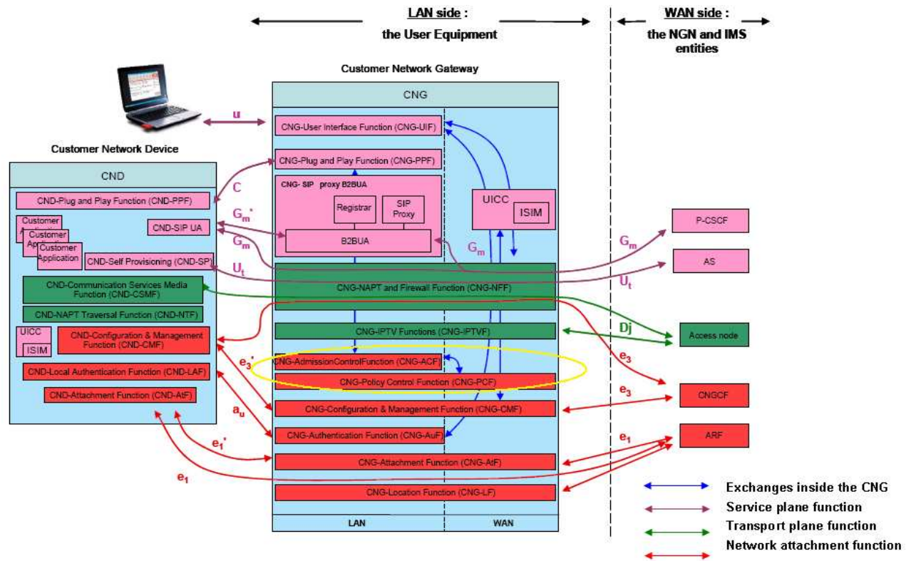
Figure 12 : Customer Network Device connecté au réseau NGN-IMS à travers un CNG
