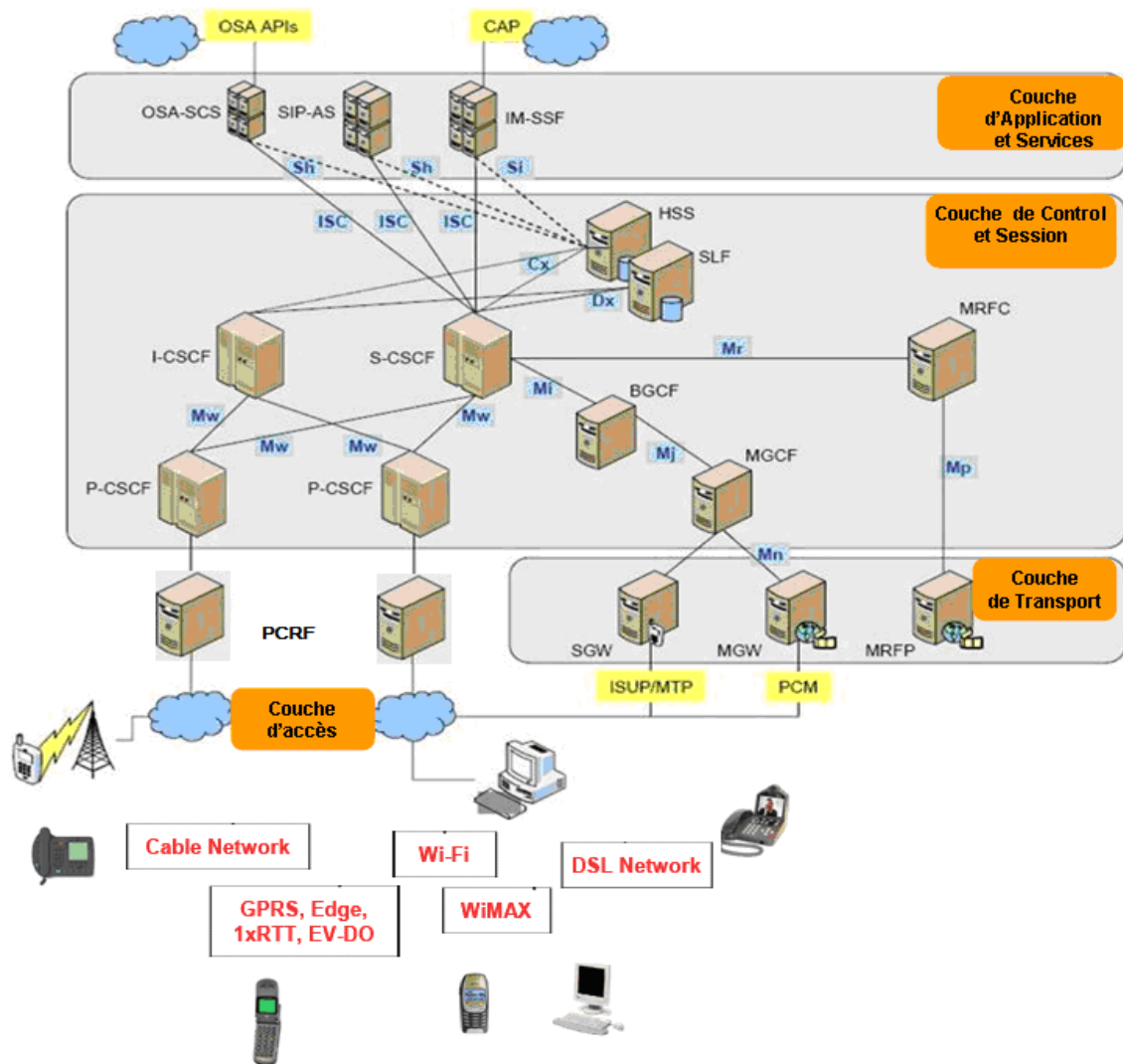
Figure 10 : Couches de l'IMS
