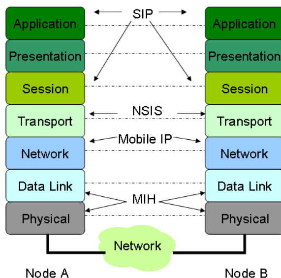
Figure 19 : Les travaux existants dans le plan de contrôle
