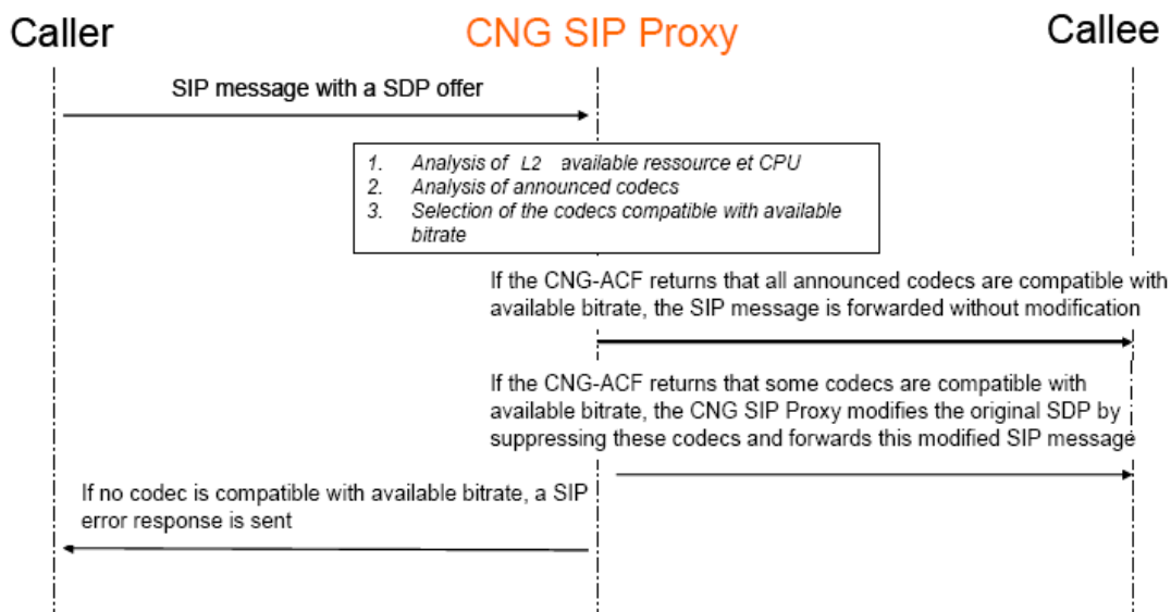
Figure 13 : Contrôle d'admission dans le CNG
