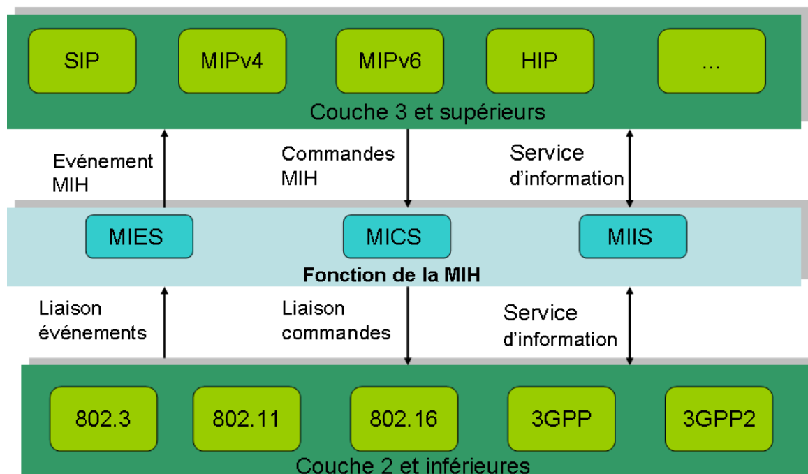
Figure 21: L'architecture du MIH
