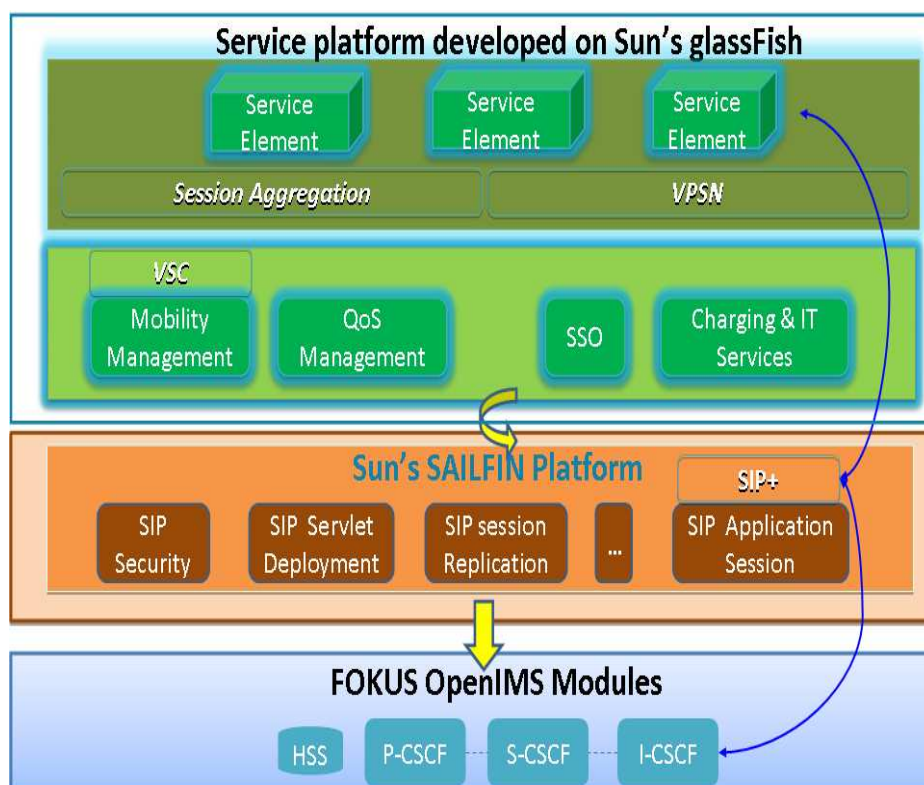
Figure 66 : La plate-forme d'implémentation
