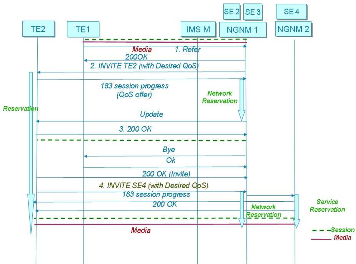
Figure 63 : Mobilité d'utilisateur
