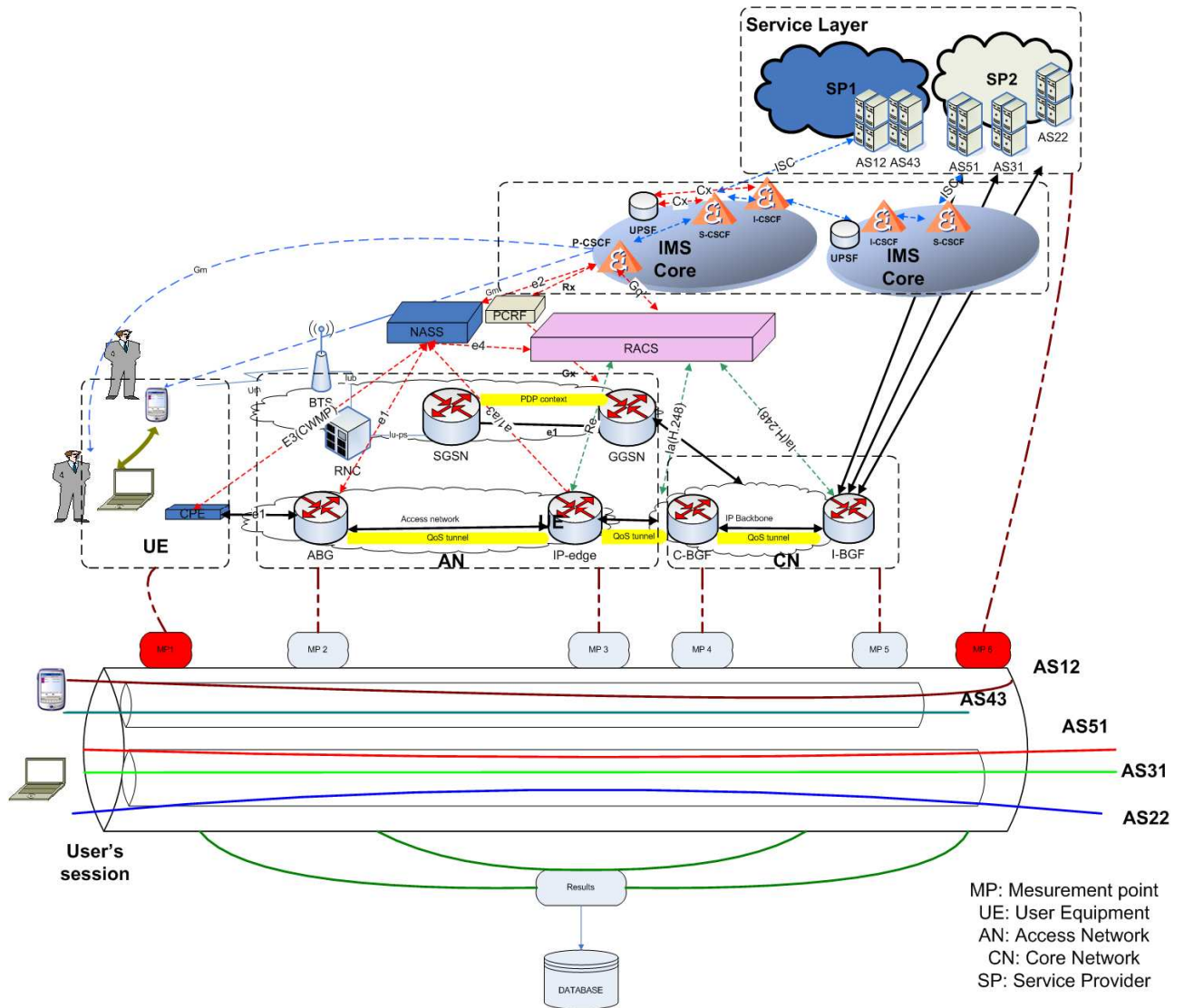
Figure 61: Les mesures de QoS de transfert de média
