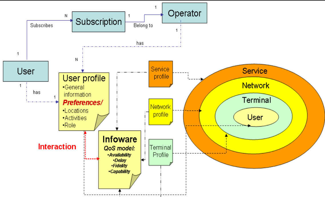
Figure 55 : Interaction avec les autres acteurs et profils
