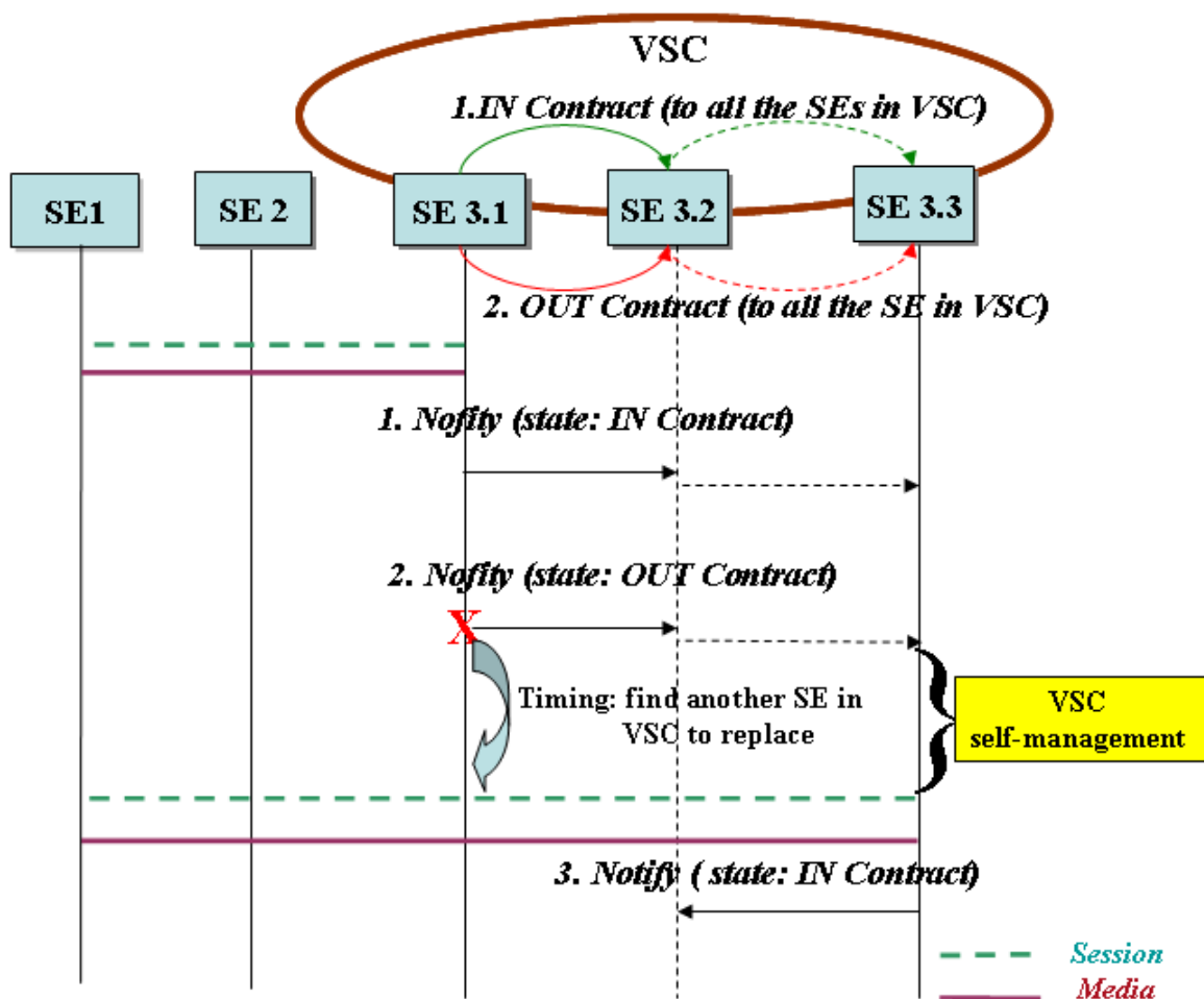
Figure 64 : Mobilité de la session
