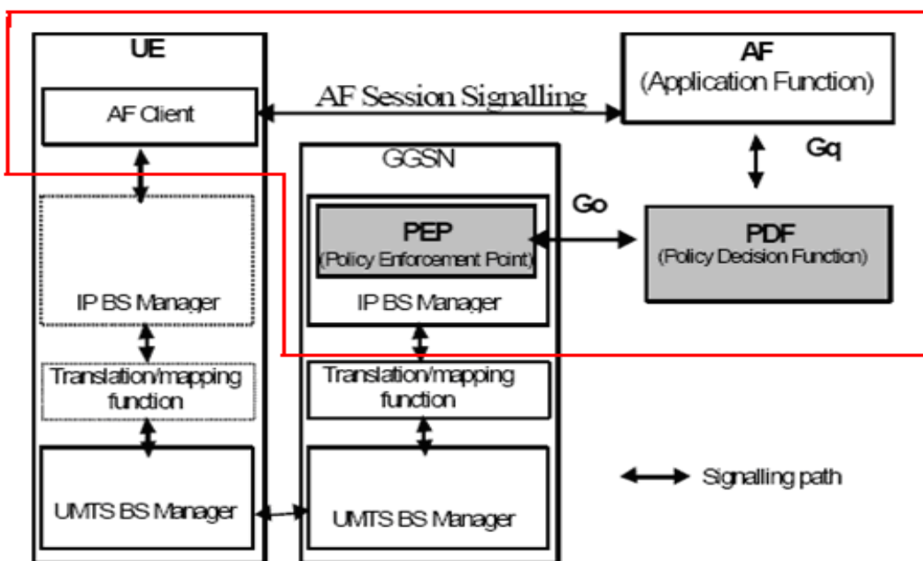
Figure 14 : L'architecture de gestion par politique dans l'IMS de 3GPP [12]
