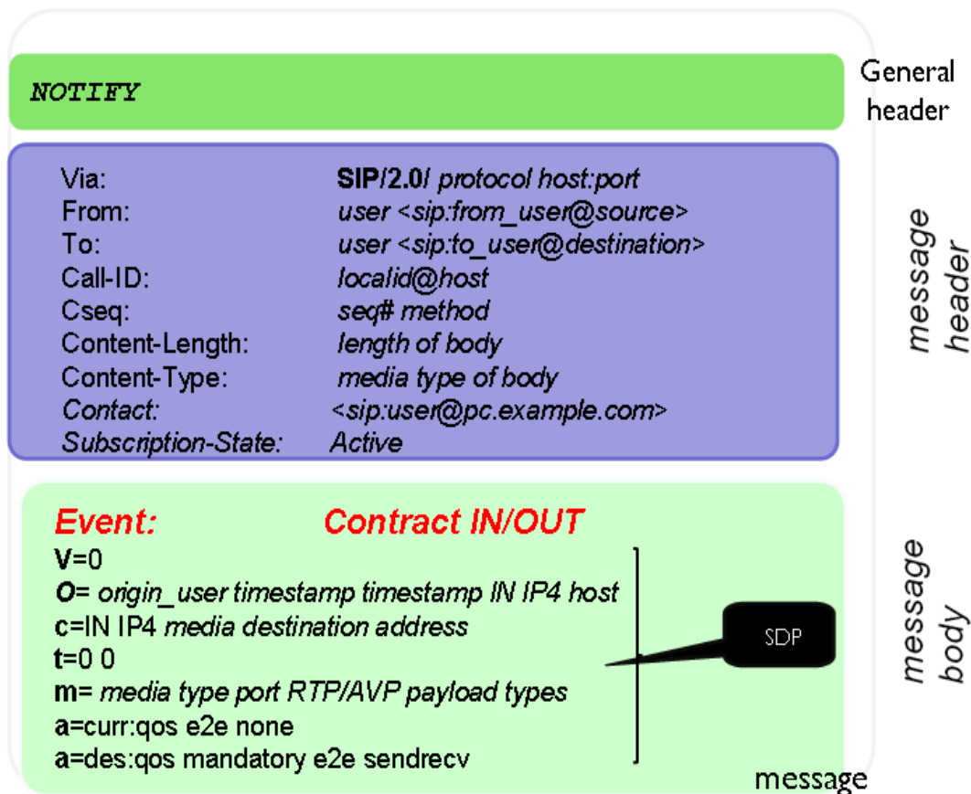
Figure 65 La structure du message SIP NOTIFY
