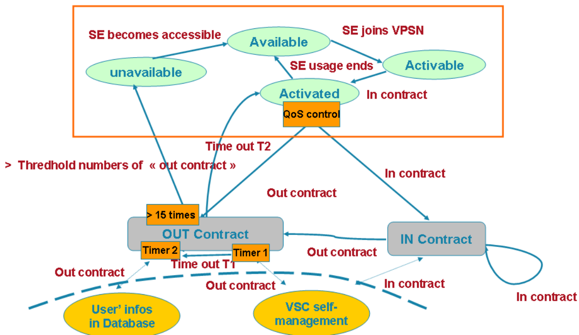
Figure 44 : Automate de gestion des composants de service
