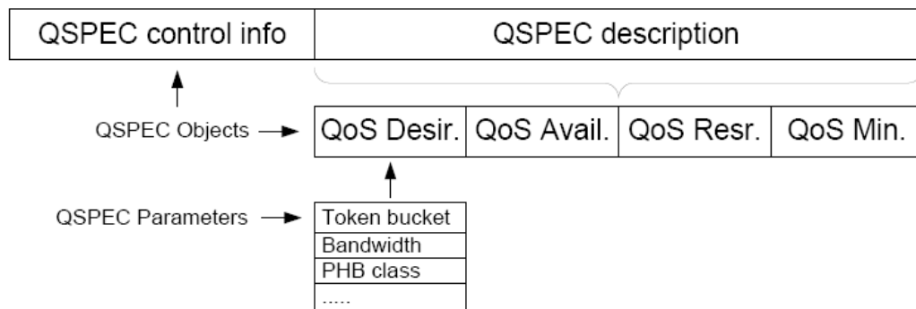
Figure 26: Modèle de Q SPEC
