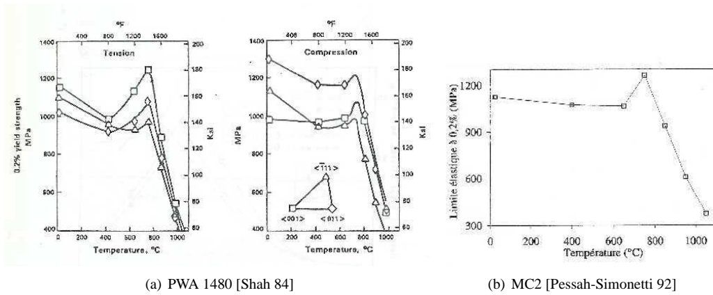
FIG. 2.4. Limite élastique de superalliages base nickel en fonction de la température.
