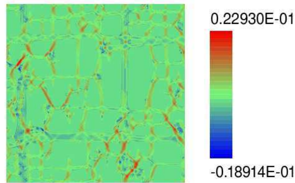
FIG. 5.31. Déformation plastique \varepsilon_{11}^p après 15.5 h de fatigue à 1050^\circ\text{C} .
