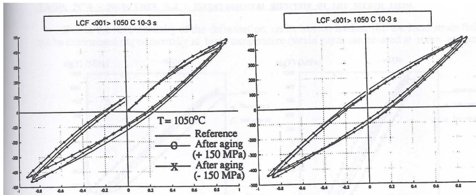
FIG. 4.9. Influence de la mise en radeaux sur le comportement mécanique à 1050^{\circ}\text{C} , résultats issus du projet BRITE EURAM [Olschewski 95].
