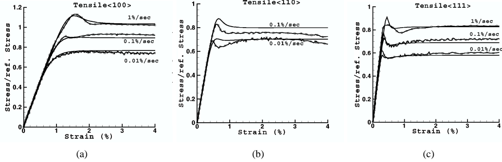
FIG. 2.1. Modèle de Levkovitch, comparaison expérience/simulation en traction monotone à 950^\circ\text{C} pour différentes orientations cristallographiques, d'après [Levkovitch 06].
