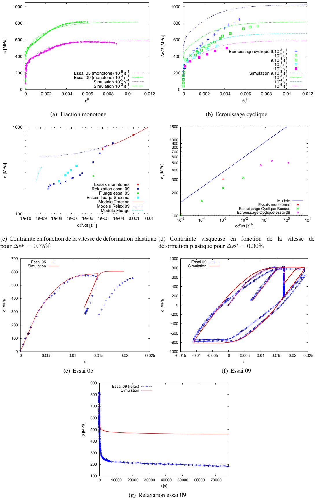
FIG. 2.12. Résultats du modèle de comportement actuel recalé sur la plage de vitesses 10^{-5} - 10^{-3} s ^{-1} . Les coefficients matériau correspondants sont donnés par le tableau 2.3.
