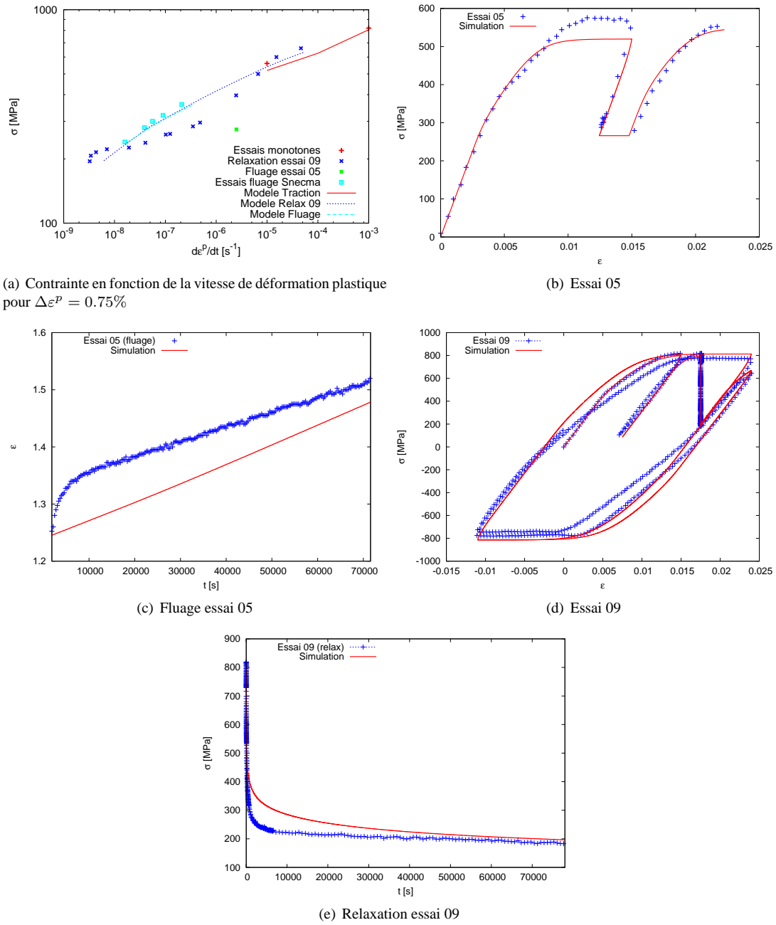
FIG. 2.19. Modèle n°2 de type Norton à deux potentiels. Ajout d'un potentiel de restauration statique. Les coefficients matériau correspondants sont donnés par le tableau 2.6.
