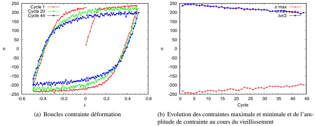
FIG. 4.29. Vieillissement cyclique à \dot{\epsilon} = 10^{-5} \text{ s}^{-1} à 1050°C pendant 24h suivant l'orientation \langle 011 \rangle (essai 20).
