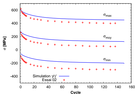
FIG. B.2. Simulation de l'essai 02.
