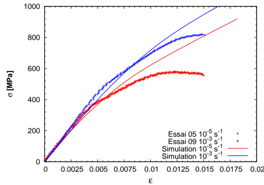
FIG. 3.8. Identification des paramètres des systèmes octaédriques de la phase \gamma à 950°C à partir d'essais de traction suivant \langle 001 \rangle à 10^{-5} s^{-1} et 10^{-3} s^{-1} .
