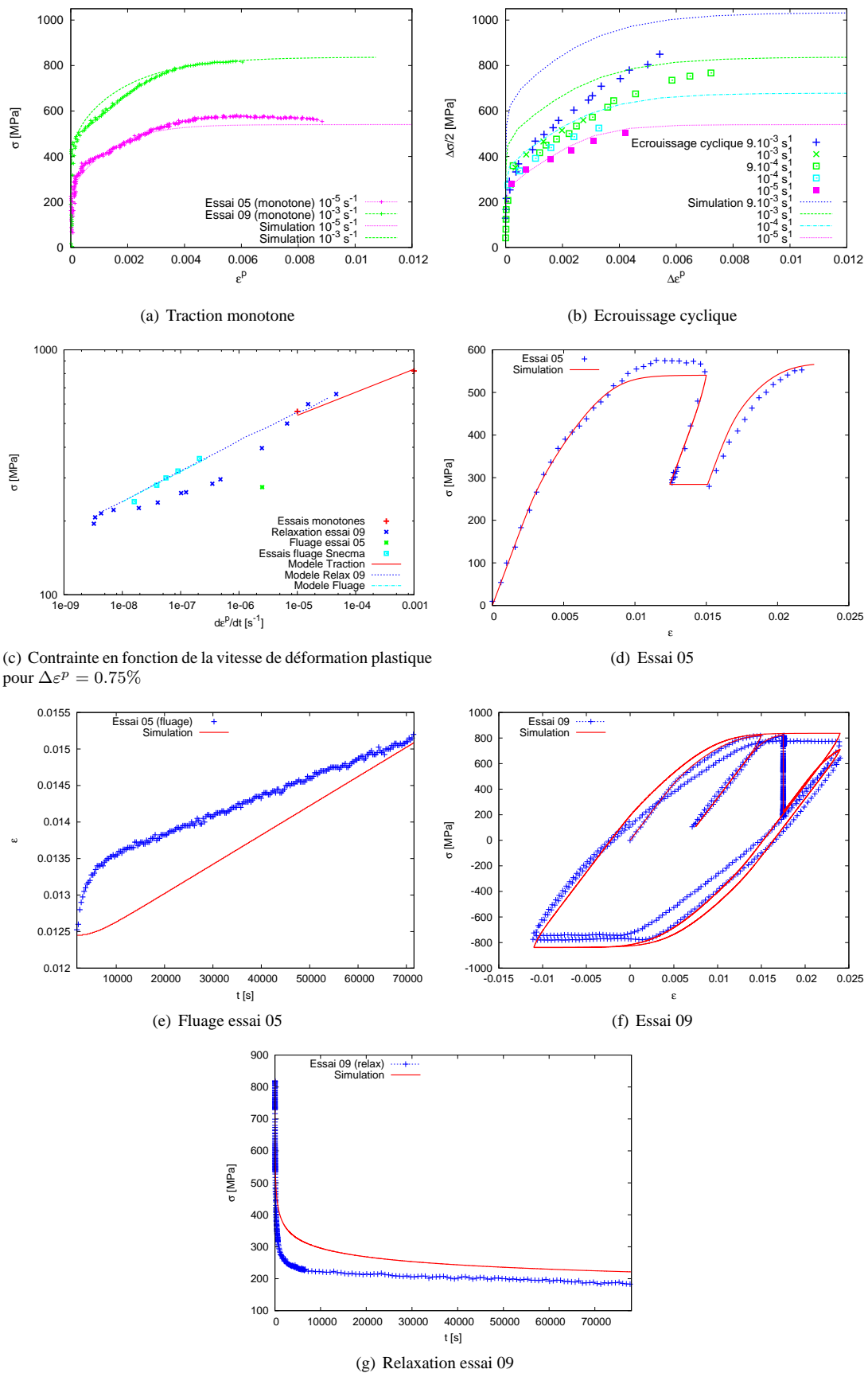
FIG. 2.15. Modèle de type Norton, ajout d'un terme de restauration statique.
