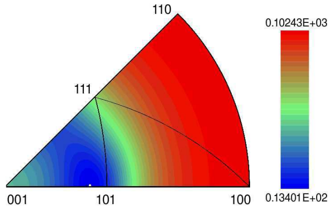
(c) Déformation plastique \varepsilon^p = 0.02
