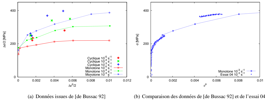
FIG. D.7. Comparaison des comportements monotone et cyclique de l'AM1 à 1100°C.
