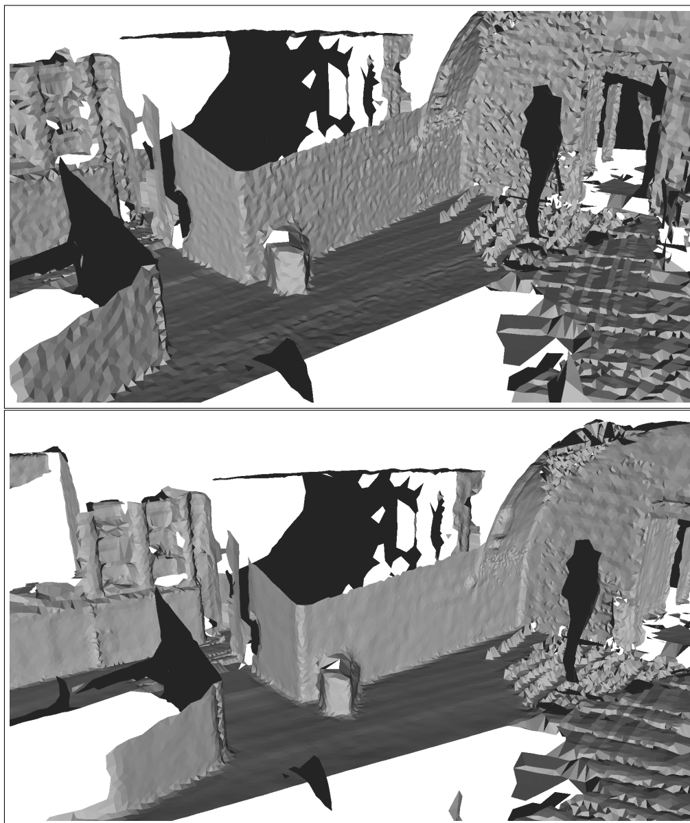
FIGURE 6.22 – En haut, maillage du nuage MINES_Rover_Indoor sans débruitage. En bas, maillage du même nuage après débruitage sans simplification.
