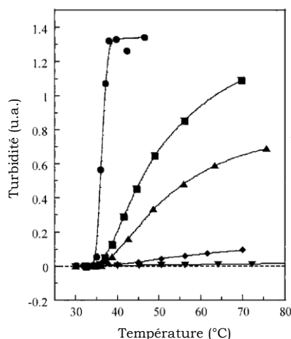
Figure 18 : Influence de la température sur la turbidité de solution aqueuse à 10 \text{ g.mL}^{-1} de \text{P(NIPAM}_{95}\text{-MADAP}_5) dans différents état d'ionisation. Le taux d'ionisation est variable : 0 (●), 0,0125 (■), 0,025 (▲), 0,035 (◆) et 0,05 (▼). D'après Bokias et al 55 .
