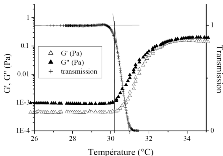
Figure 3 : Mesures de transmission et de rhéologie sur un échantillon de PNIPAM ( C_p = 1 %) à des rampes de 0,013 ( \Delta et \blacktriangle ) et 0,1°C/min (+). D'après C. Balu 29 .
