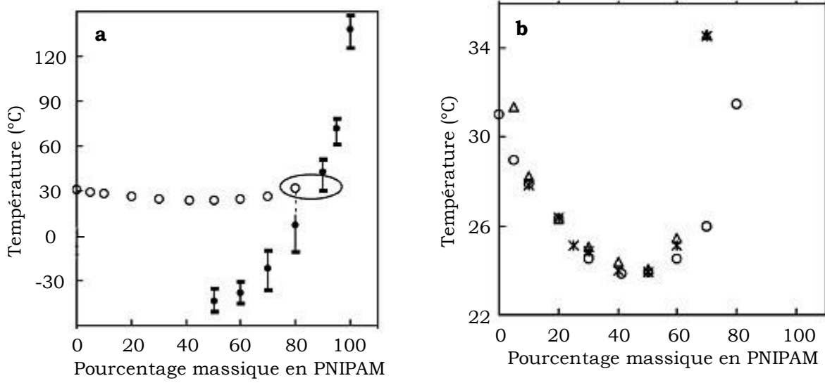
Figure 6 : Diagrammes de phase du mélange binaire PNIPAM/eau. a : Courbes de démixture (O) et transition vitreuse de solution de PNIPAM ( M = 74 \text{ kg/mol} ) - b : Courbes de démixture de solutions aqueuses de PNIPAM de masses différentes : M = 18 \text{ kg/mol} ( \Delta ); M = 74 \text{ kg/mol} (O) et M = 187 \text{ kg/mol} ). D'après Van Durme et al 34 .
