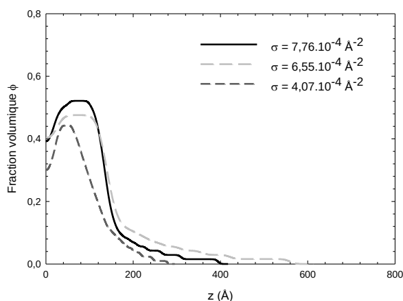
Figure 19 : Profils de fraction volumique de brosses de PNIPAM de masse M_n = 121\,000\text{ g.mol}^{-1} de densités de greffage \sigma = 7,76.10^{-4}\text{ Å}^{-2} , \sigma = 6,55.10^{-4}\text{ Å}^{-2} et \sigma = 4,07.10^{-4}\text{ Å}^{-2} dans l'eau lourde à 60°C.
