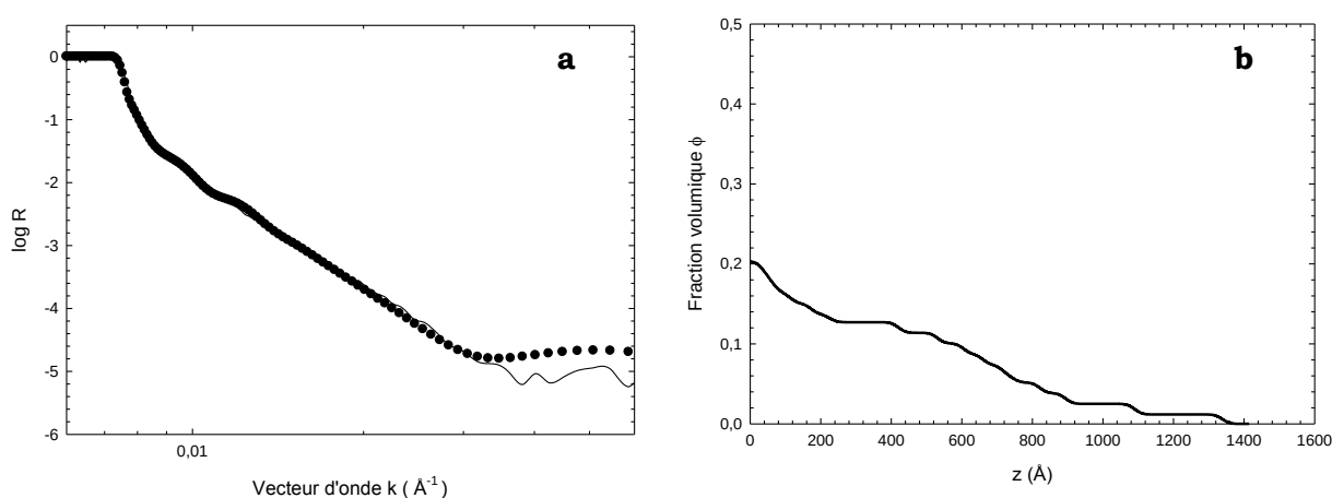
Figure 10 : Courbe de réflectivité de neutrons (a) et profil de fraction volumique correspondant (b) d'une brosse de PNIPAM ( M_n = 121\,000\text{ g.mol}^{-1} et \sigma = 7,76 \cdot 10^{-4}\text{ \AA}^{-2} ) dans l'eau lourde à température ambiante.
