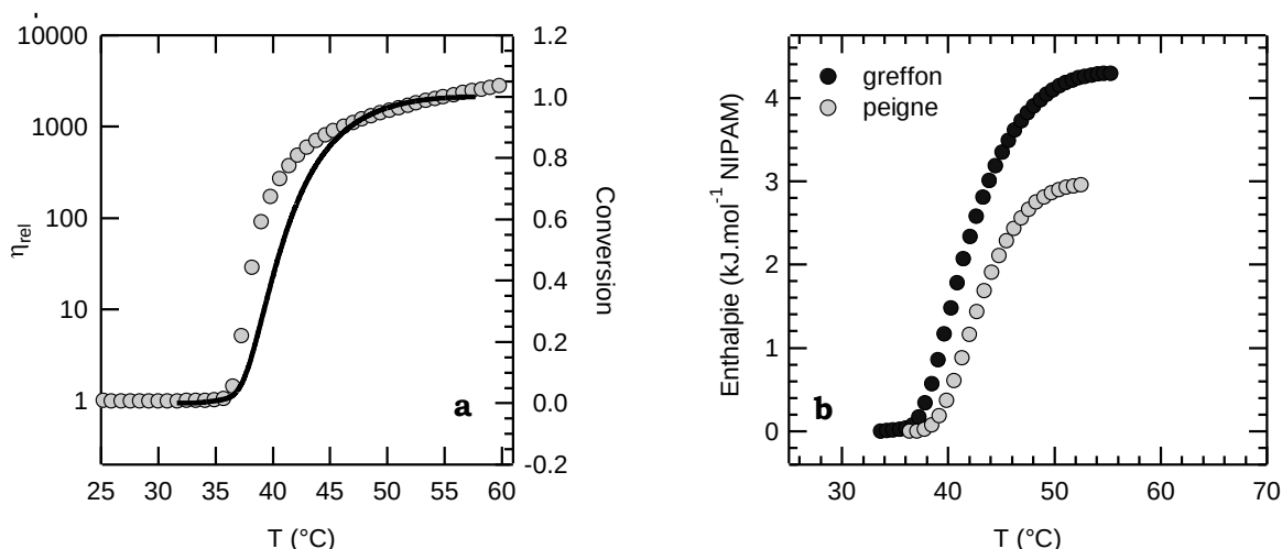
Figure 9 : a : Evolution en fonction de la température de la viscosité relative (●) et de la conversion (-) issue des analyses de DSC pour le PAM- g -PNIPAM- b ( C_p = 80 \text{ g.L}^{-1} ) – b : Comparaison des courbes enthalpiques pour les greffons PNIPAM- a ( C_p = 10 \text{ g.L}^{-1} ) et le PAM- g -PNIPAM- a ( C_p = 20 \text{ g.L}^{-1} ).
