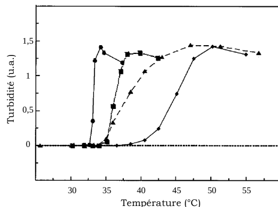
Figure 17 : Influence de la température sur la turbidité de solutions aqueuses à 10 \text{ g.mL}^{-1} de \text{P(NIPAM}_{(1-x)}\text{-MADAP}_x) sous forme basique. x = 0 (●), 5 (■), 10 (▲) et 25 % molaire (◆). D'après Bokias et al 55 .
