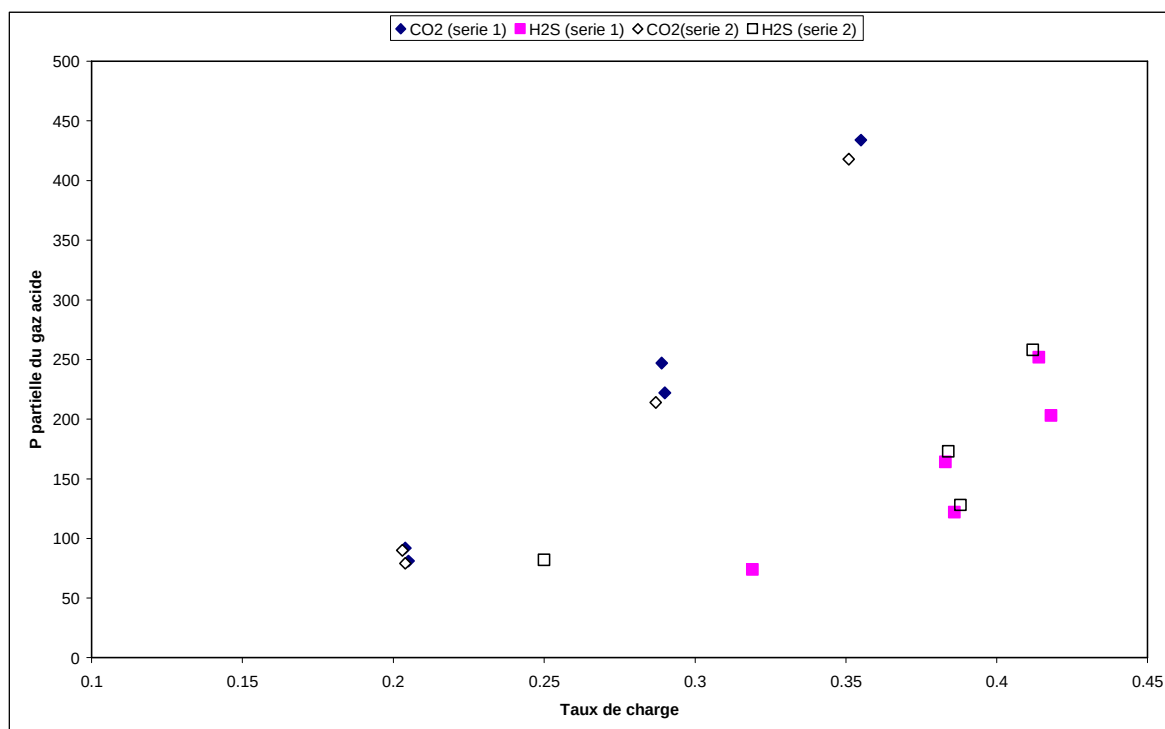
Figure I.20: Solubilité des mélanges CO 2 +H 2 S dans le mélange 40% masse Eau- 30% masse DEA- 30% masse Méthanol à 343.5K (Blanchon Le Bouhelec-Tribouillois, 2006 )
