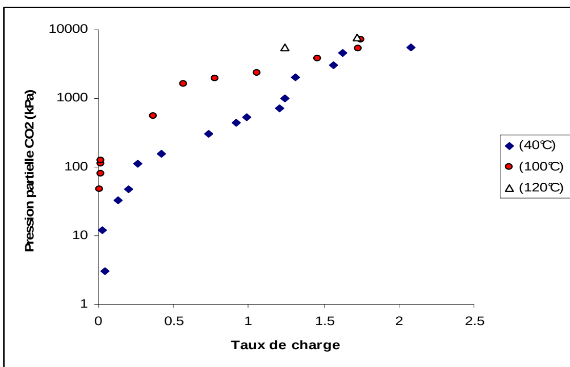
Figure I.18: Effet de la température sur la solubilité de \text{CO}_2 dans le mélange 40%masse MDEA-40%masse \text{CH}_3\text{OH} -20%masse \text{H}_2\text{O}
