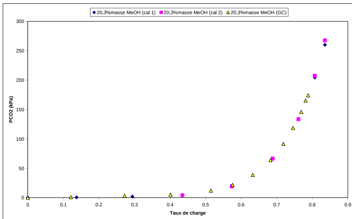
Figure III.25: Comparaison de la solubilité de \text{CO}_2 dans le système 30%masse DEA-20%masse MeOH-50%masse \text{H}_2\text{O}
