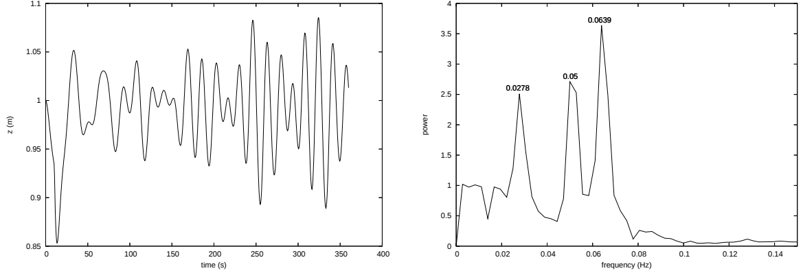
FIG. 4.5 – Altitude d'un point de l'interface en fonction du temps et transformée de Fourier associée, pour B_{0,z} = 280\text{ G} . Cette expérience numérique est effectuée en utilisant le modèle non linéaire, sur une cuve parallélépipédique avec L_x = L_y = 2m et h_1 = h_2 = 1m .
