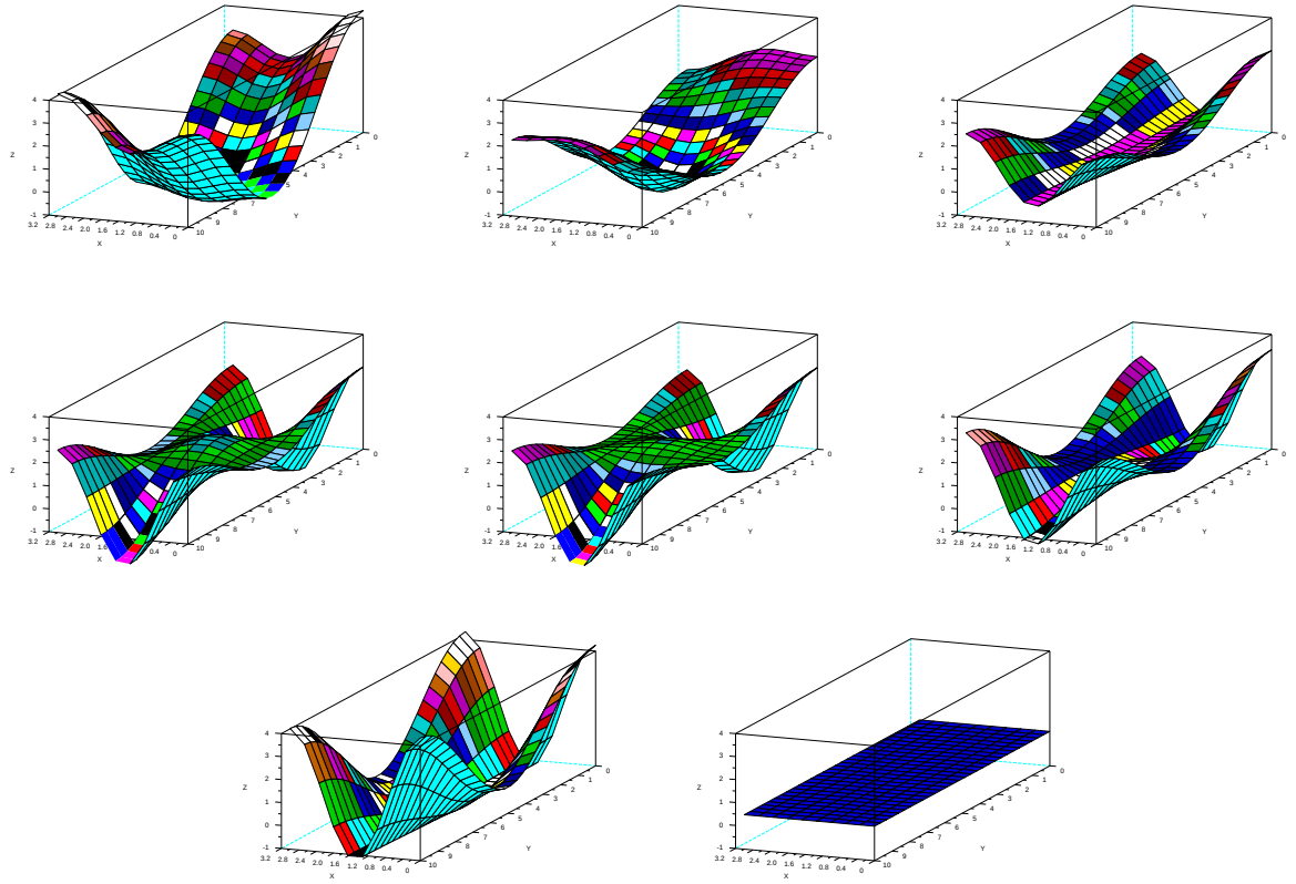
FIG. 5.20 – Commande optimale B_z(x, y) en t = 0.25, 0.5, 0.75, 1, 1.25, 1.5, 1.75 et 2 .
