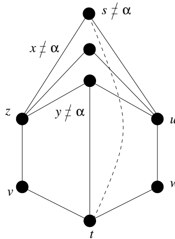
Figure C.VI – Lemme C.3, illustration pour le résultat 3.
