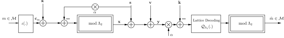
FIGURE 8 – Schéma d’encodage/décodage pour le problème de Costa utilisant deux réseaux de points imbriqués. Le réseau de points externe ( coarse lattice ) \Lambda_2 doit être un bon code source et le réseau de points interne doit être un bon code canal. \Lambda_1 should be a good channel code.
