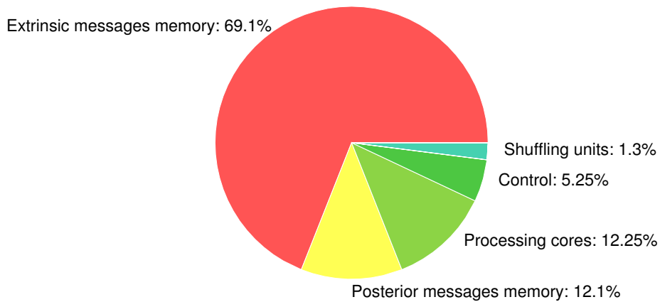
Figure A.20: Distribution de la surface du décodeur implémenté.
