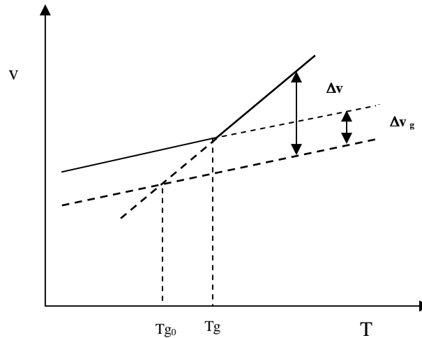
Figure 22 : Variation du volume spécifique v avec la température T
