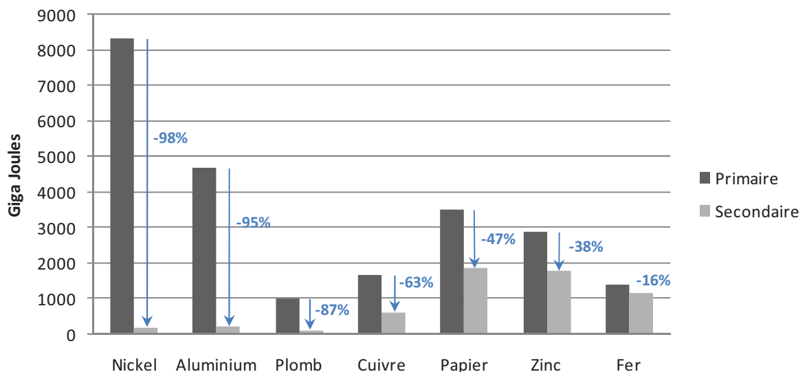
Figure 6 : Quantités d'énergie nécessaire à la fabrication des matériaux industriels usuels, partant de sources primaires (minerais) ou secondaires (déchets). (BIR 2008)
