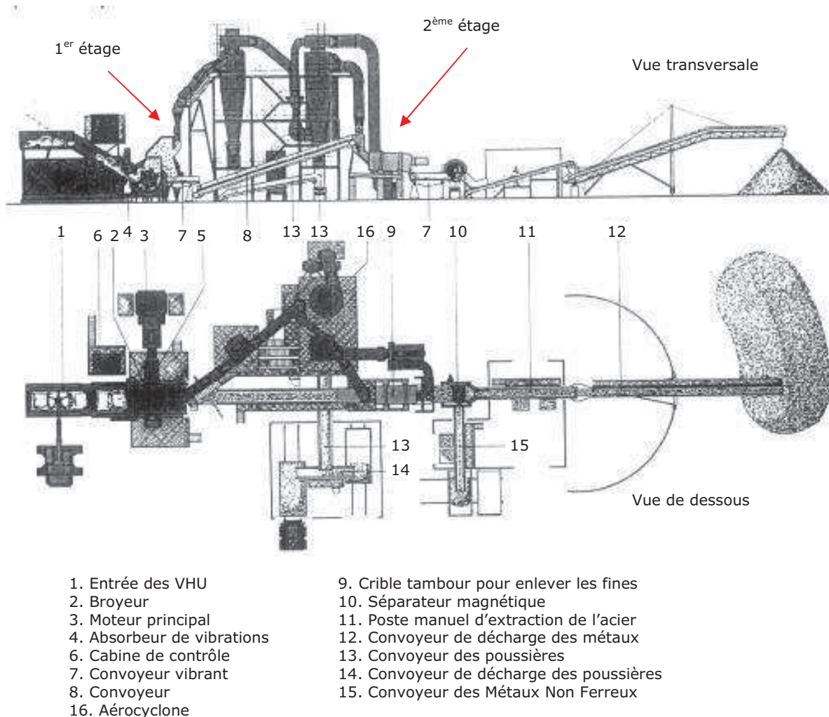
Figure 23 : Vue schématique d'une unité de broyage et tri post-broyage pour les VHU (Source METSO 2010 / NOVA CONCEPT)
