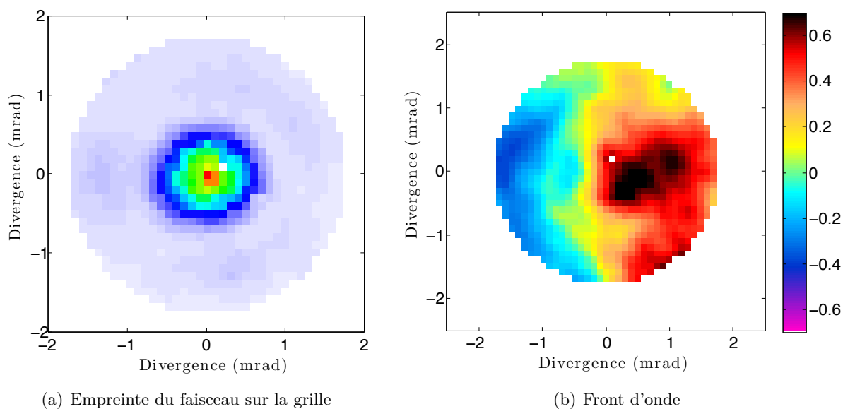
FIGURE 4.8 – Mesure du front d'onde du faisceau laser injecté par harmonique
