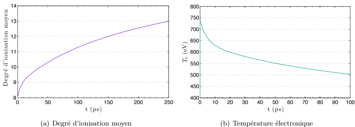
FIGURE 2.12 – Évolution temporelle de (a) l'état de charge et (b) la température électronique du plasma après ionisation par le champ laser, pour une pression initiale de krypton de 30 mbar
