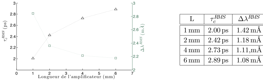
FIGURE 5.17 – Temps de cohérence et largeur spectrale quadratiques : rétrécissement spectral par le gain
