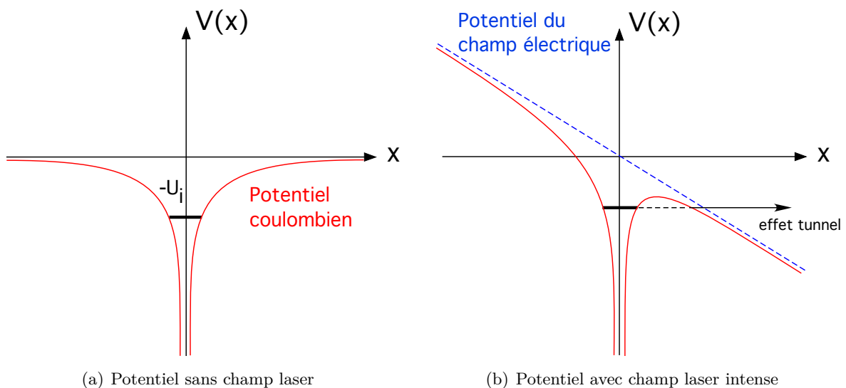
FIGURE 2.6 – Principe de l'ionisation tunnel : abaissement de la barrière de potentiel liant l'électron au noyau
