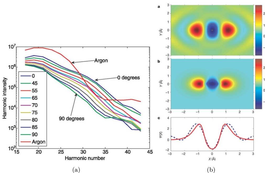
FIGURE 1.17 – (a) Les spectres harmoniques produit dans un gaz diatomique ( N_2 ) sont enregistrés pour différents angles d'alignement des molécules d'azote. L'argon sert de référence. (b) Le panneau [a] donne la reconstruction de l'orbitale moléculaire de N_2 à partir d'une inversion tomographique des spectres obtenus pour différents alignements des molécules. Le panneau [b] donne le calcul de l'orbitale 2p\sigma_g . Les échelles de couleur sont les mêmes. Le panneau [c] donne la coupe selon l'axe moléculaire de l'orbitale mesurée (pointillés) et calculée (trait plein).
