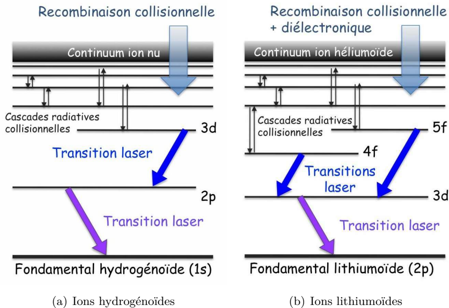
FIGURE 1.18 – Principe du schéma de recombinaison sur des espèces hydrogéoïde et lithumioïdes
