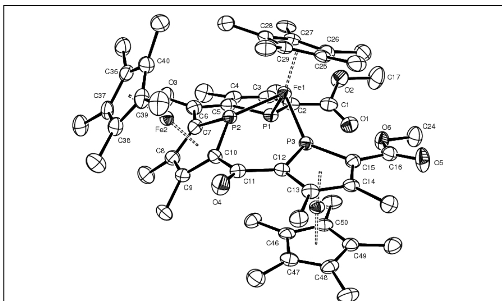
Figure IV-7 : Structure de IV-67 . Une molécule de THF omise pour raison de clarté. Ellipsoïdes à 30% probabilité. Distances et angles particuliers : Fe(1)-P(2) 2.149(1); Fe(1)-P(3) 2.192(1); Fe(1)-P(1) 2.276(1); Fe(2)-P(2) 2.292(1); Fe(3)-P(3) 2.236(1); angle entre les plans P(3)C 4 -P(2)C 4 41.7°; P(2)C 4 -P(1)C 4 47.2°.
