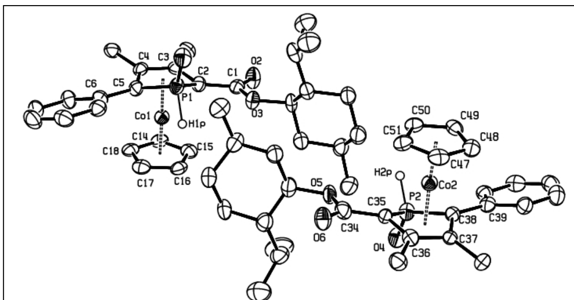
Figure II-3 : Structure RX du mélange de diastéréoisomères II-6a et II-6b . Méthyles des Cp* omis pour raisons de clarté. Sauf mention contraire, les représentations des structures RX seront toujours constituées d'ellipsoïdes à 50% de probabilité. Distances particulières : Co(1)-C(3) 1.984(4) ; Co(1)-C(4) 2.023(5) ; Co(1)-C(15) 2.044(5) ; Co(1)-C(2) 2.053(5) ; Co(1)-C(16) 2.065(5) ; Co(1)-C(5) 2.065(5) ; Co(1)-C(17) 2.066(4) ; Co(1)-C(18) 2.073(5) ; Co(1)-C(14) 2.080(5) ; Co(1)-P(1) 2.700(2) ; Co(2)-C(36) 1.979(4) ; Co(2)-C(37) 2.026(4) ; Co(2)-C(51) 2.036(5) ; Co(2)-C(50) 2.045(5) ; Co(2)-C(35) 2.055(5) ; Co(2)-C(47) 2.067(5) ; Co(2)-C(49) 2.072(4) ; Co(2)-C(38) 2.077(5) ; Co(2)-C(48) 2.078(5) ; Co(2)-P(2) 2.702(2) ; P(1)-O(1) 1.484(4) ; P(1)-C(5) 1.778(5) ; P(1)-C(2) 1.781(5) ; P(2)-O(4) 1.483(4) ; P(2)-C(35) 1.777(5) ; P(2)-C(38) 1.798(5) ; C(4)-C(3) 1.418(6) ; C(4)-C(5) 1.442(6) ; C(48)-C(47) 1.421(6) ; C(48)-C(49) 1.459(7) ; C(48)-C(53) 1.491(7) ; C(38)-C(37) 1.455(6) ; C(38)-C(39) 1.473(5) ; O(5)-C(34) 1.356(6) ; O(3)-C(1) 1.345(5) ; P(2)-H(2P) 1.39(3) Å.
