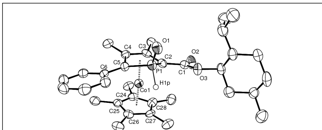
Figure II-4 : Structure RX de II-6b ( R_{Mc} ). Distances particulières : P(1)-H(1P) (H affiné) 1.40(6) ; Co(1)-C(3) 1.985(5) ; Co(1)-C(4) 2.034(5) ; Co(1)-C(2) 2.053(5) ; Co(1)-C(27) 2.055(6) ; Co(1)-C(25) 2.058(5) ; Co(1)-C(28) 2.065(6) ; Co(1)-C(26) 2.069(6) ; Co(1)-C(5) 2.075(6) ; Co(1)-C(24) 2.088(5) ; Co(1)-P(1) 2.708(1) ; P(1)-O(1) 1.485(4) ; P(1)-C(2) 1.794(5) ; P(1)-C(5) 1.803(5) ; O(2)-C(1) 1.203(6) ; O(3)-C(1) 1.361(7) ; C(1)-C(2) 1.457(8) ; C(2)-C(3) 1.450(8) ; C(3)-C(4) 1.435(8) ; C(4)-C(5) 1.450(7) ; C(5)-C(6) 1.482(7) Å.
