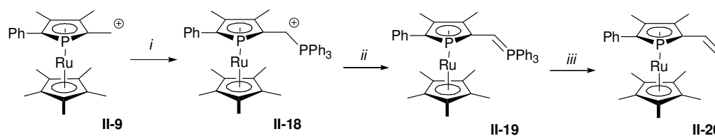
Schéma II-17 : i) PPh_3 , THF, -78^\circ C à TA ; ii) n-BuLi , -78^\circ C à TA, 45 min ; iii) HCHO, -78^\circ C à TA.
