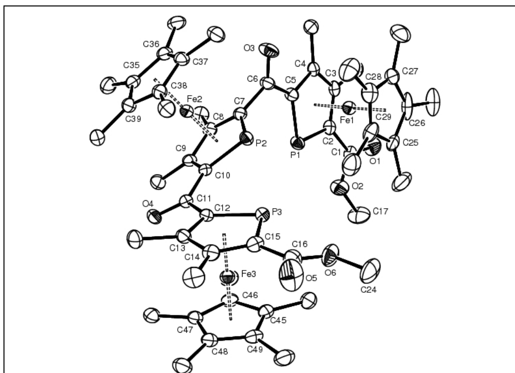
Figure IV-8 : Structure RX de IV-68 ( rac ). Deux molécules de benzène omises pour raison de clarté. Ellipsoïdes 30% probabilité. Distances et angles particuliers : Fe(1)-Ct(phospholye) 1.642 ; Fe(2)-Ct(phospholye) 1.632 ; Fe(3)-Ct(phospholye) 1.637 ; Fe(1)-Ct(Cp*) 1.673 ; Fe(2)-Ct(Cp*) 1.677 ; Fe(3)-Ct(Cp*) 1.674 Å ; angle entre les plans P(3)C 4 -P(2)C 4 36.1°; P(2)C 4 -P(1)C 4 76.7°.
