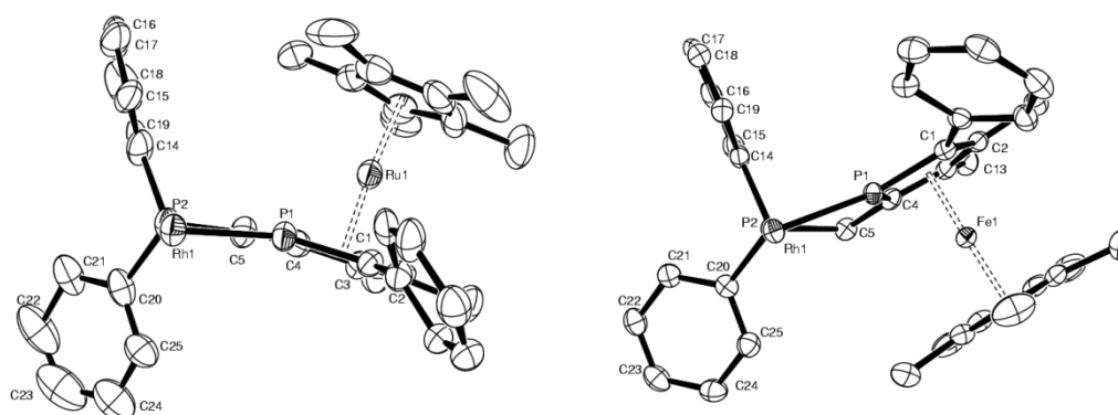
Figure II-10 : Structures RX des complexes de rhodium II-13 (M=Ru, R Mc ) et II-14 (M=Fe, S Mc ). Vue dans l'axe de la liaison P2-Rh. Les motifs Ph 2 P-Rh sont superposables, mais en inversant la chiralité plane. Le phényle encombrant au niveau du rhodium est dans les deux cas celui du haut de la figure.
