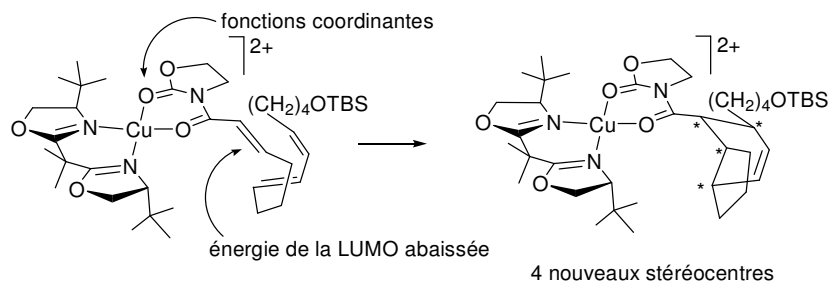
Schéma I-1 : Exemple de catalyse acide de Lewis par un complexe BOX-cuivre(II) 2
