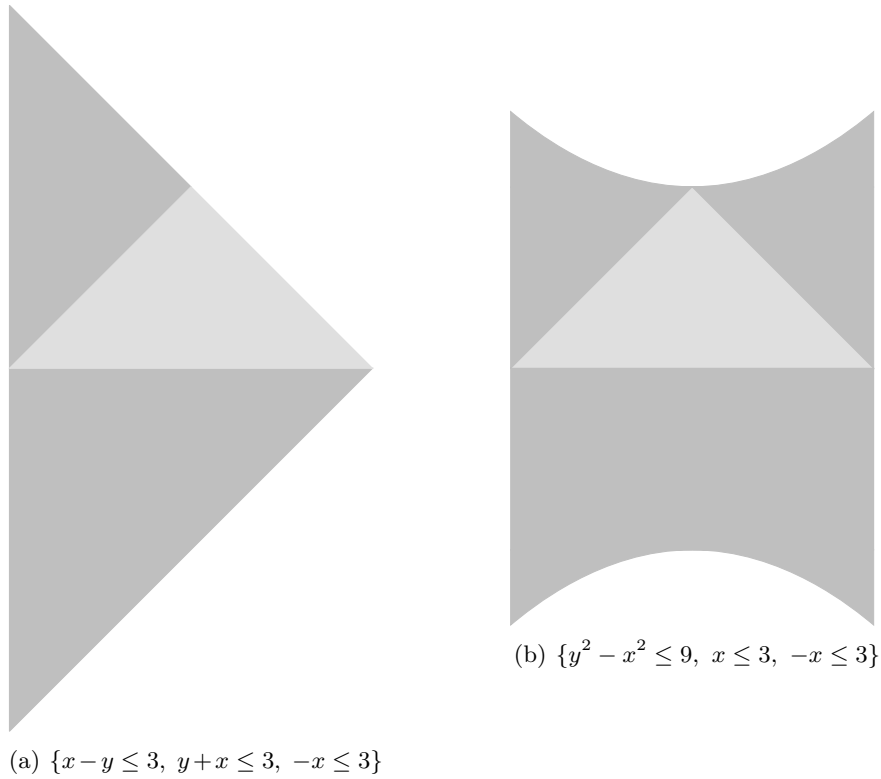
Figure 4.13 – Deux \mathbb{P} -envelopes du triangle de la figure 4.13
