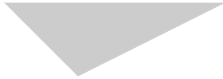
Figure 8.5 – Un cône pointé engendré par deux vecteurs non colinéaires
