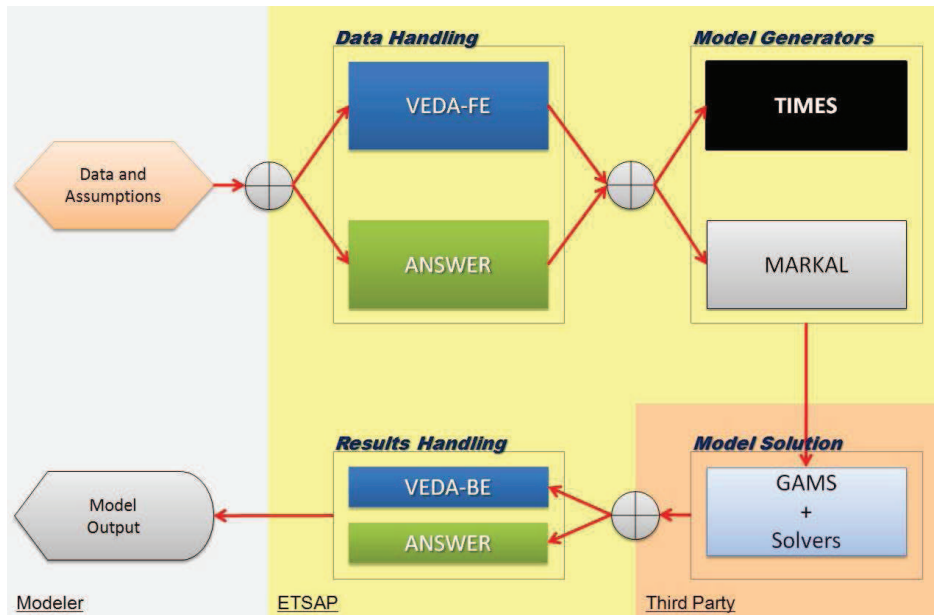
Figure 4.4 : Principe de fonctionnement de la modélisation VEDA-TIMES
