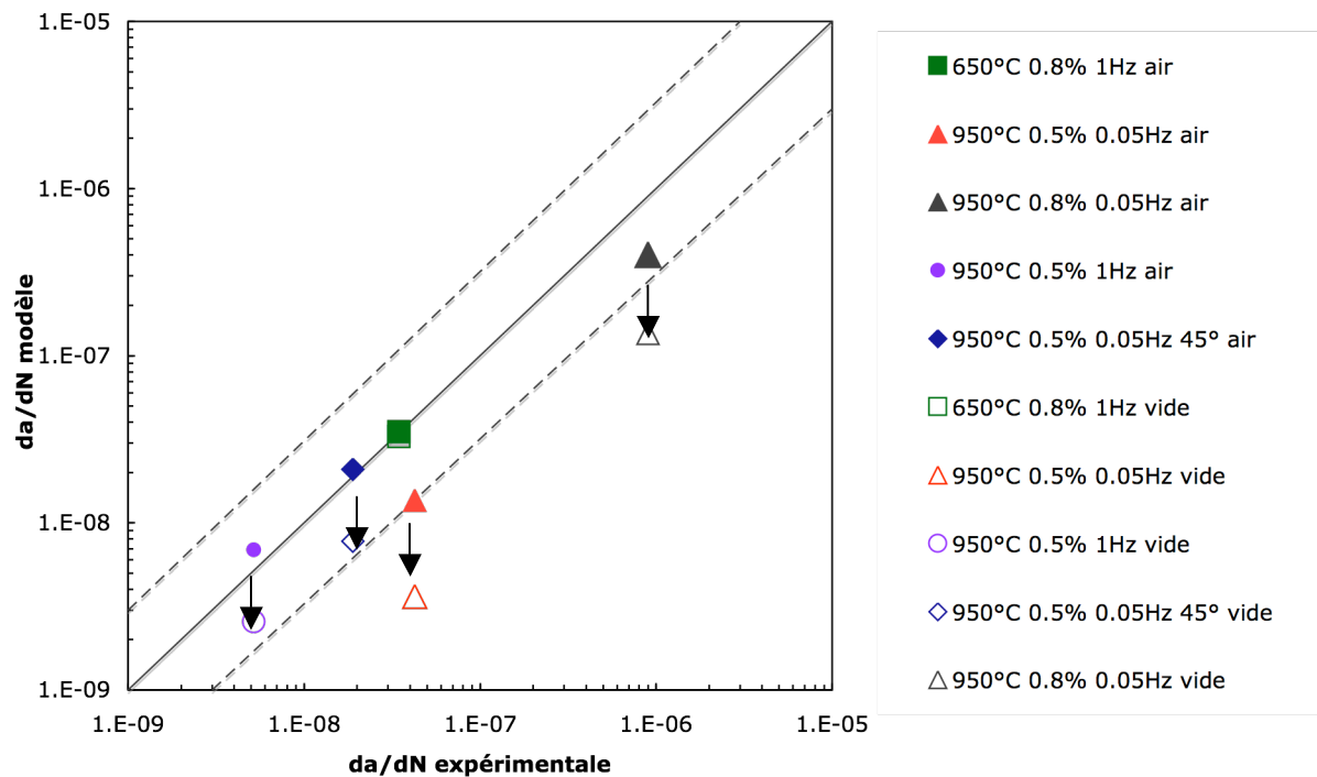
Figure 4.4-8 : Comparaison des vitesses de propagation de fissure estimées par le modèle avec les vitesses de propagation expérimentale. Influence de l'oxydation. (a=0.273mm)
