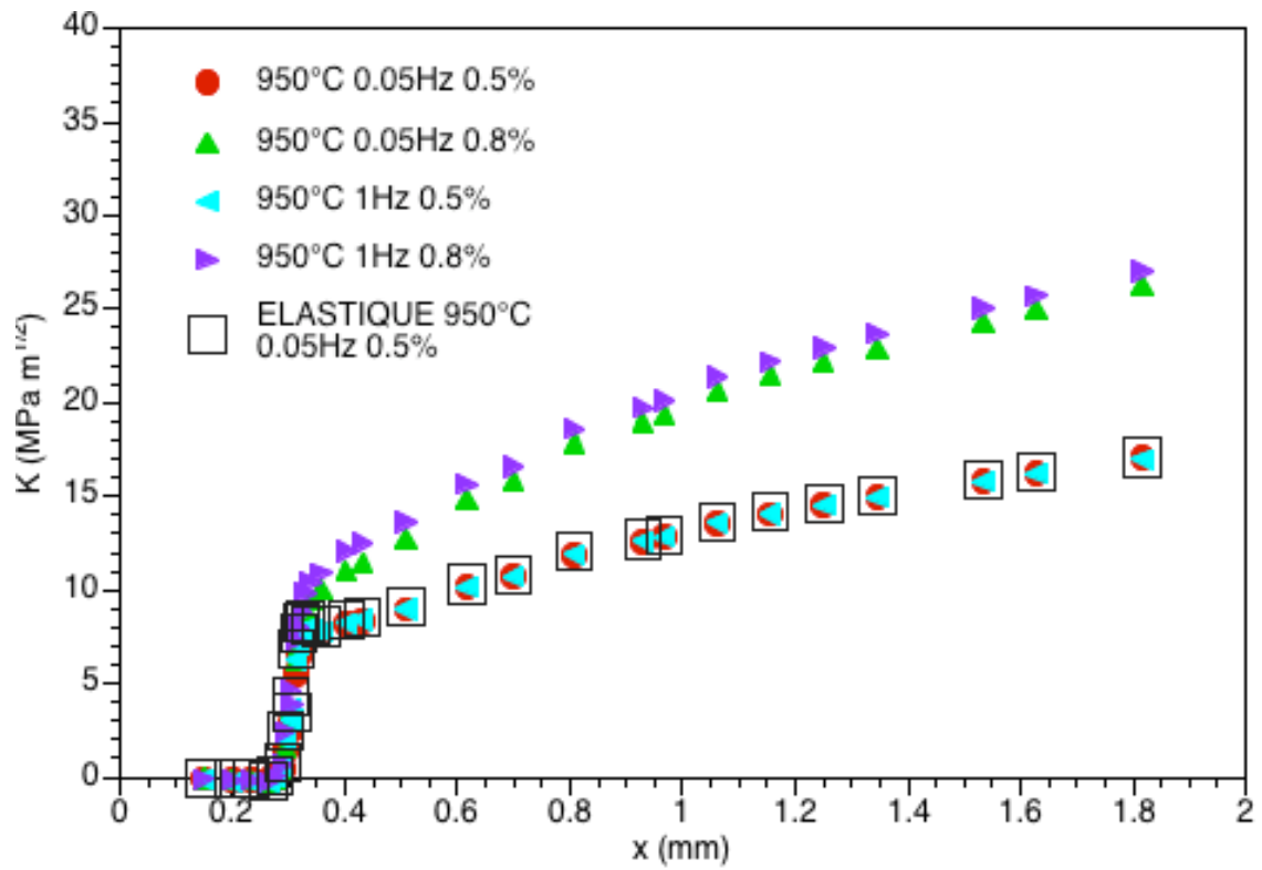
Figure 3.5-2 : Evolution du facteur d'intensité de contrainte en fonction de x à 950°C
