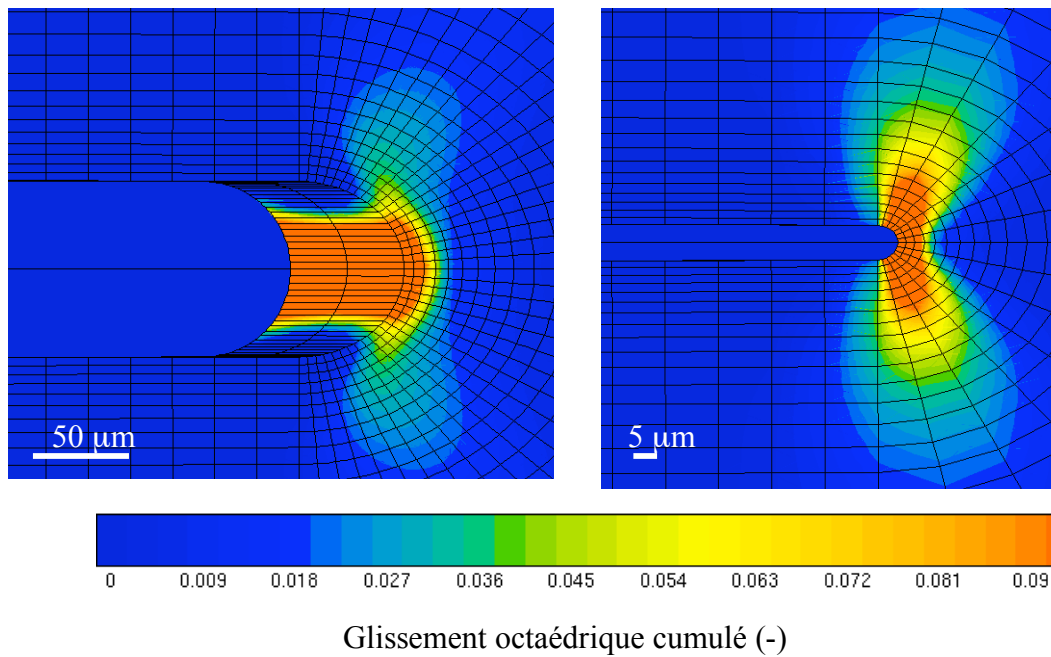
Figure 3.4-2 : Cartographie des glissements octaédriques cumulés pour entaille a) rayon 50 \mu\text{m} b) rayon 5 \mu\text{m}
