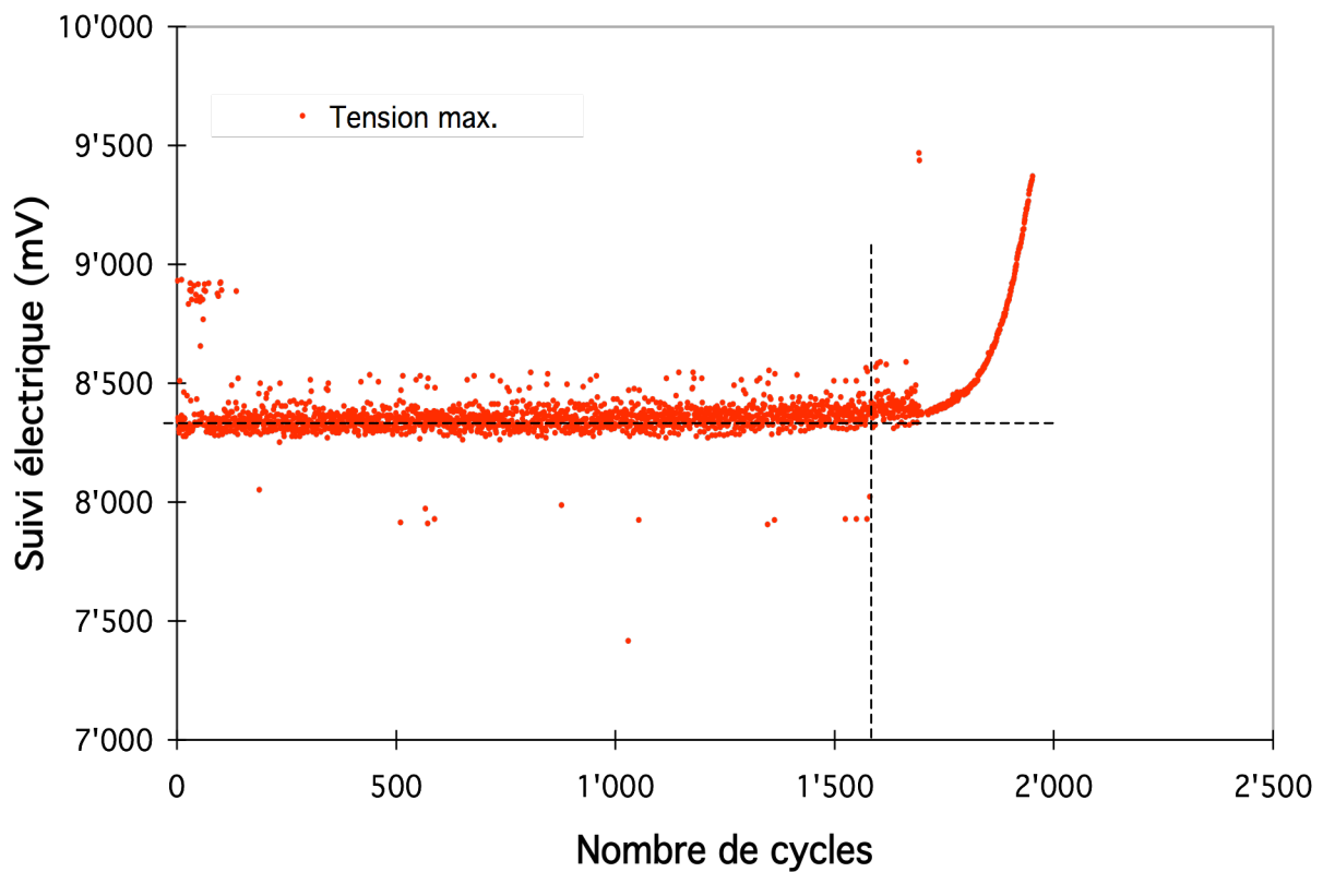
Figure 2.4-4 : Evolution du suivi électrique de la fissure dans l'éprouvette X2271D (T=950°C D_e=0.5\% f=0.05\text{Hz} )
