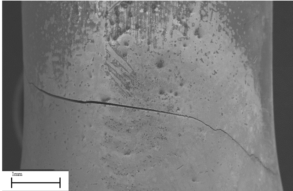
Figure 2.4-5 : Fissuration de l'éprouvette X2271D ( T=950^{\circ}\text{C} \Delta\epsilon=0.5\% f=0.05\text{Hz} )
