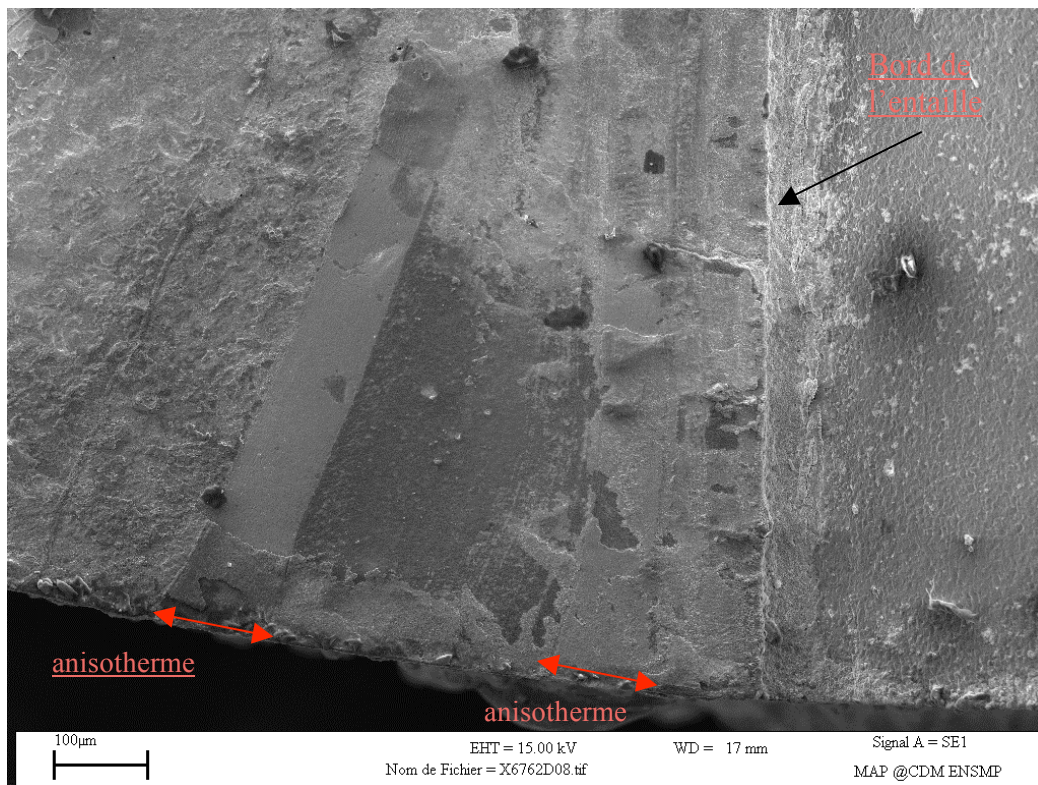
Figure 2.3-32 : Faciès de l'éprouvette X6762D isotherme / anisotheimer.
