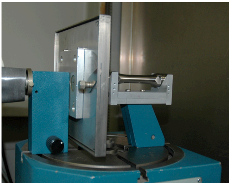
Figure 1.2-1 : Dispositif du montage de Laue en retour
