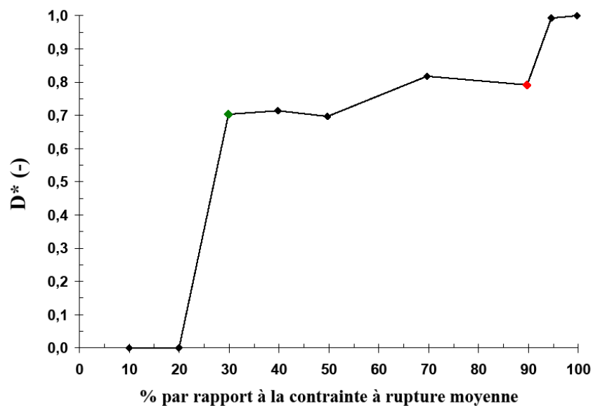
Figure IX.17 – Variable d'endommagement D^* vs pourcentage à la contrainte à rupture moyenne durant un essai de traction plane sur éprouvette de séquence 0^\circ/+45^\circ/0^\circ/+45^\circ/0^\circ/-45^\circ/0^\circ du composite tissé satin 5 carbone/PPS
