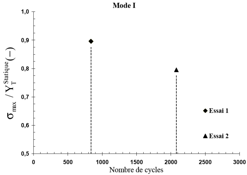
Figure X.16 – Rapport \sigma_{\max} / Y_T^{\text{Statique}} vs nombre de cycles, essais Arcan-Mines en mode I (traction) et en fatigue sur du carbone/PPS consolidé à sept plis tissés à 0^\circ
