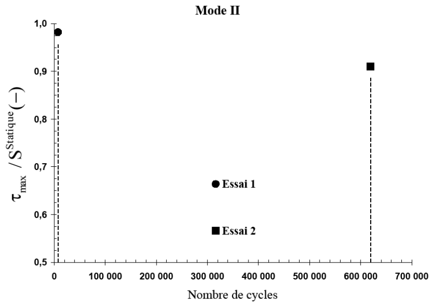
Figure X.17 – Rapport \tau_{\max} / S^{\text{Statique}} vs nombre de cycles, essais Arcan-Mines en mode II (cisaillement) et en fatigue sur du carbone/PPS consolidé à sept plis tissés à 0^\circ
