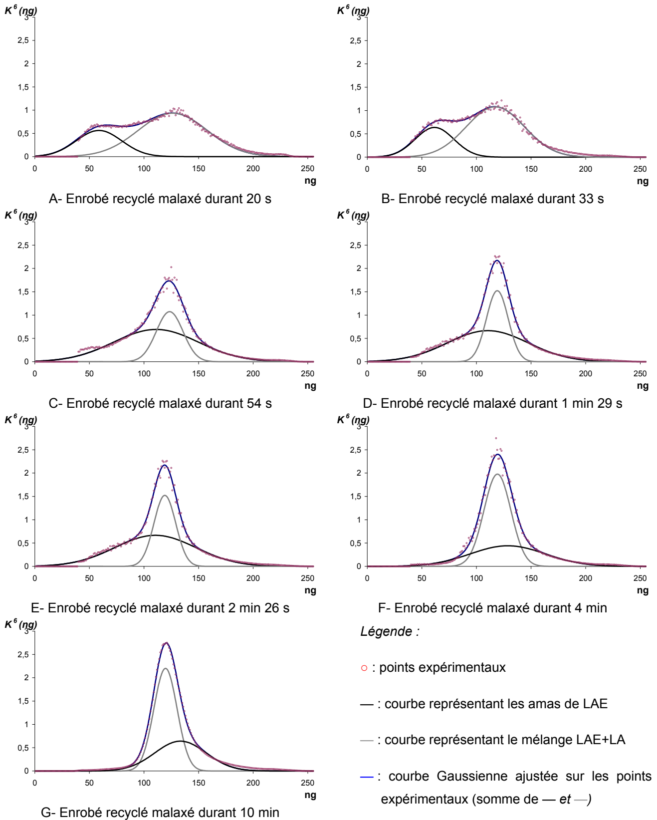
Fig. II-3 : essais de validation du protocole expérimental d'analyse d'images réalisés à partir de 6 couples de photographies pour un mélange réalisé à 130°C et un taux de recyclage égal à 70 % conditionnant une teneur en liant d'apport de 1,8 %
