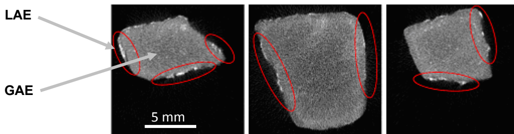
Fig. I-18 : agrégats d'enrobé artificiels enrobés par un bitume contenant des oxydes métalliques (Druta et al. 2009)
