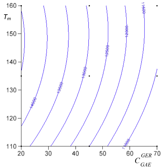
B - Courbes de niveau du module TD15°C (MPa) en fonction du pourcentage de recyclage C_{GAE}^{GER} (%) et de T_m la température de malaxage (°C) pour une durée de malaxage t_m = 140 s
