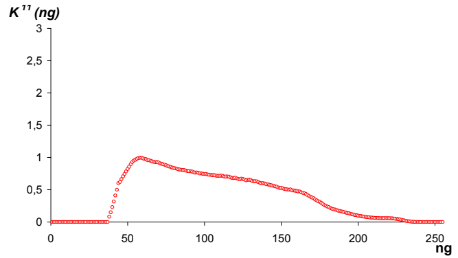
B- Enrobé recyclé malaxé durant 33 s à 110°C
