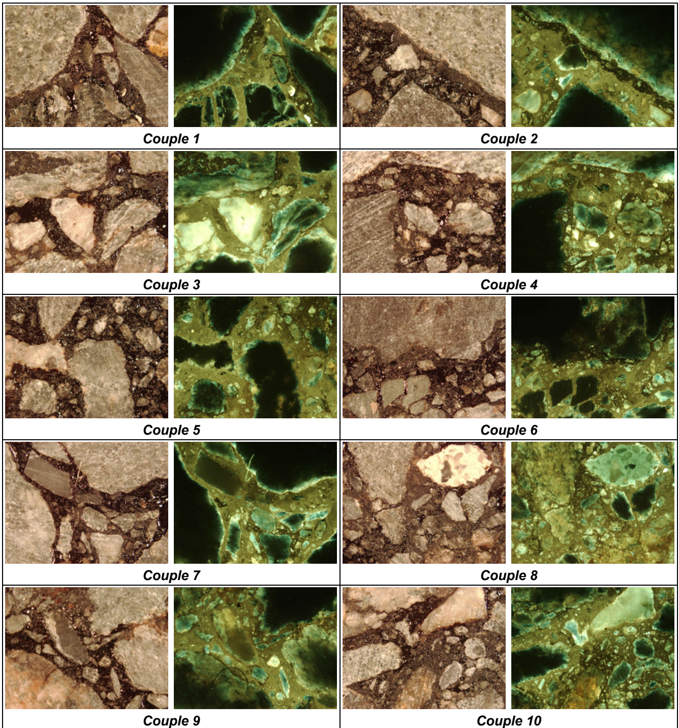
Couples de photographies sous éclairage naturel et UV caractérisant le prélèvement après 40 s de malaxage à 130°C – échantillon 2, (échelle de prise de vue 4.6*3.5 mm)
