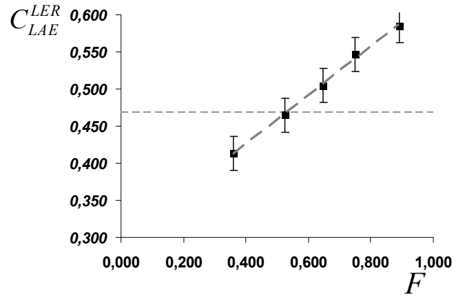
Fig. Annexe XXI-8B : Graphique corrigé présentant le résultat de la lixiviation (N°6) de l'enrobé ER_{110,40}^{45} qui se caractérise par une pente a = 0,33 \pm 0,09
