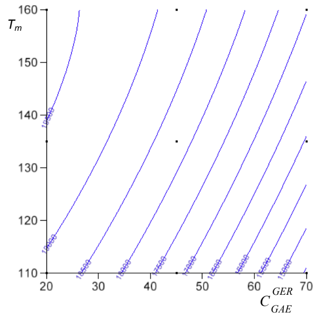
B - Courbes de niveau du module flexion 2 points à 10°C (MPa) en fonction du pourcentage de recyclage C_{GAE}^{GER} (%) et de T_m la température de malaxage (°C) pour une durée de malaxage t_m = 140 s
