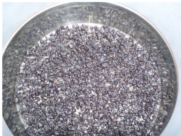
Fig. III-3 : vue du dessus de la cellule de lixiviation, en absence du système de pulvérisation, présentant un échantillon d'enrobé recyclé positionné avant lixiviation.
