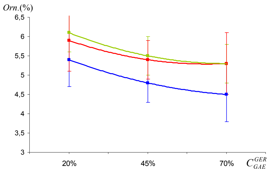
Fig. IV-8 : orniérage en fonction du pourcentage de recyclage pour une durée de malaxage de 240 s (110°C en bleu, 135°C en vert, 160°C en rouge)
