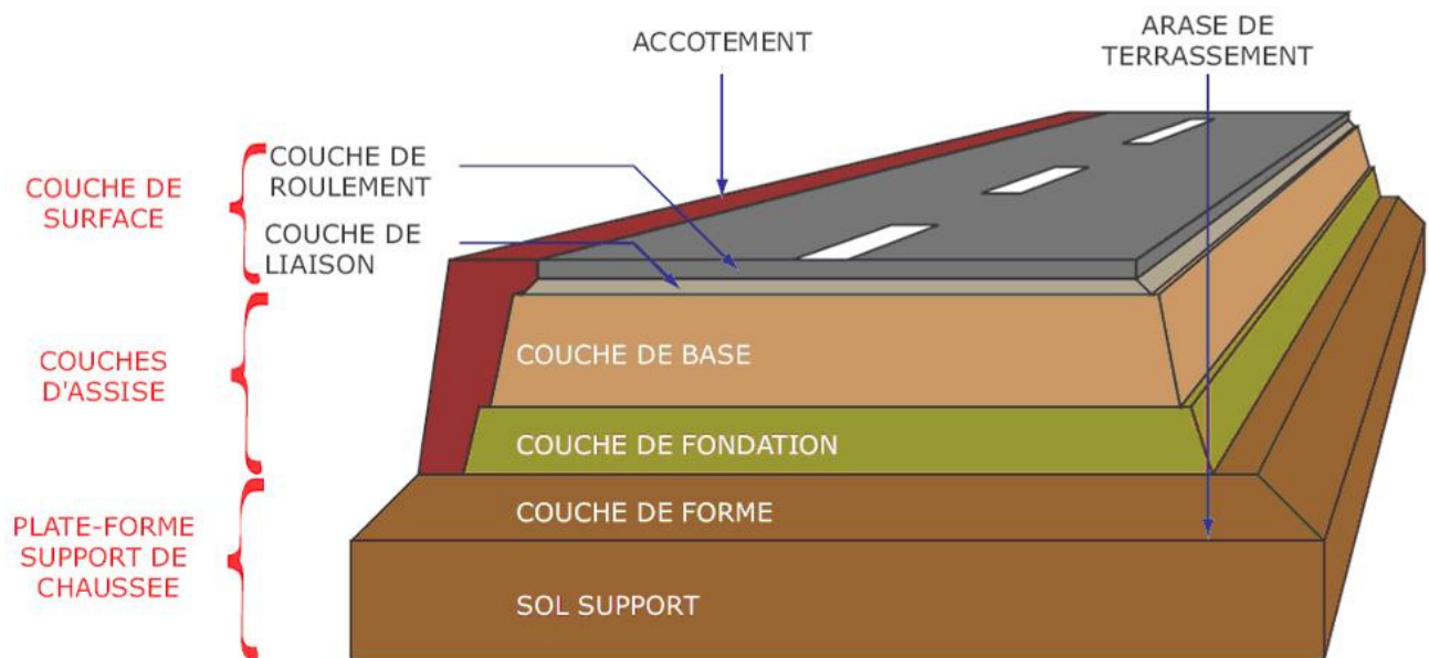
Fig. I-1 : constitution d'une structure routière (Pouteau 2004)
