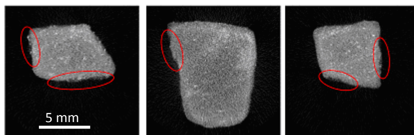
Fig. I-19 : agrégats d'enrobé artificiels après leur malaxage avec un bitume de grade 70/100 (Druta et al. 2009)
