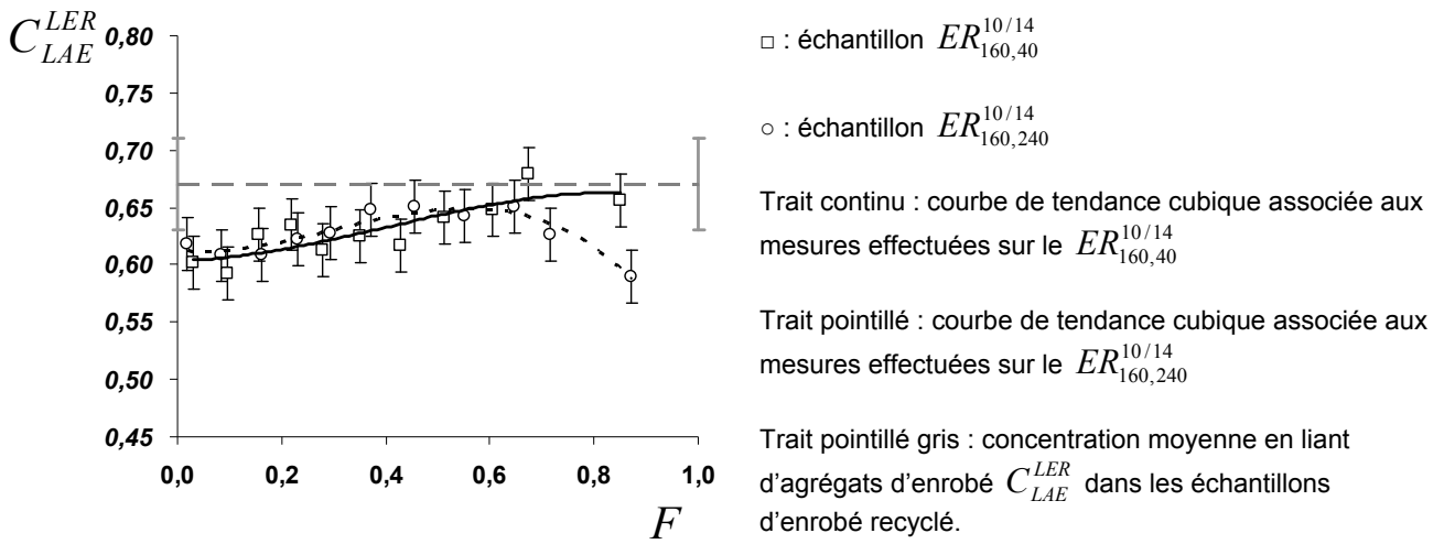
Fig. III-13 : influence de la durée de malaxage sur des enrobés recyclés fabriqués à 160°C de granulométrie 10/14 mm (échantillons ER_{160,40}^{10/14} et ER_{160,240}^{10/14} ) : évolution de la concentration C_{LAE}^{LER} en liant d'agrégat d'enrobé dans le liant lixivié en fonction de la fraction massique F de liant lixivié
