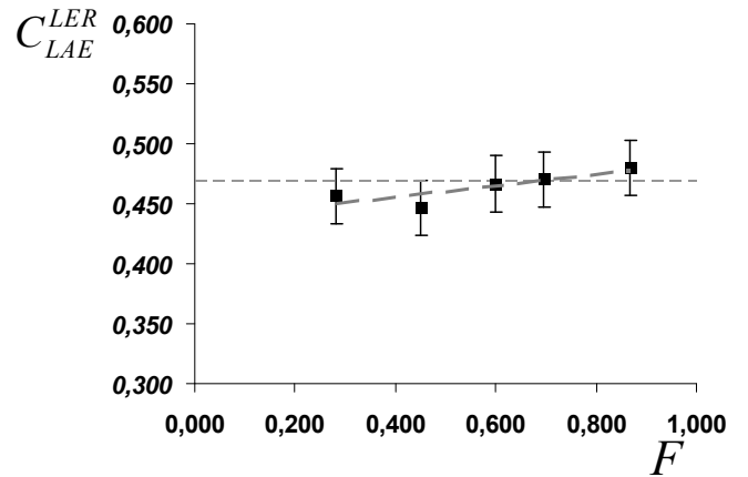
Fig. Annexe XXI-5B : Graphique corrigé présentant le résultat de la lixiviation (N°1) de l'enrobé ER_{160,240}^{45} qui se caractérise par une pente a = 0,05 \pm 0,05
