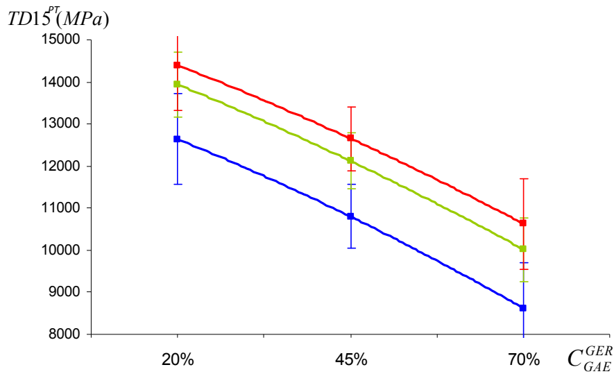
Fig. IV-9 : module en traction directe à 15°C post traité en fonction du pourcentage de recyclage pour une durée de malaxage de 40 s (110°C en bleu, 135°C en vert, 160°C en rouge)
