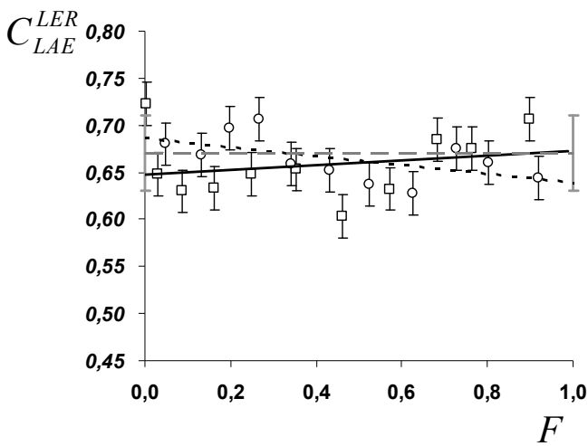
Fig. III-11 : influence de la durée de malaxage sur des enrobés recyclés fabriqués à 160°C de granulométrie 0/14 mm (échantillons ER_{160,40}^{0/14} et ER_{160,240}^{0/14} ) : évolution de la concentration C_{LAE}^{LER} en liant d'agrégat d'enrobé dans le liant lixivié en fonction de la fraction massique F de liant lixivié
