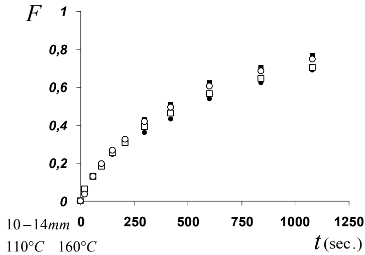
Fig. III-8 : fraction massique F de liant lixivié en fonction du temps de lixiviation Echantillons ER_{110,40}^{10/14} (■), ER_{110,240}^{10/14} (●), ER_{160,40}^{10/14} (□) et ER_{160,240}^{10/14} (○)
