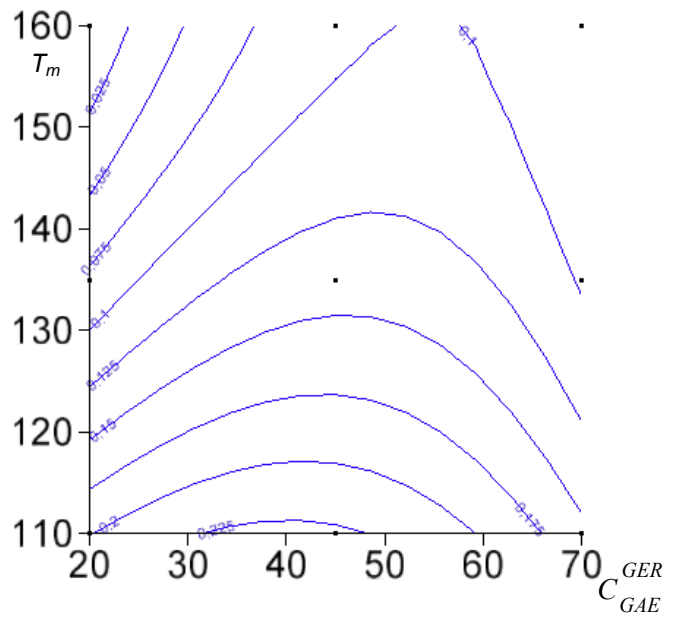
Fig. Annexe XXII-B : pente a des échantillons ER_{T_m, t_m}^{C_{GAE}^{GER}} en fonction de la température T_m et du pourcentage de recyclage C_{GAE}^{GER} , pour une durée de malaxage de 140 s.
