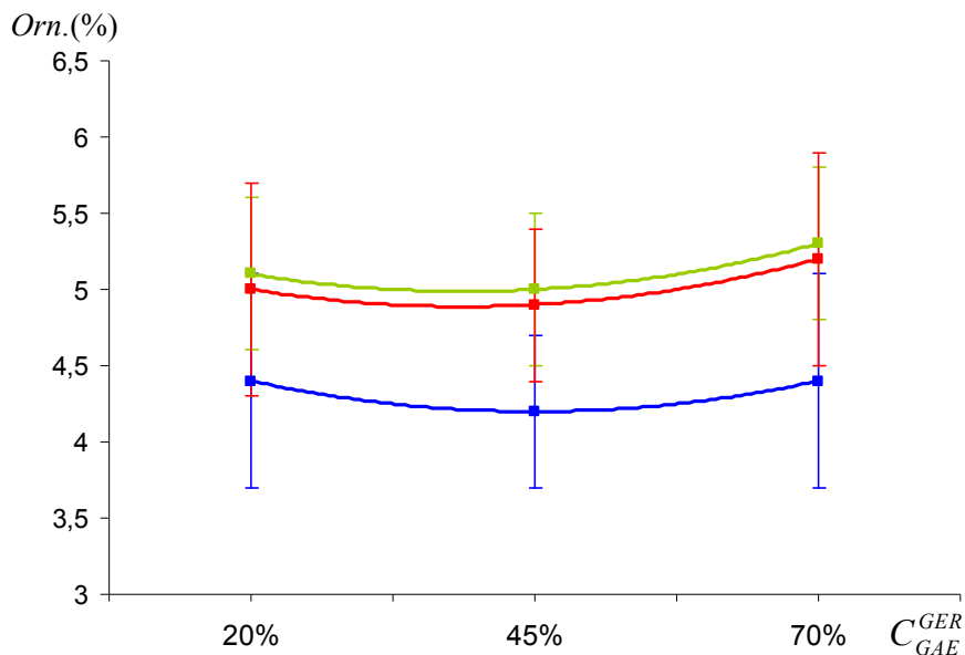
Fig. IV-7 : orniérage en fonction du pourcentage de recyclage pour une durée de malaxage de 40 s (110°C en bleu, 135°C en vert, 160°C en rouge)
