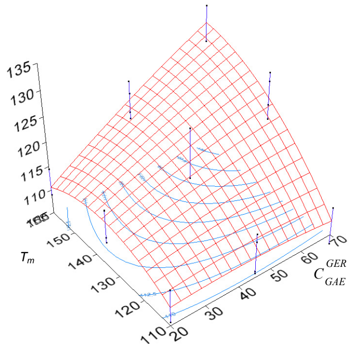
D - fatigue ( \epsilon_6 ) en fonction du pourcentage de recyclage C_{GAE}^{GER} (%) et de T_m la température de malaxage ( ^{\circ}C ) pour une durée de malaxage t_m = 240 s
