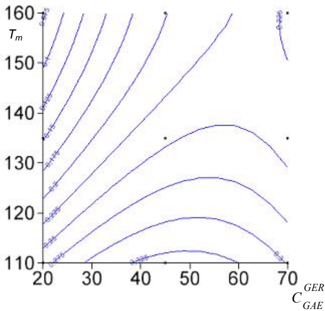
Fig. Annexe XXII-A : pente a des échantillons ER_{T_m, t_m}^{C_{GAE}^{GER}} en fonction de la température T_m et du pourcentage de recyclage C_{GAE}^{GER} , pour une durée de malaxage de 40 s.
