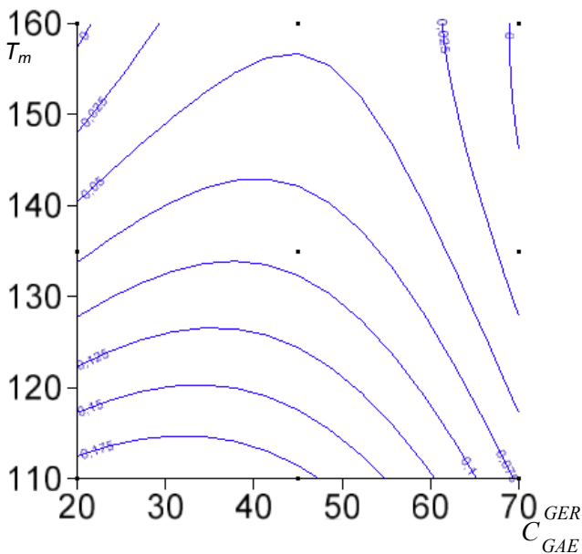
Fig. Annexe XXII-C : pente a des échantillons ER_{T_m, t_m}^{C_{GAE}^{GER}} en fonction de la température T_m et du pourcentage de recyclage C_{GAE}^{GER} , pour une durée de malaxage de 240 s
