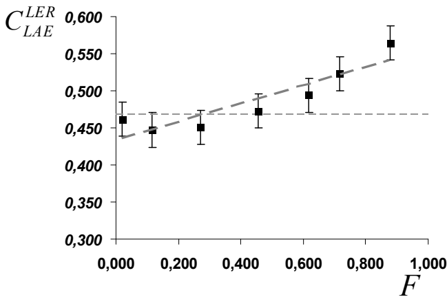
Fig. Annexe XXI-6A : Graphique présentant le résultat de la lixiviation (N°2) de l'enrobé ER_{160,40}^{45} qui se caractérise par une pente a = 0,12 \pm 0,06
