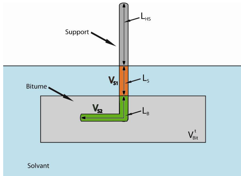
Volumes et longueurs caractérisant le volume immergé de l'échantillon de liant bitumineux
