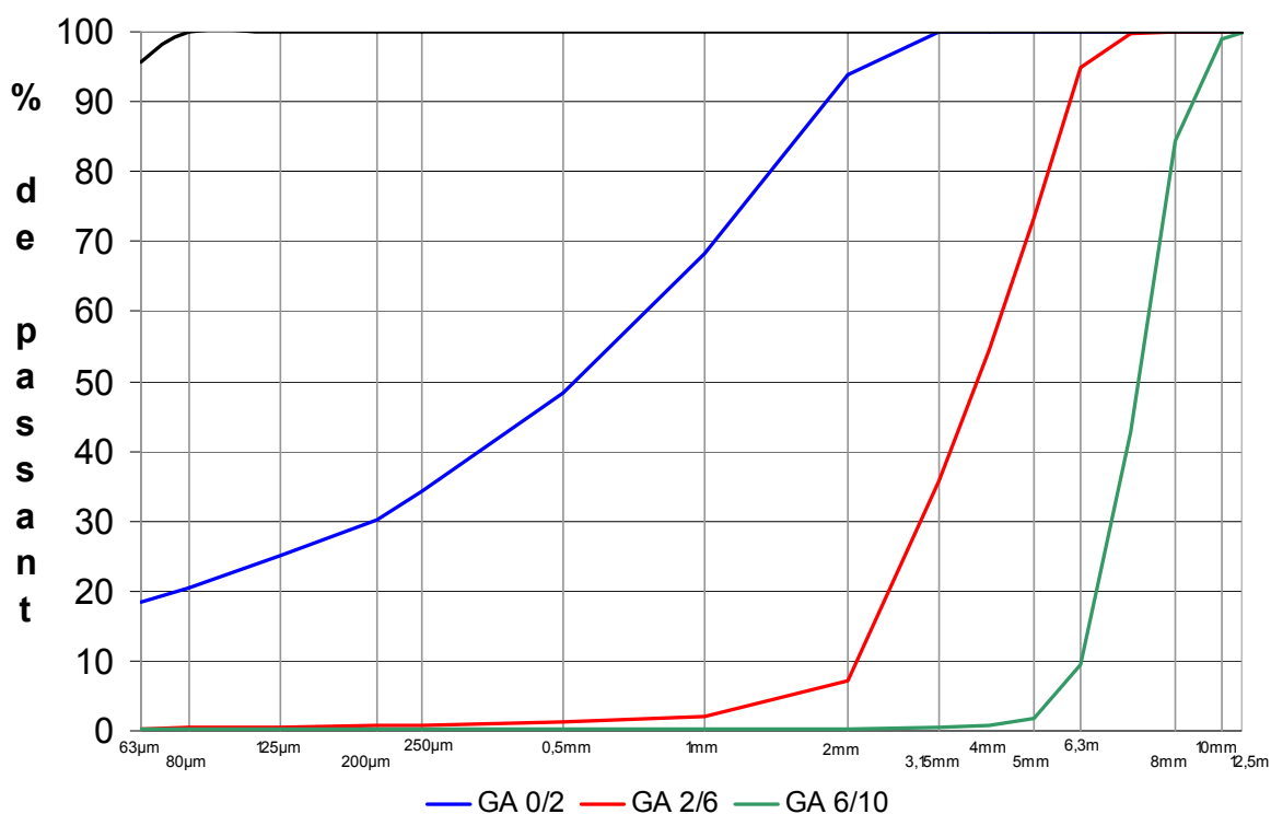
Courbes granulométriques des granulats d'apport GA de fraction 0/2 mm, 2/6 mm et 6/10 mm
