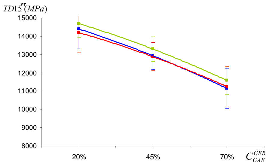
Fig. IV-10 : module en traction directe à 15°C post traité en fonction du pourcentage de recyclage pour une durée de malaxage de 240 s (110°C en bleu, 135°C en vert, 160°C en rouge)
