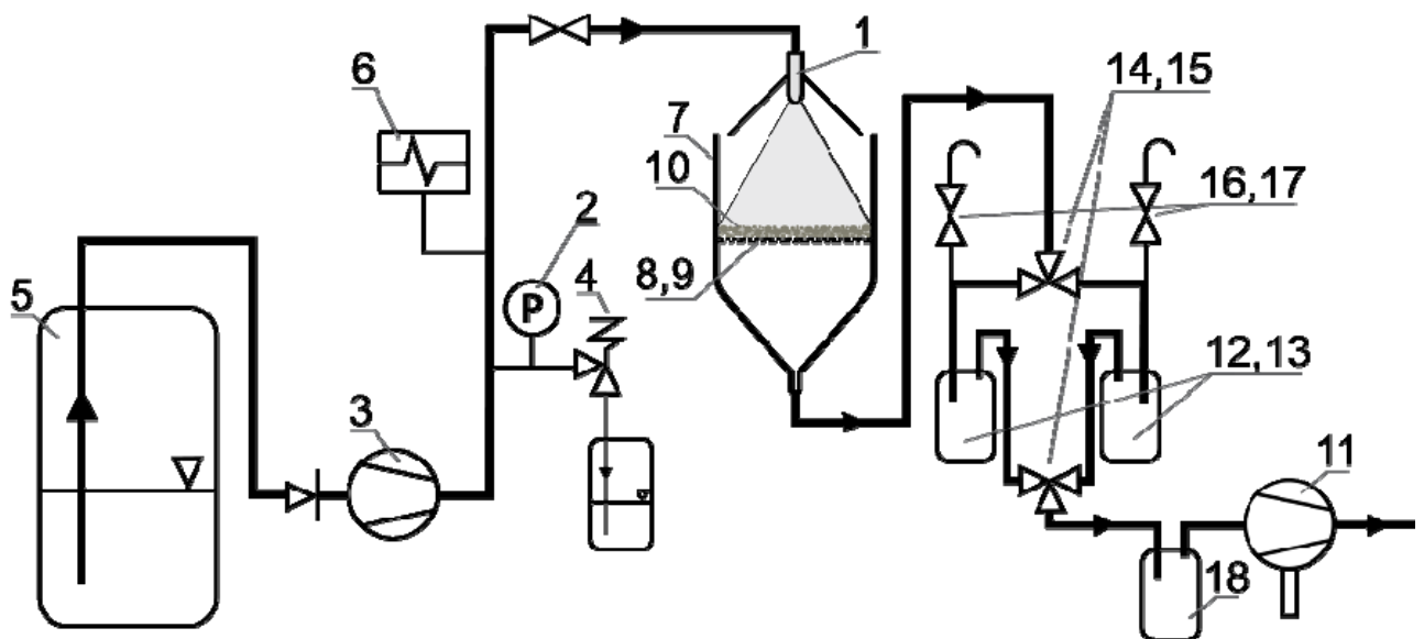
Fig. III-1 : schéma du dispositif expérimental d'extraction par lixiviation.
