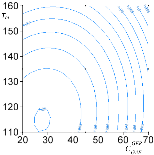
C - Courbes de niveau du rapport des modules en traction directe à 10°C et 15°C (MPa) en fonction du pourcentage de recyclage C_{GAE}^{GER} (%) et de T_m la température de malaxage (°C) pour une durée de malaxage t_m = 240 s
