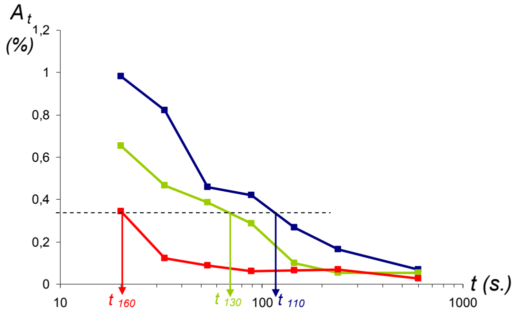
Fig. II-7 : cinétique de la disparition des amas d'agrégats d'enrobé en fonction de la durée du malaxage et de la température de la fabrication (110°C en bleu, 130°C en vert et 160°C en rouge)
