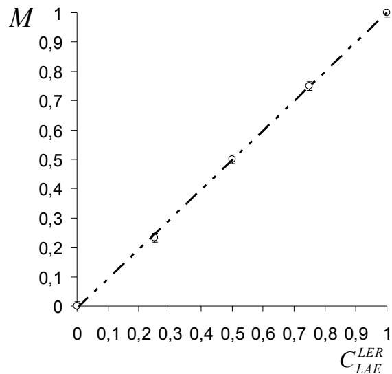
Figure B : Validation de la mesure M à l'aide de 5 solutions étalons d'une concentration en LER de 0,008 et de concentrations C_{LAE}^{LER} = (0 ; 0,23 ; 0,5 ; 0,75 ; 1)
