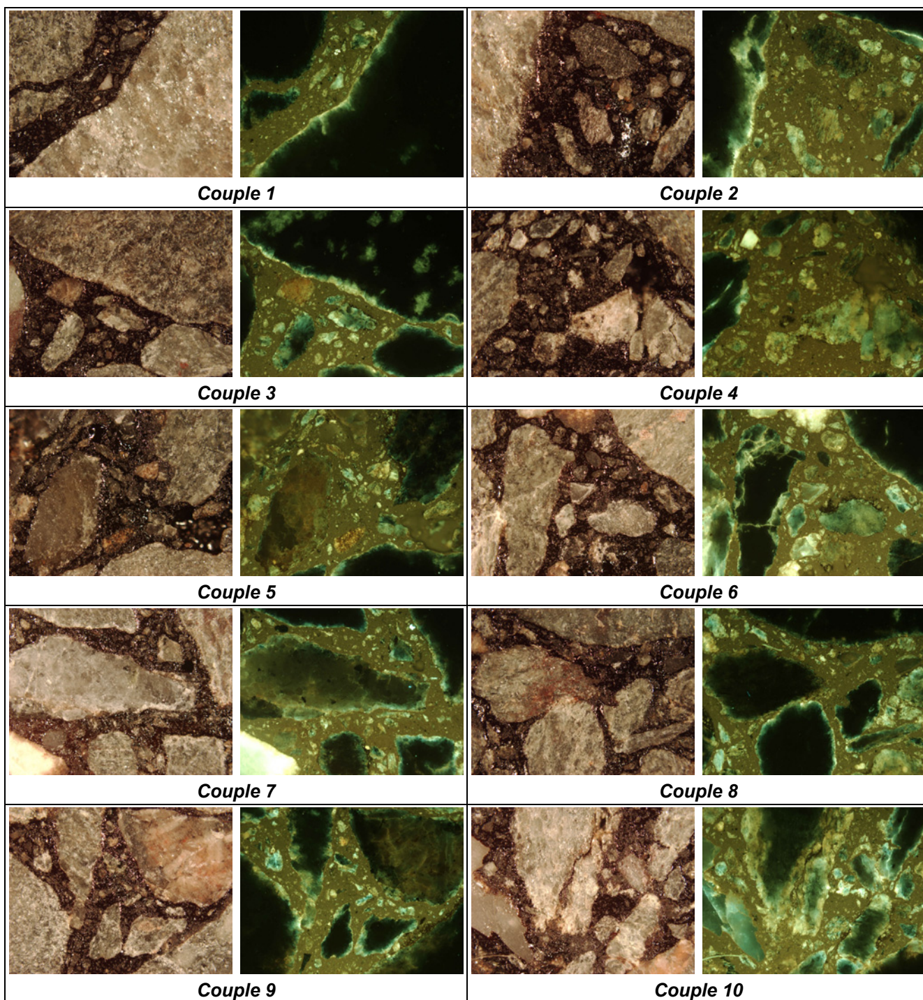
Couples de photographies sous éclairage naturel et UV caractérisant le prélèvement après 4 min de malaxage à 130°C – échantillon 6, (échelle de prise de vue 4.6*3.5 mm)
