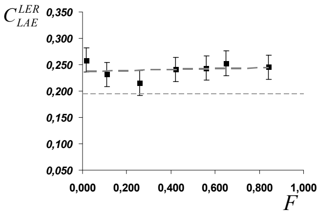
Fig. Annexe XXI-2A : Graphique présentant le résultat de la lixiviation (N°8) de l'enrobé ER_{135,240}^{20} qui se caractérise par une pente a = 0,01 \pm 0,05
