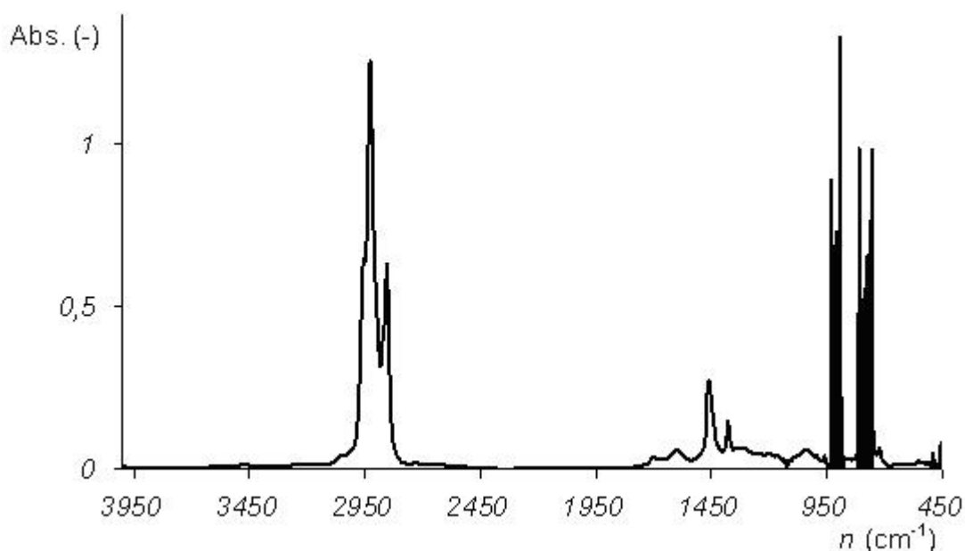
Fig. III-4 : spectre infrarouge d'un liant d'agrégats d'enrobé de concentration égale à 0,008
