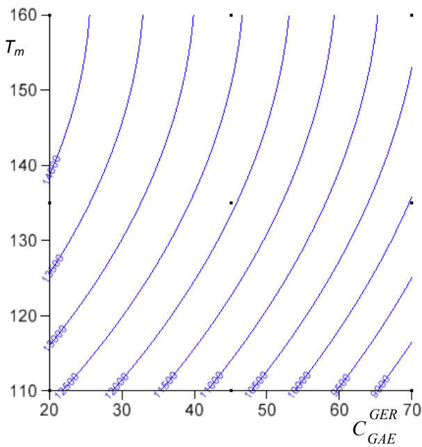
A - Courbes de niveau du module TD15°C (MPa) en fonction du pourcentage de recyclage C_{GAE}^{GER} (%) et de T_m la température de malaxage (°C) pour une durée de malaxage t_m = 40 s
