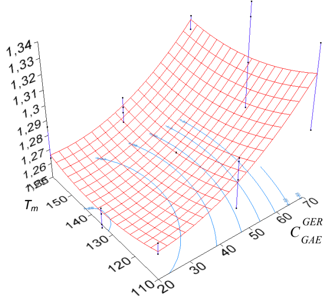
D - Rapport des modules en traction directe à 10°C et 15°C (MPa) en fonction du pourcentage de recyclage C_{GAE}^{GER} (%) et de T_m la température de malaxage (°C) pour une durée de malaxage t_m = 140 s
