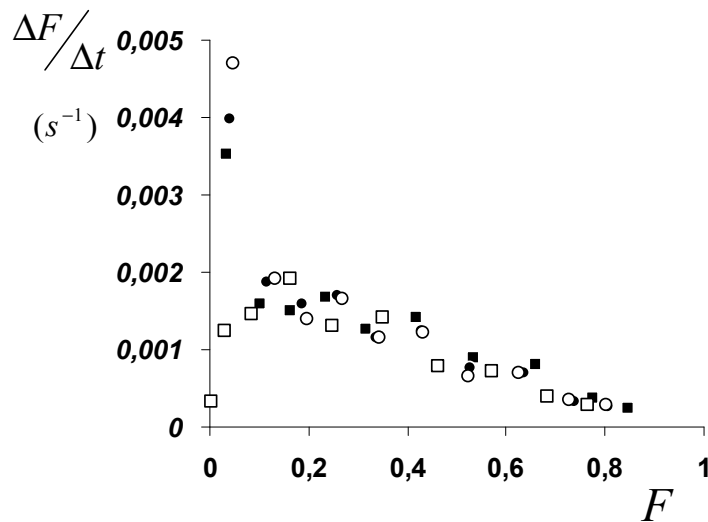
Fig. III-9 : vitesse d'extraction \Delta F/\Delta t en fonction de la fraction massique F de liant lixivié Echantillons ER_{110,40}^{0/14} (■), ER_{110,240}^{0/14} (●), ER_{160,40}^{0/14} (□) et ER_{160,240}^{0/14} (○)
