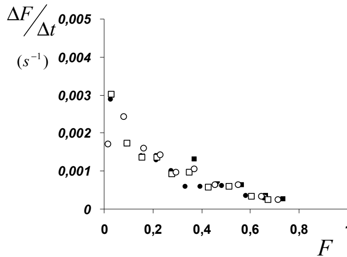
Fig. III-10 : vitesse d'extraction \Delta F/\Delta t en fonction de la fraction massique F de liant lixivié Echantillons ER_{110,40}^{10/14} (■), ER_{110,240}^{10/14} (●), ER_{160,40}^{10/14} (□) et ER_{160,240}^{10/14} (○)
