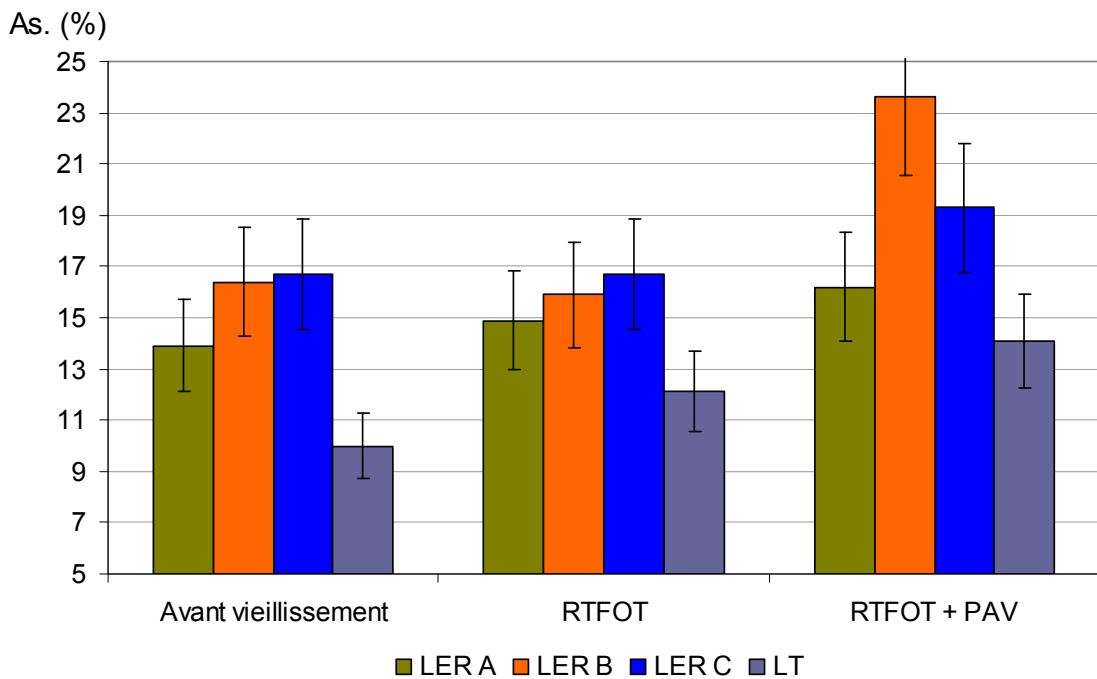
Teneur en asphaltènes des liants d'enrobé recyclé A, B, C et du liant témoin LT, en fonction des étapes de vieillissement
