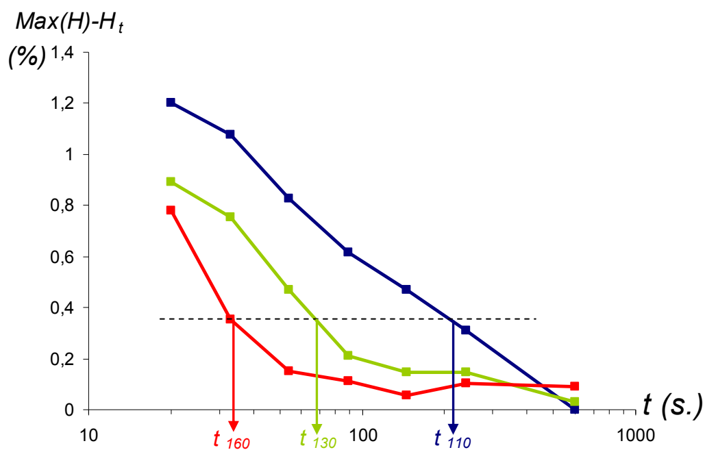
Fig. II-8 : cinétique de l'homogénéisation du liant de l'enrobé recyclé en fonction de la durée du malaxage et de la température de la fabrication (110°C en bleu, 130°C en orange et 160°C en rouge)
