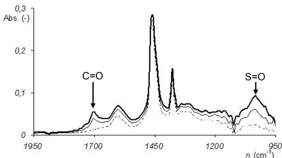
Fig. III-5 : spectres IR de solutions de bitumes modèles de concentration 0,008 g/g Solution de LA en trait pointillé, solution de LAE en trait gras, solution de LA + LAE en trait fin
