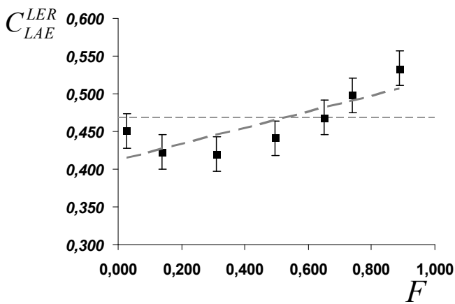
Fig. Annexe XXI-9A : Graphique présentant le résultat de la lixiviation (N°7) de l'enrobé ER_{110,240}^{45} qui se caractérise par une pente a = 0,11 \pm 0,06
