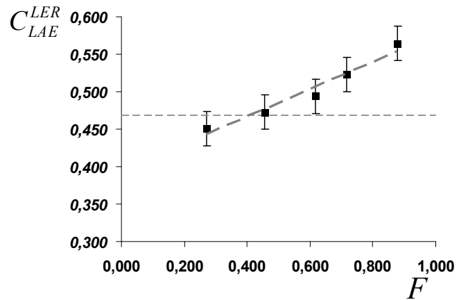
Fig. Annexe XXI-6B : Graphique corrigé présentant le résultat de la lixiviation (N°2) de l'enrobé ER_{160,40}^{45} qui se caractérise par une pente a = 0,18 \pm 0,07
