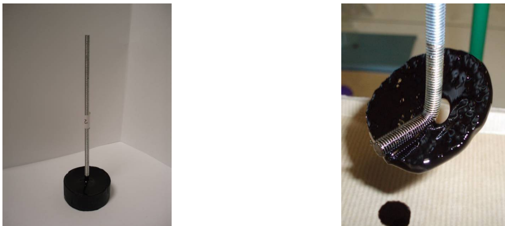
Figure 3 - Présentation des échantillons de bitumes avant l'essai (gauche) et dans le cas d'un échantillon ayant perdu environ 80% de sa masse (droite)
