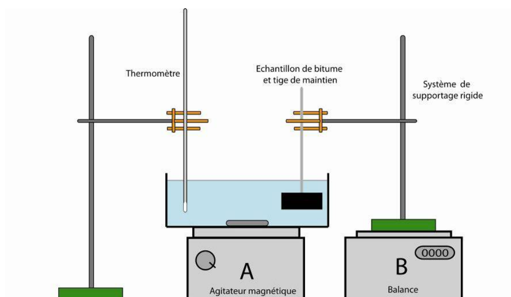
Figure 1 - Dispositif expérimental permettant la mesure du coefficient de solvation d'un échantillon de bitume dans du tétrachloroéthylène par l'exploitation de la poussée d'Archimède
