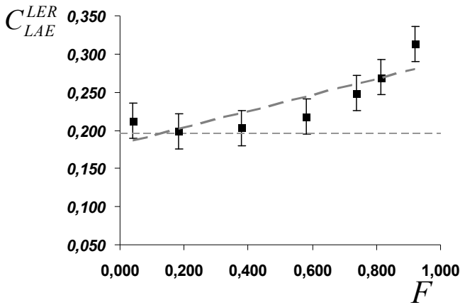
Fig. Annexe XXI-1A : Graphique présentant le résultat de la lixiviation (N°4) de l'enrobé ER_{110,140}^{20} qui se caractérise par une pente a = 0,11 \pm 0,06
