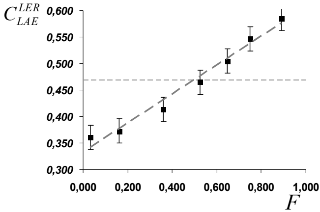
Fig. Annexe XXI-8A : Graphique présentant le résultat de la lixiviation (N°6) de l'enrobé ER_{110,40}^{45} qui se caractérise par une pente a = 0,27 \pm 0,07
