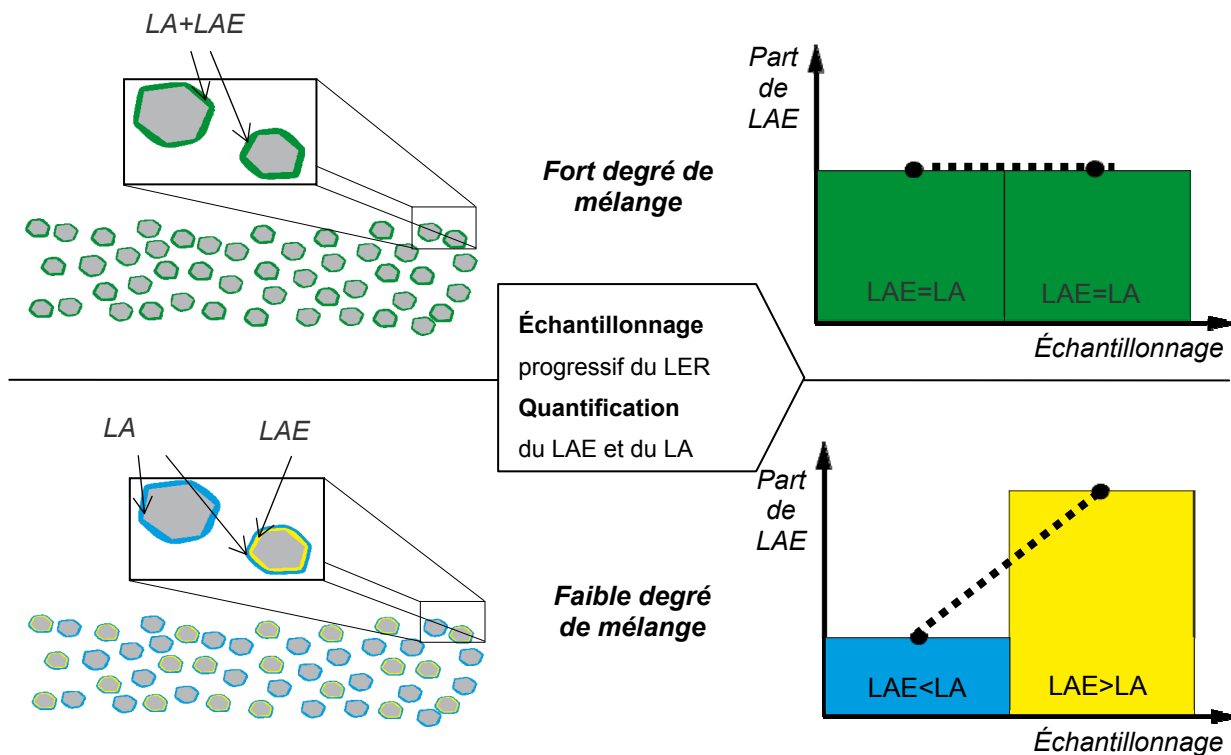
Fig. I-24 : caractérisation du degré de mélange des liants dans le cas d'un enrobé recyclé composé d'une part identique de liant d'agrégats d'enrobé et de liant d'apport
