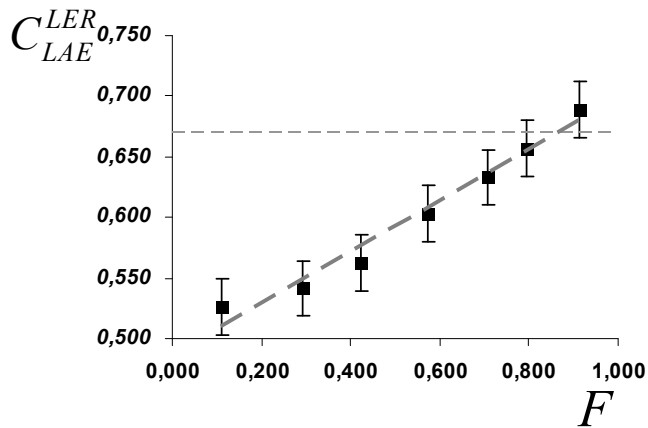
Fig. Annexe XXI-10A : Graphique présentant le résultat de la lixiviation (N°3) de l'enrobé ER_{110,140}^{70} qui se caractérise par une pente a = 0,13 \pm 0,06
