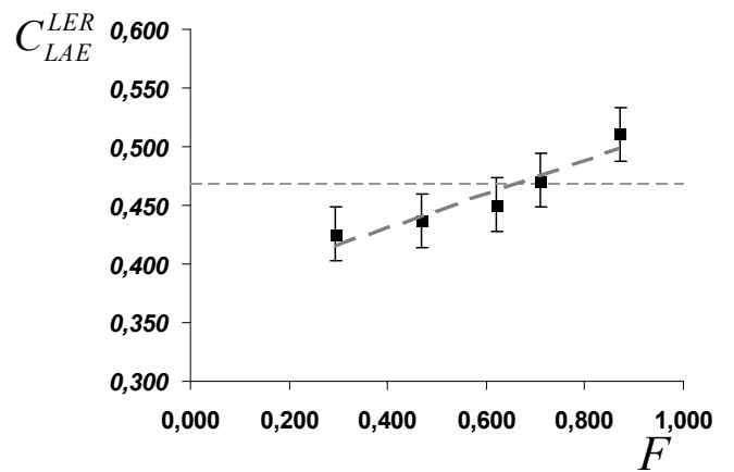
Fig. Annexe XXI-7B : Graphique corrigé présentant le résultat de la lixiviation (N°5) de l'enrobé ER_{135,140}^{45} qui se caractérise par une pente a = 0,14 \pm 0,07
