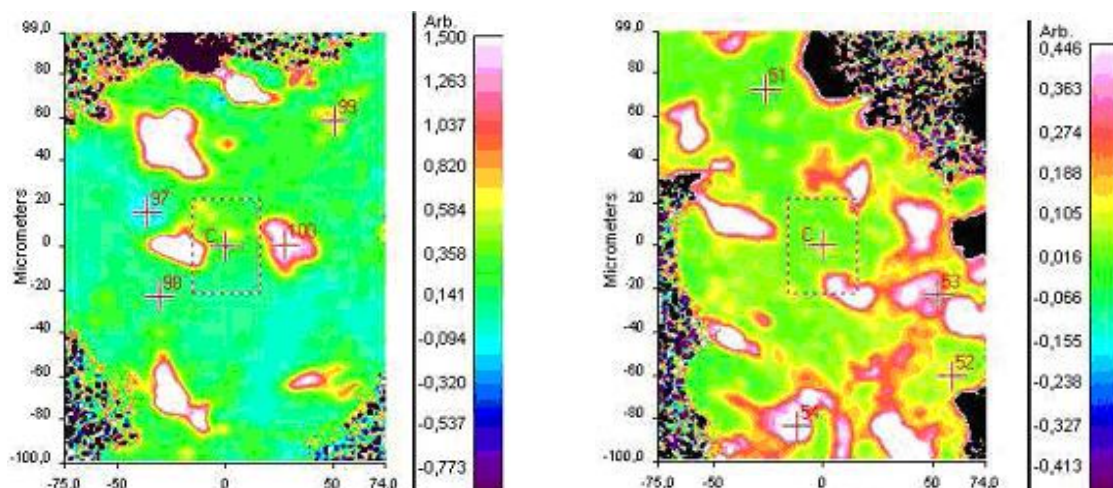
Fig. I-20 : cartographie des amas d'agrégats d'enrobé (en blanc) au sein d'un enrobé recyclé dans le cas de l'utilisation d'un agrégat vieilli artificiellement durant 4 jours (à gauche) et durant 8 jours (à droite) (El Beze 2008)
