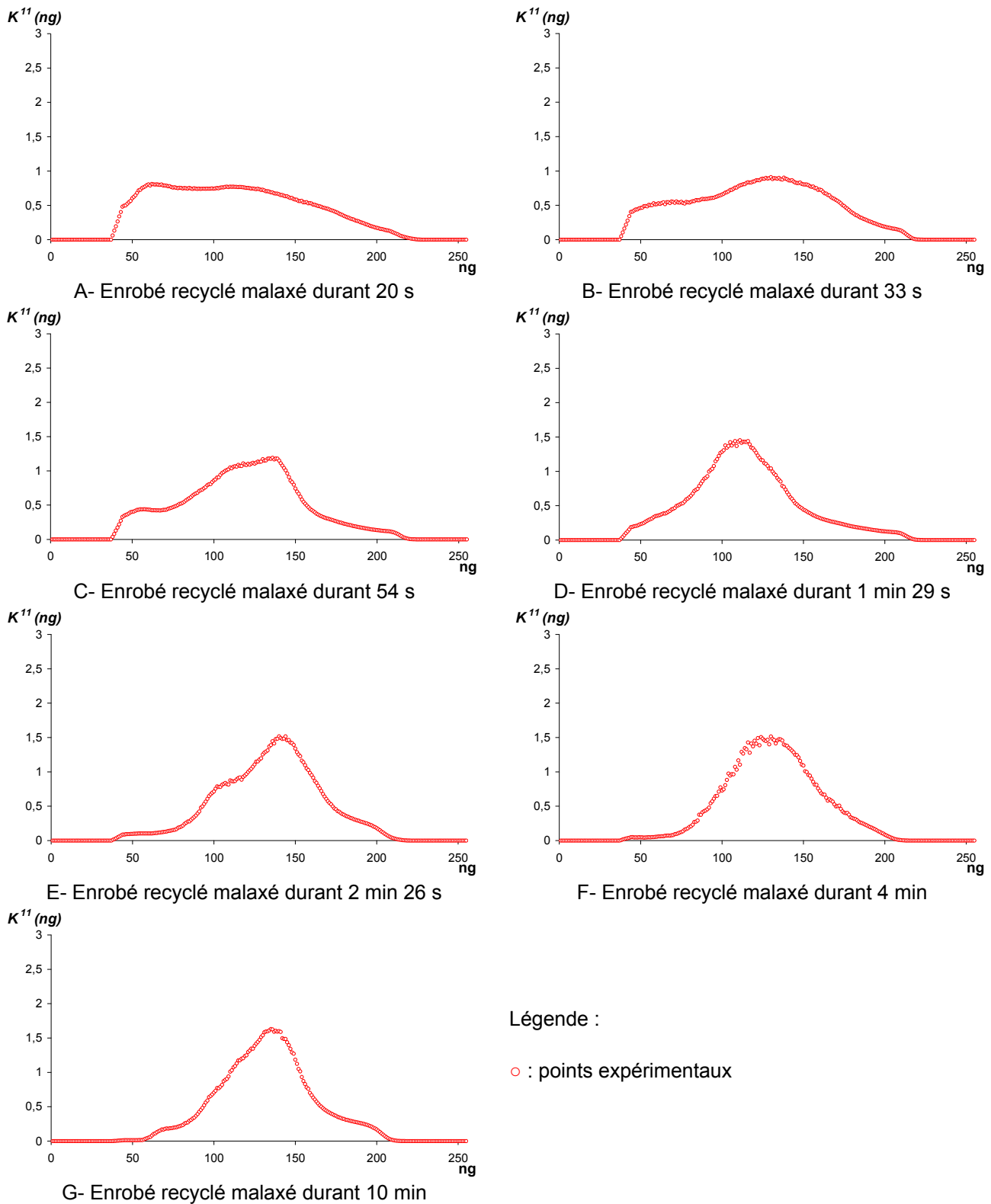
Fig. II-6 : présentation des chromatogrammes moyens obtenus par l'étude d'enrobé recyclé caractérisé à chaque prélèvement par 11 couples de photographies LB/UV, fabriqués à 130°C et pour un taux de recyclage égal à 70 % conditionnant une teneur en liant d'apport de 1,8 %
