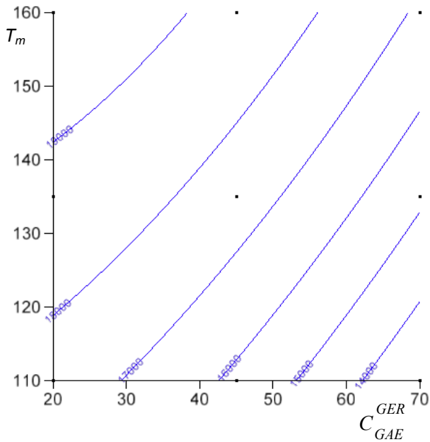
A - Courbes de niveau du module flexion 2 points à 10°C (MPa) en fonction du pourcentage de recyclage C_{GAE}^{GER} (%) et de T_m la température de malaxage (°C) pour une durée de malaxage t_m = 40 s
