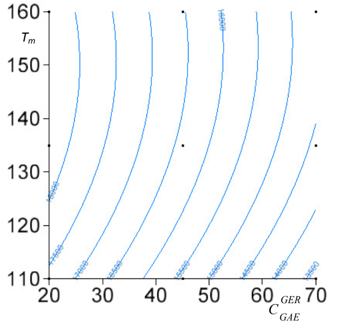
B - Courbes de niveau du module TD10°C (MPa) en fonction du pourcentage de recyclage C_{GAE}^{GER} (%) et de T_m la température de malaxage (°C) pour une durée de malaxage t_m = 140 s
