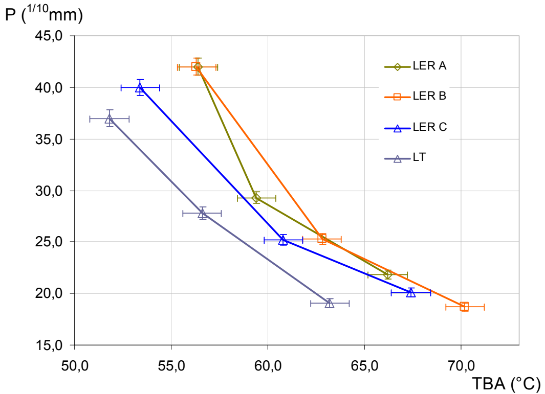
Figure comparant l'évolution des caractéristiques des liants d'enrobé recyclé lors de la réalisation des essais RTFOT et PAV, avec un liant 35/50 témoin
