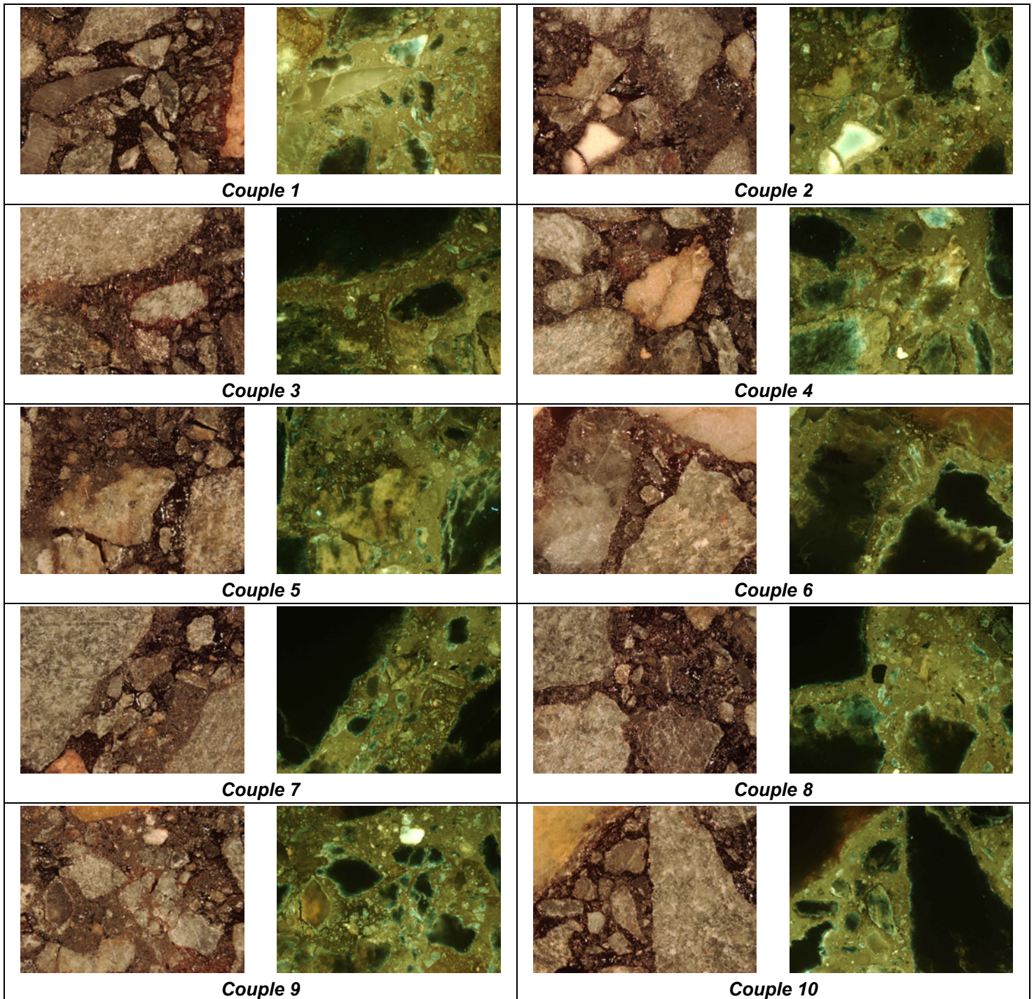
Couples de photographies sous éclairage naturel et UV caractérisant le prélèvement après 20 s de malaxage à 160°C – échantillon 1, (échelle de prise de vue 4.6*3.5 mm)
