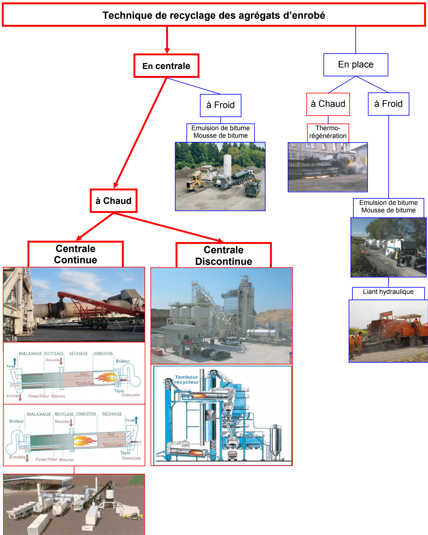
Fig. I-10 : présentation des possibilités techniques de recyclage des chaussées bitumineuses Images empruntées (Serfass 2008)
