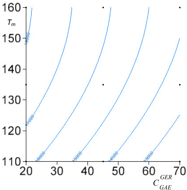
A - Courbes de niveau du module TD10°C (MPa) en fonction du pourcentage de recyclage C_{GAE}^{GER} (%) et de T_m la température de malaxage (°C) pour une durée de malaxage t_m = 40 s
