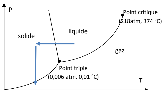
Figure IV-18. Diagramme de phase de l'eau. Les flèches bleues représentent les étapes d'un séchage par cryodessication.
