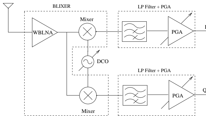
Figure 1: L'architecture du frontal radio pour les applications multistandards de communication sans fils : illustration [5].
