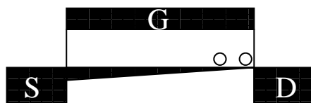
Figure 2: Phénomène HCI: illustration.
