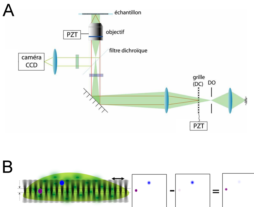
FIGURE 4.2 – (A) Schéma du microscope à illumination structurée utilisé (DO : Diaphragme d'Ouverture, DC : Diaphragme de Champ). (B) Image de la grille dans l'échantillon : l'image de la grille n'est nette que dans le plan de mise au point. et ne modulera donc le signal que des objets qui s'y trouvent. Les objets se trouvant hors du plan de mise au point ne seront pas modulés et pourront être supprimés lors de la reconstruction.
