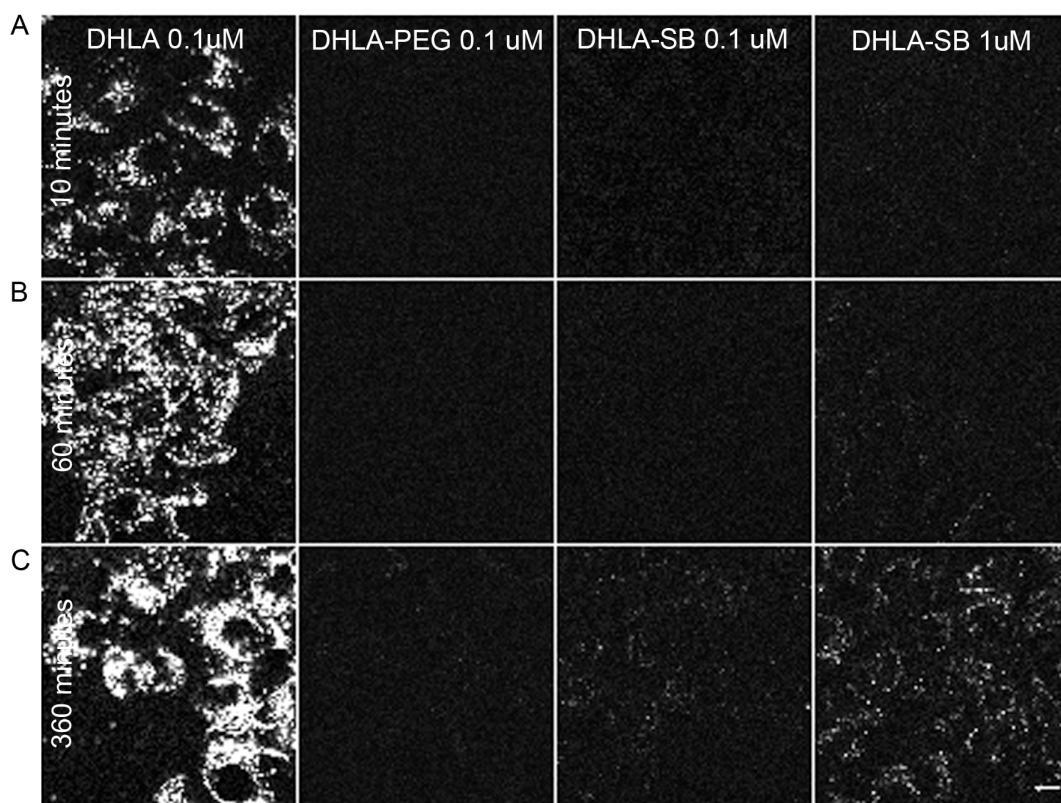
FIGURE 1.7 – Adsorption non spécifique des QDs (CdSe/CdS/ZnS) DHLA, DHLA-PEG 750 et DHLA-SB avec différents temps d'incubation : 10 minutes (A), 60 minutes (B) et 360 minutes (C). Les images ont été acquises dans des conditions identiques et sont représentées avec le même contraste. La barre d'échelle vaut 10 \mu\text{m} .
