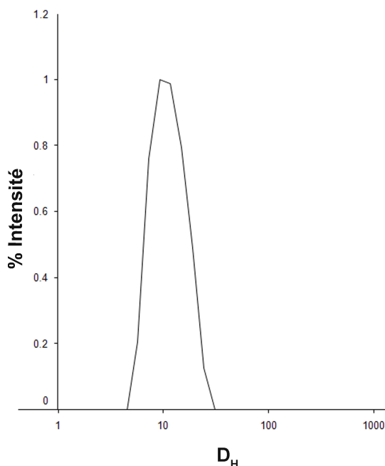
FIGURE 1.5 – Mesure du diamètre hydrodynamique des QDs DHLA-SB par Diffusion Dynamique de la Lumière. Les QDs CdSe/ZnS ici analysés présentent un diamètre au TEM de 4,5 nm.
