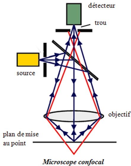
FIGURE 4.1 – Schéma du microscope confocal.
