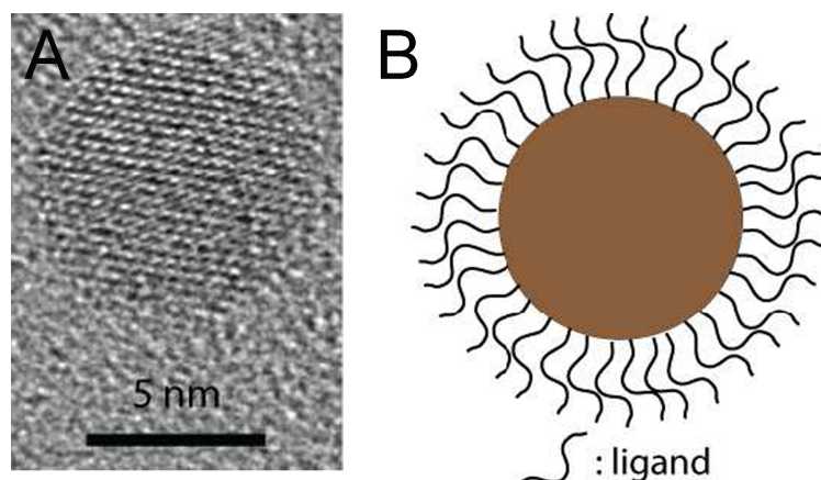
FIGURE 1 – Image de microscopie électronique à transmission (TEM) à haute résolution d'un nanocristal de semiconducteur (A). Schéma d'un quantum dot avec ses ligands de fin de synthèse (B).
