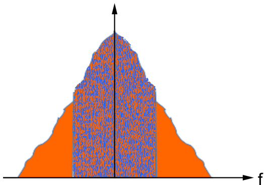
FIGURE 4.5 – Spectre schématique de l’image uniformément éclairée, où les fréquences provenant du plan de mise au point ( I_{if} dans l’équation 4.1) sont représentées en orange et les fréquences provenant des plans hors du plan de mise au point ( I_{of} dans l’équation 4.1) sont représentées en bleu.
