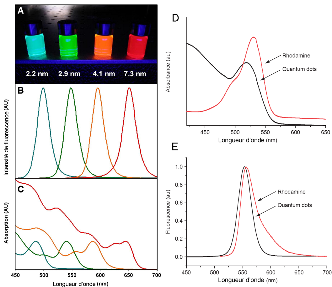
FIGURE 4 – Spectres d’absorbance (C et D) et d’émission de fluorescence (B et E) de Quantum Dots de même composition chimique et de tailles croissantes (A, B, C) et de Quantum Dots comparés à la Rhodamine. Les images A, B et C proviennent de la référence [24] et les images D et E de la référence [25].
