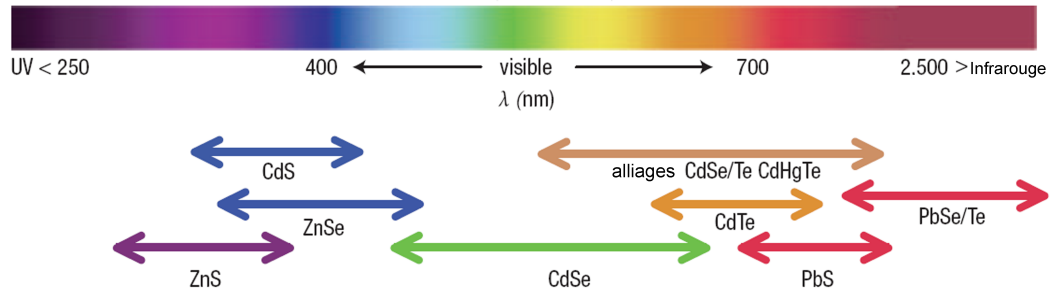
FIGURE 2 – Matériaux disponibles pour la synthèse de Quantum Dots et permettant d’obtenir des sondes dans l’ensemble des spectres visible et infrarouge. [7]
