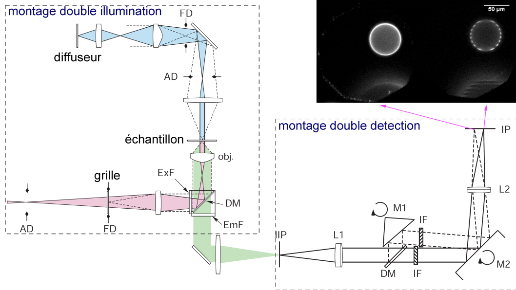
FIGURE 4.8 – Schéma du montage optique. La partie 'double illumination' utilise un statif de microscope commercial Olympus IX-71 et exploite à la fois les chemins d'épi-illumination et d'illumination en transmission. La partie 'double détection' est conçue pour séparer spectralement les deux images et les conjuguer sur la même caméra CCD. AD : diaphragme d'ouverture, FD : diaphragme de champ, obj. : objectif de microscope, ExF : filtre d'excitation, EmF : filtre d'émission, DM : miroir dichroïque, IIP : 'image intermédiaire, L1 et L2 : lentilles achromatiques, M1 and M2 : miroirs , IF : filtres interférentiels, IP : image sur la caméra.
