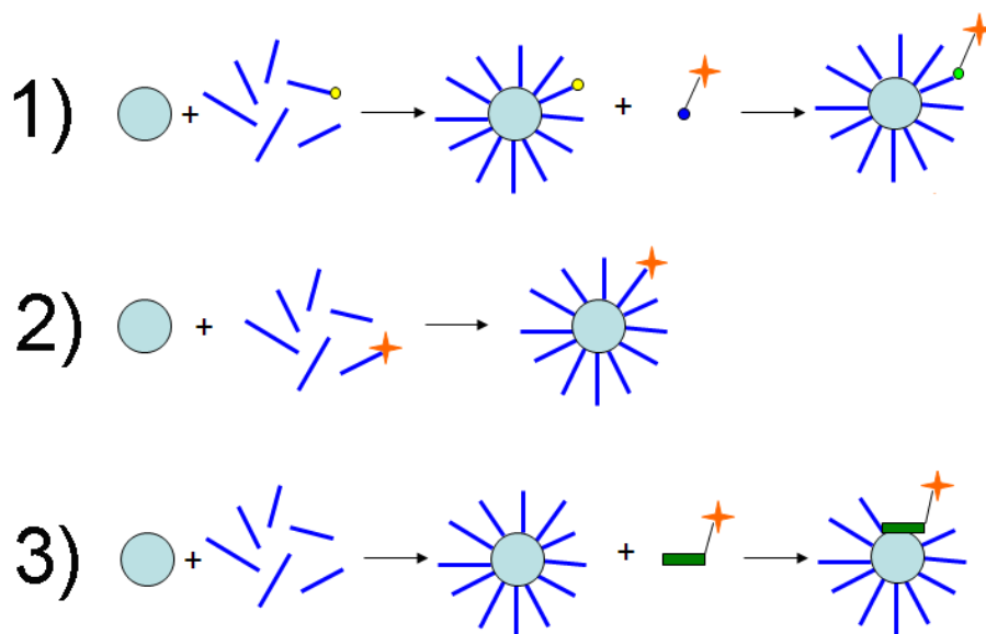
FIGURE 3.1 – Schéma des stratégies de fonctionnalisation des QDs. 1) Le QD est solubilisé à l’aide de molécules dont certaines présentent un groupe réactif, que l’on fera ensuite réagir avec la molécule de ciblage ; 2) le QD est solubilisé directement à l’aide de molécules dont certaines présentent une fonction de ciblage ; 3) le QD est solubilisé puis mélangé avec des molécules de ciblage contenant un groupe affín pour sa surface inorganique (par exemple le His TAG).
