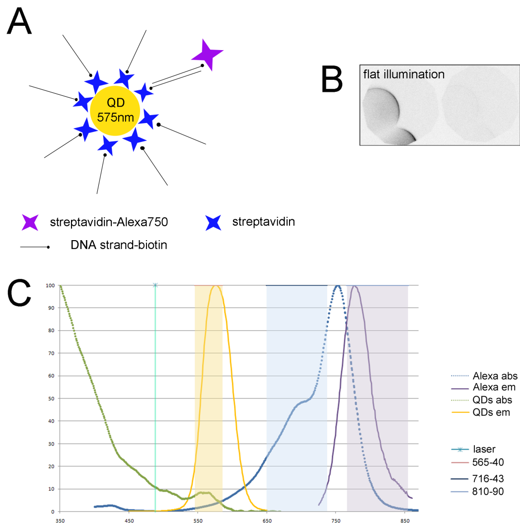
FIGURE 4.9 – Schéma de la sonde bi-couleur (A) ; absence de FRET grâce à l'espaceur d'ADN quand on éclaire seulement le donneur, soit les QDs (illumination uniforme) (B) ; spectres d'absorption et d'émission des deux fluorophores choisis (C).
