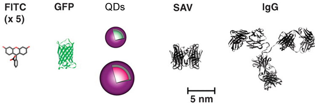
FIGURE 3 – Comparaison de la taille d’un QD (CdSe/ZnS vert = 4nm et rouge = 6,5 nm de diamètre) à celle d’autres fluorophores (isothiocyanate de la fluorescéine (FITC), Green Fluorescent Protein, (GFP)) et de protéines pour le ciblage (streptavidine (SAV) et anticorps (IgG)). [8]
