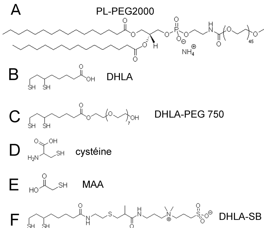
FIGURE 1.2 – Formules chimiques de certains des ligands présentés dans le texte : le phospholipide – PEG pour l'encapsulation en micelles (A), le DHLA (B), le DHLA-PEG750 (C), la Cystéine (D) et le DHLA-SB (E) pour l'échange de ligands.
