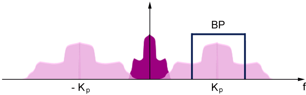
FIGURE 4.7 – Spectre schématique de l’image D (équation 4.3) correspondant à la division de l’image structurée par l’image homogène : l’élément central dans notre cas n’est pas un Dirac comme dans le système de J. Mertz et peut avoir un poids important et ainsi « polluer » les spectres « satellites » centrés autour de K_p et qui nous intéressent.
