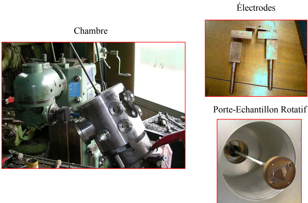
Figure 3.3 : Photos des éléments réalisés pour le montage du bâti d'évaporation thermique.
