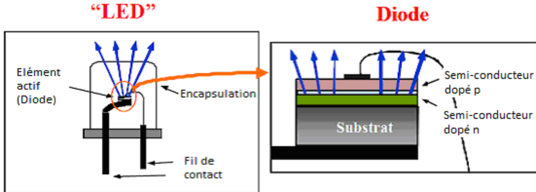
Figure 1.6: Schéma d'une LED.
