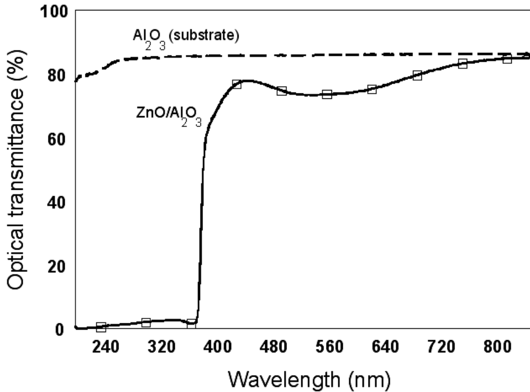
Figure 1.13 : Courbes de transmission à température ambiante d'un substrat Al_2O_3 et d'une couche mince de ZnO type n déposé par PLD sur Al_2O_3 . Après le dépôt de ZnO la transmittance reste quasi constante dans le visible (~80%) puis diminue pour s'annuler à partir de 375 nm [25].
