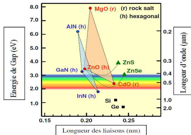
Figure IV.2: Énergie de bande interdite (gap) et longueur d'onde d'émission en fonction de la longueur des liaisons.
