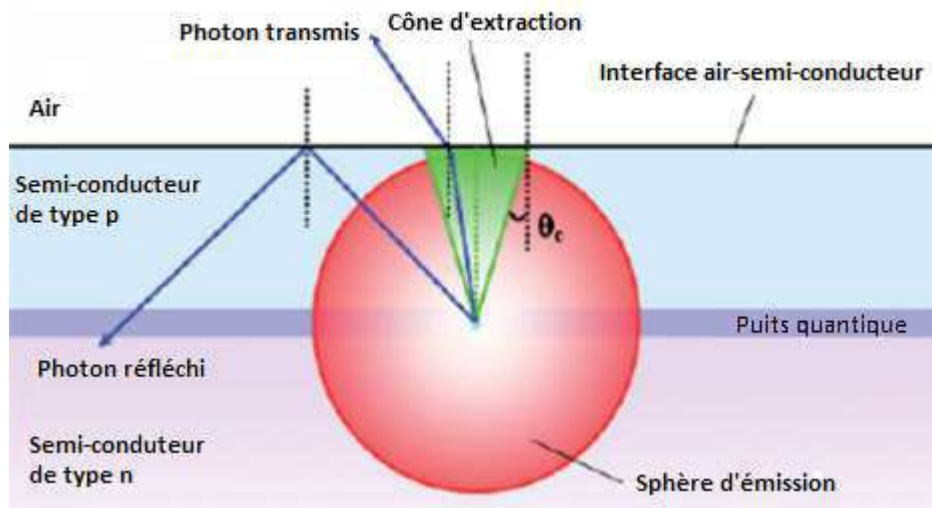
Figure IV.6 Représentation du cône d'extraction (en vert) d'angle solide \theta_c , dans le cas d'une interface air-semi-conducteur. La sphère d'émission des photons est représentée en rouge. [5]
