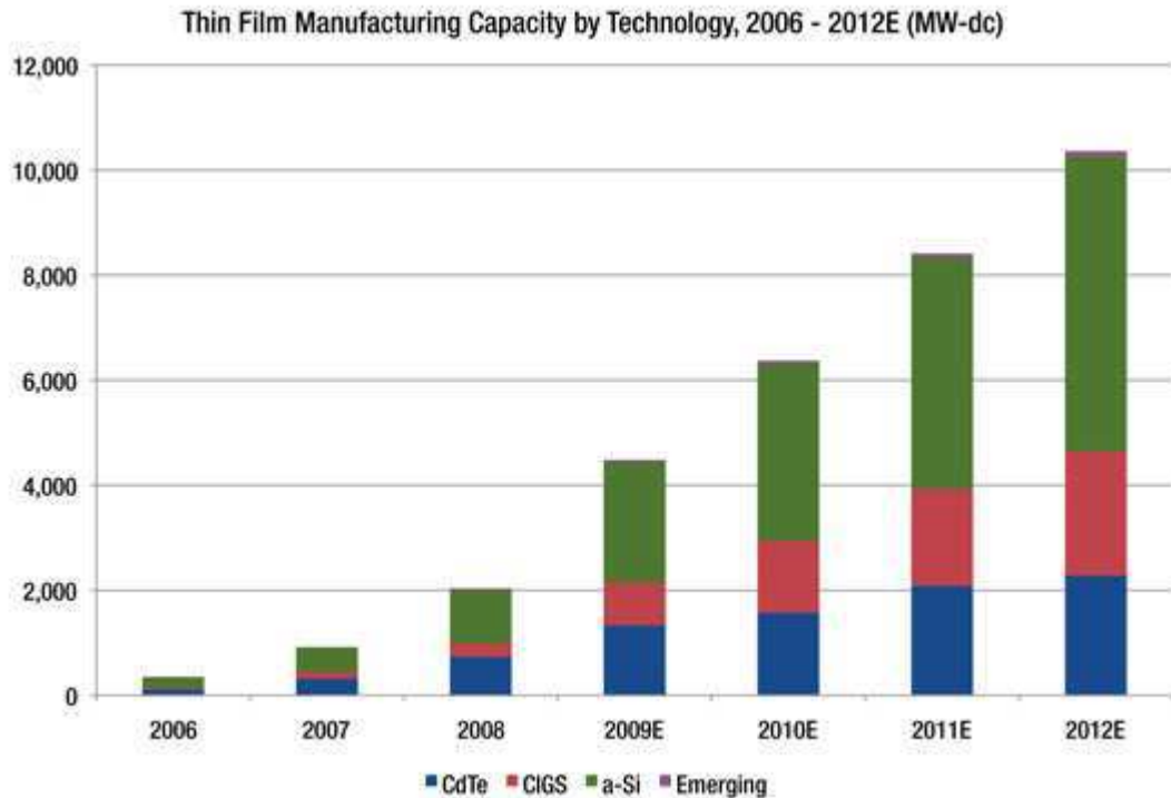
Figure 1.11 : Courbe comparant l'évolution des capacités de production de quatre technologies de PVs en MW en fonction des années. En bleu la technologie CdTe présente une évolution constante comparable à celle basée sur Cu (In,Ga)Se 2 (noté CIGS). Le silicium, représenté en vert, domine nettement le marché et les technologies émergentes en violet sont encore peu représentées. [19]
