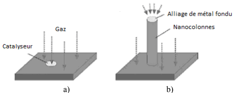
Figure 3.2 : Schéma du principe de mécanisme de croissance par PVT.
