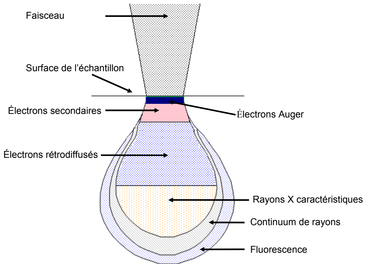
Figure I.3 : Poire d'interaction formée lors de la diffusion des électrons dans un matériau.
