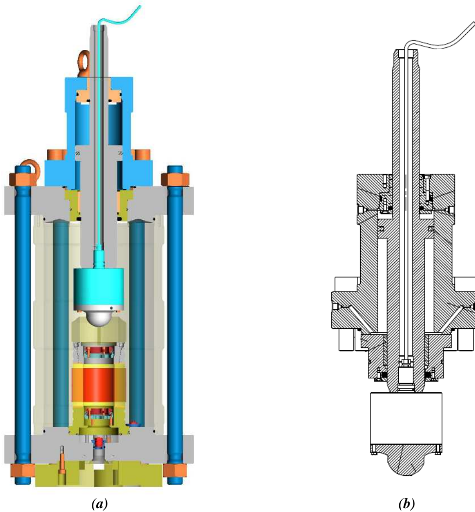
Figure 3-22 : (a) La cellule triaxiale avec le piston piloté par le CPV ; (b) Le détail du piston déviatorique piloté par le CPV.
