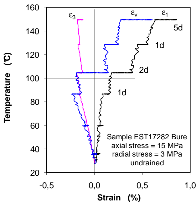
Figure 1-36 : Les déformations radiale, axiale et volumique pendant l'essai de chauffage non-drainé (Zhang, 2010).
