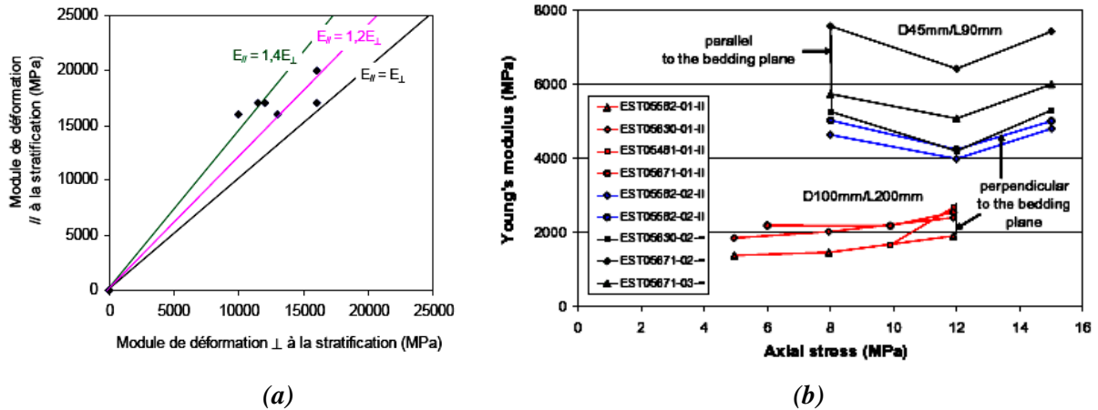
(a) Figure 1-19 : Anisotropie des modules de déformation des argilites, (a) rapport Andra 2005 (Auvray, 2004a, 2004b) ; (b) Zhang et Rothfuchs (2004)
