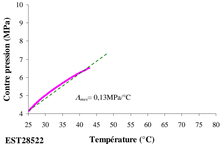
Figure 5-23 : La variation de la contre pression au cours du chauffage non-drainé.
