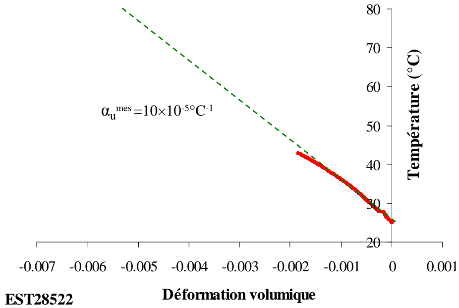
EST2852 Déformation volumique Figure 5-24 : déformation volumique mesurée de l'échantillon EST2852 au cours du chauffage non-drainé.
