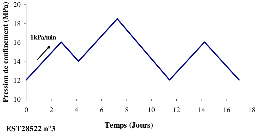
EST28522 n°3 Figure 5-1: Cycle de charge-décharge suivi pour l'essai drainé.
