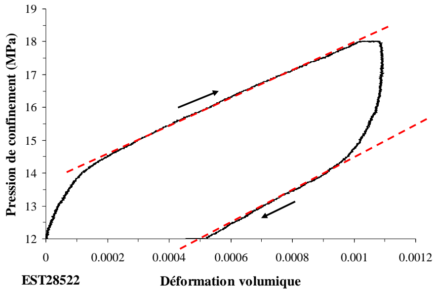
Figure 5-12 : Essai de compression isotrope non-drainé, déformation volumique- pression de confinement.
