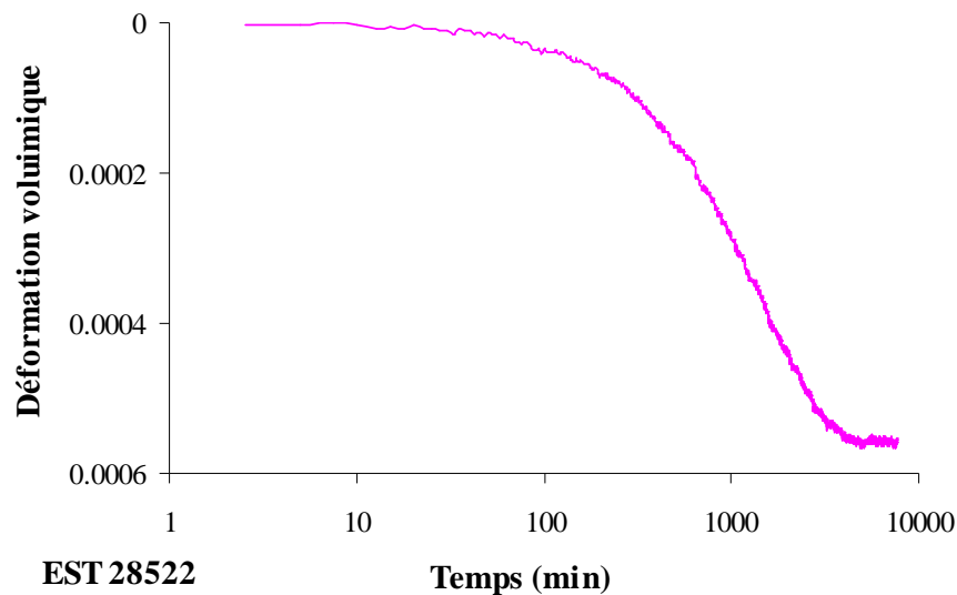
(a) Consolidation sous 13,6 après chargement.
