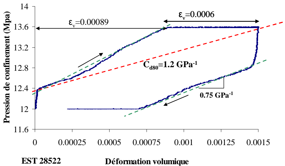
Figure 5-18 : Essai de compression isotrope drainé à 80°C.
