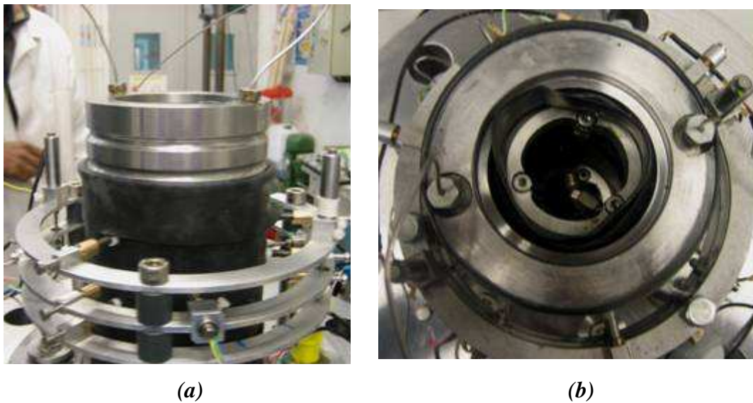
Figure 3-30 : la mise en place de l'embase supérieure et les LVDTs.
