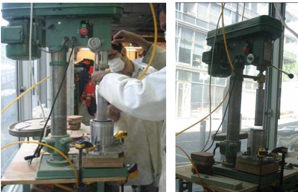
Figure 3-27: Réalisation du cylindre intérieur au carottage diamant.
