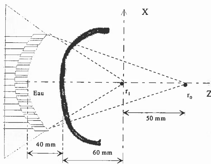
Figure 25. Configuration de l'expérience d'angulation axiale. Le point d'accrochage r_0 se trouve à 150 mm du réseau, le point de focalisation désiré r_l se trouve à 100 mm du réseau.
