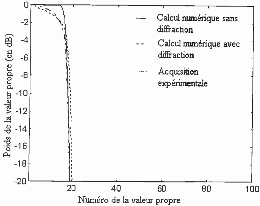
Figure 43. Distribution des valeurs singulières de H calculée numériquement pour la configuration décrite : (a) en ne prenant pas en compte la directivité des transducteurs (ligne solide) et (b) en prenant en compte la directivité des transducteurs (ligne hachurée). Le nombre de degrés de liberté est égal à 17. Il est comparé avec la distribution de valeurs propres trouvée expérimentalement dans la même configuration (ligne pointillée).
