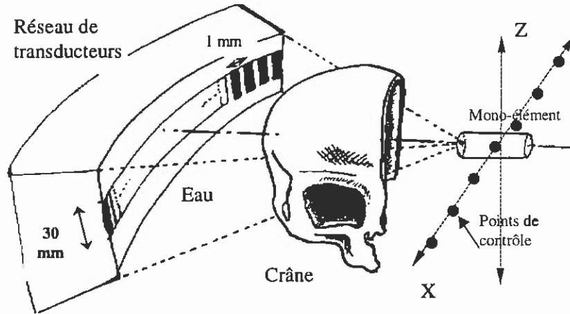
Figure 54. Configuration de la première expérience : L'hydrophone est déplacé le long de l'axe X de point en point lors de l'acquisition de la matrice de propagation H .
