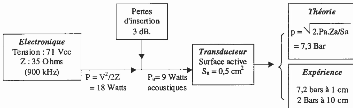
Figure 75. Performances de la chaîne d'émission.
