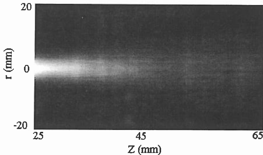
Figure 76. Champ de pression rayonné par un transducteur pour une profondeur variant de 2,5 cm à 6,5 cm et sur une largeur de 4 cm.
