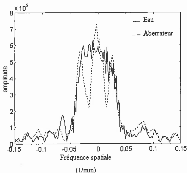
Figure 67. Spectre des fréquences spatiales du champ ultrasonore reçu sur le réseau après propagation dans l'eau (ligne pleine) ou à travers l'aberrateur (ligne pointillée), lorsque le 50 ème point de contrôle agit en tant que source acoustique.
