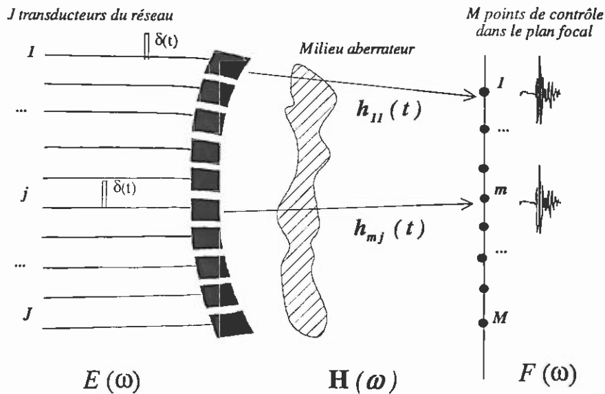
Figure 41. Réponses impulsionnelles transducteur-point de contrôle et opérateur de propagation H .
