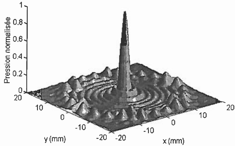
Figure 79. Simulation numérique du faisceau ultrasonore créé par le réseau dans le plan focal z=100 mm.
