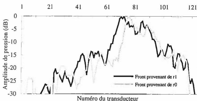
Figure 18. Modulation d'amplitude du front d'onde reçu sur le réseau lorsque la source est située en r_1 comparée à celle du front d'onde calculé à partir du front d'onde provenant de r_0 .
