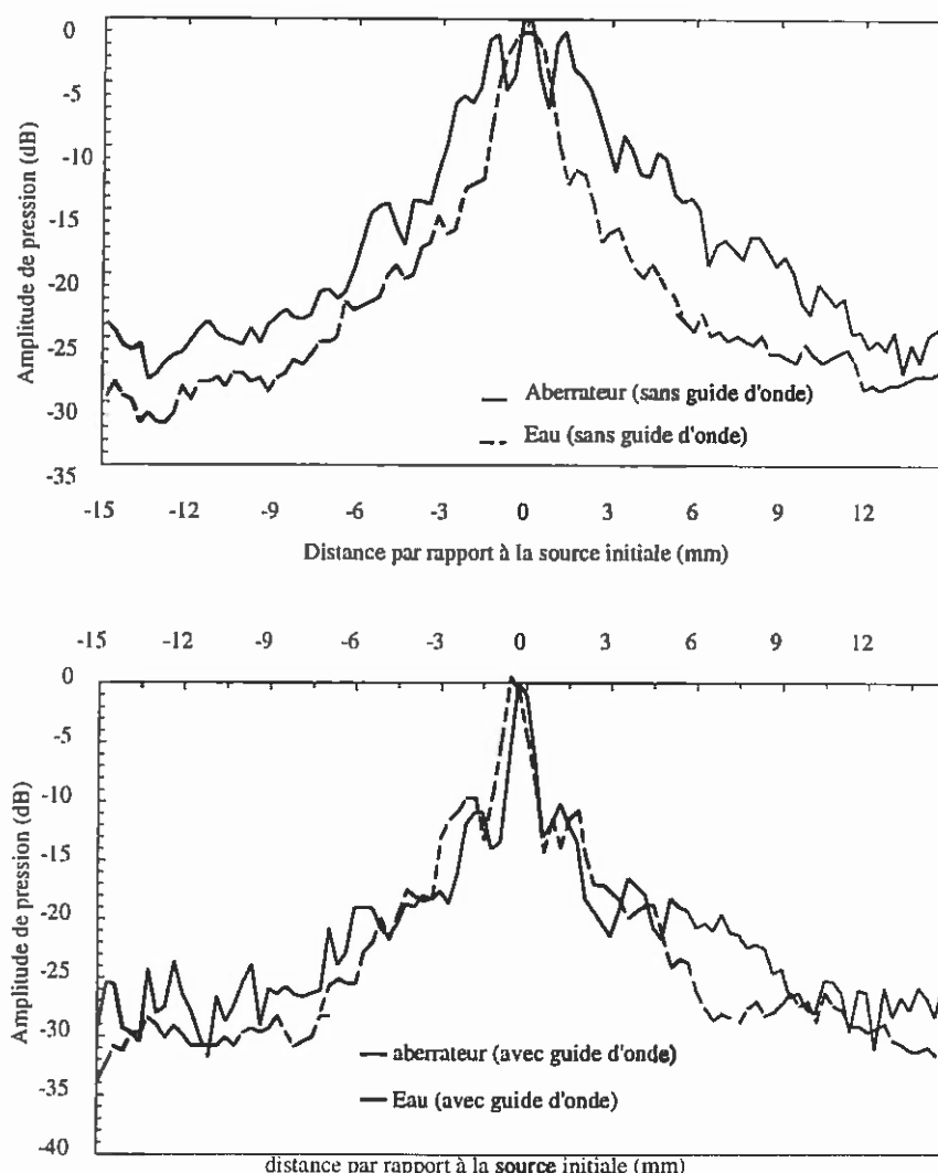
Figure 70. Diagramme de focalisation expérimentaux obtenus à travers l'aberrateur avec et sans parois réfléchissantes. Comparaison avec les diagrammes de focalisation optimaux obtenus dans l'eau, à la fois avec et sans parois réfléchissantes.
