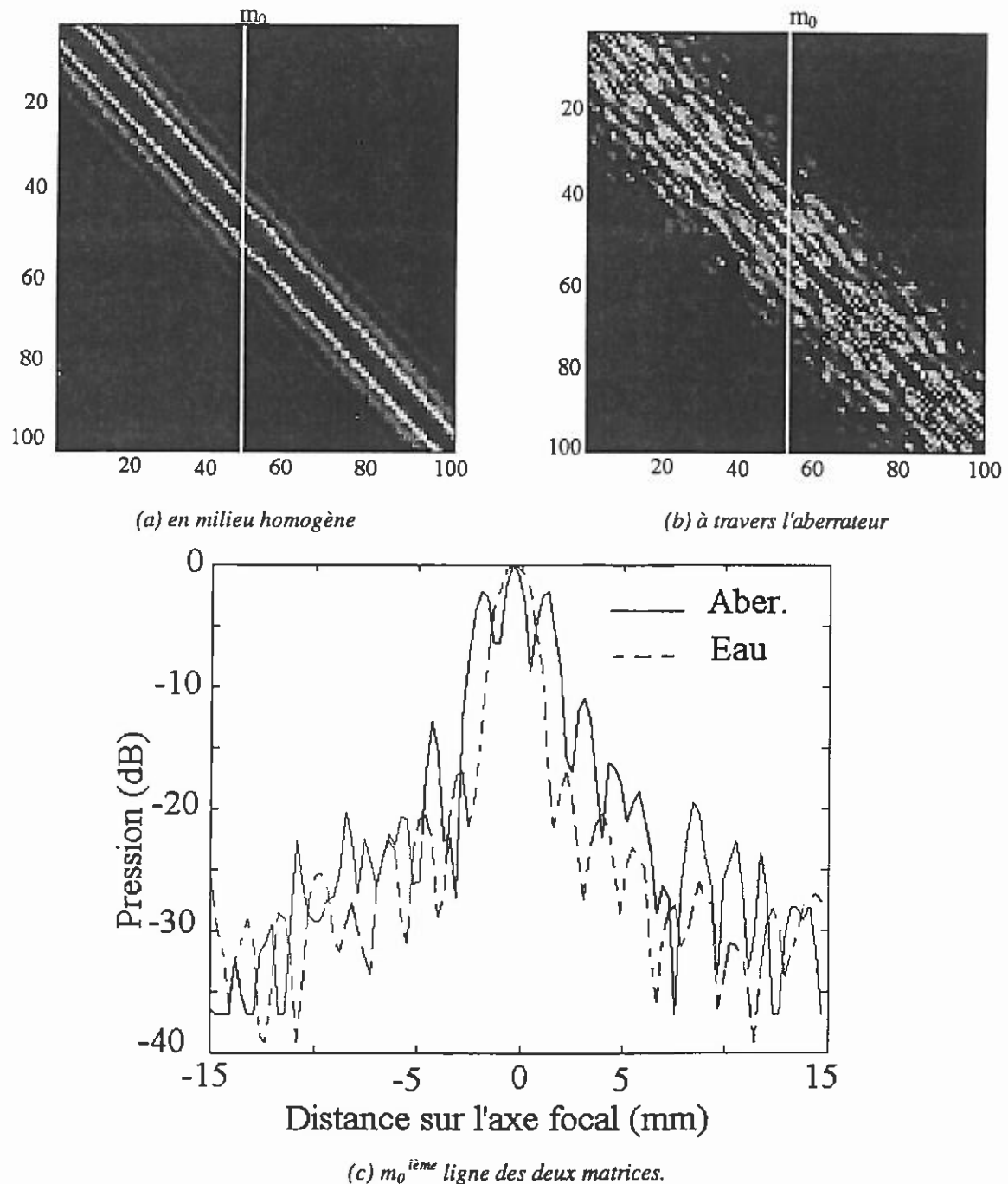
Figure 61. Expérience à travers un aberrateur non dissipatif et fortement diffractant : Représentation de l'amplitude de la matrice \mathbf{H}^t \mathbf{H}^* , (a) en milieu homogène, (b) à travers l'aberrateur. Les axes verticaux et horizontaux correspondent au numéro du point de contrôle dans le plan focal. En (c), la m_0^{\text{ième}} colonne de chaque matrice correspondant aux diagrammes de focalisation que l'on obtiendrait dans les deux cas en appliquant le processus de focalisation par retournement temporel à une source initialement située en S = m_0 dans le plan de contrôle.
