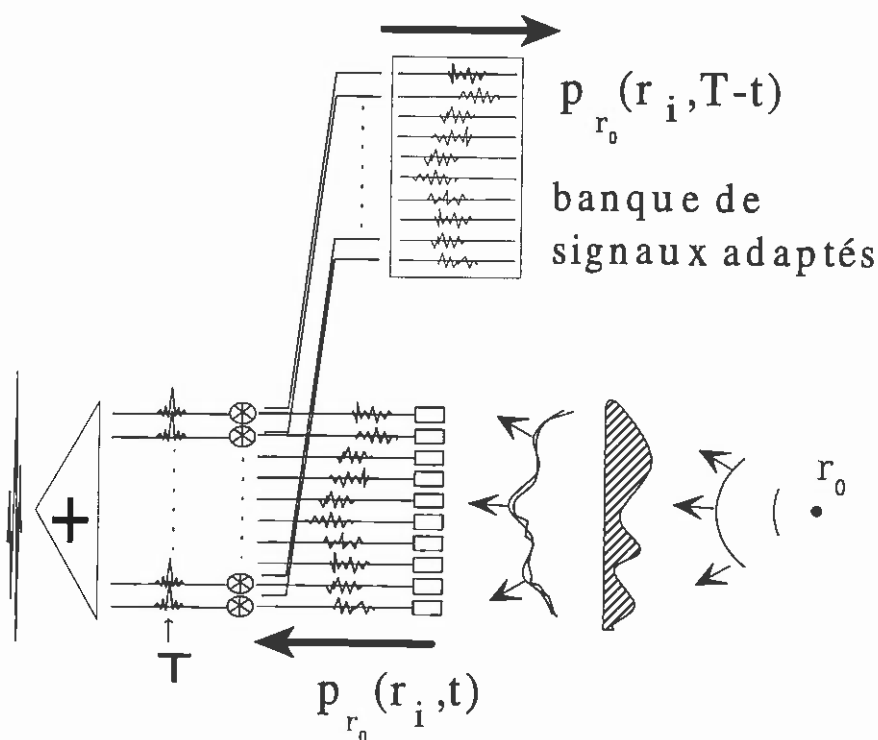
Fig. II.II Séquence complète de focalisation en émission-réception. La banque de signaux adaptés est utilisée initialement pour focaliser en émission. Elle est sauvegardée dans des mémoires extérieures au MRT. En réception, quand un écho est effectivement rétrodiffusé par le réflecteur, les signaux reçus sont convolués avec ceux de la banque adaptée pour produire un ensemble de signaux ayant tous leur maximum au même instant. Leur sommation est alors pleinement constructive.
