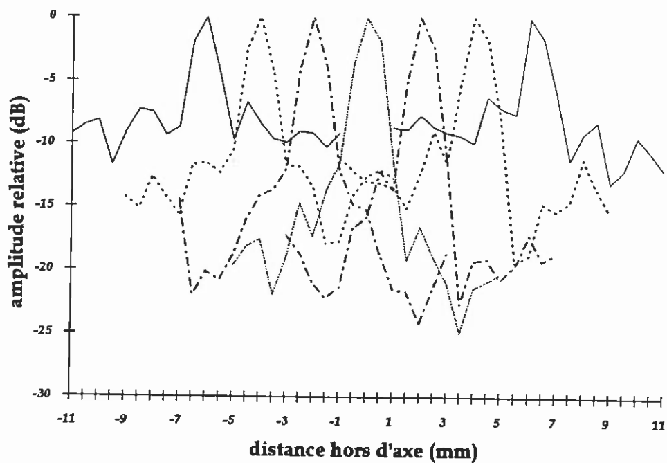
Fig. III.4 Diagrammes de directivité obtenus par inclinaison de la banque de données initiale adaptée au point r_0 situé sur l'axe. La focalisation reste correcte jusqu'à 2 mm autour de cette position. Au delà, les lobes secondaires remontent sévèrement. Ceci illustre l'effet très limitatif de l'angle isoplanétique dans les milieux modélisés par des aberrations de phase distantes du réseau de transducteurs.
