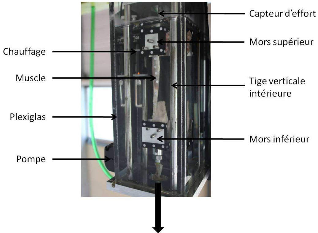
Figure 52 : Montage expérimental en place sur le vérin hydraulique, Photographie
