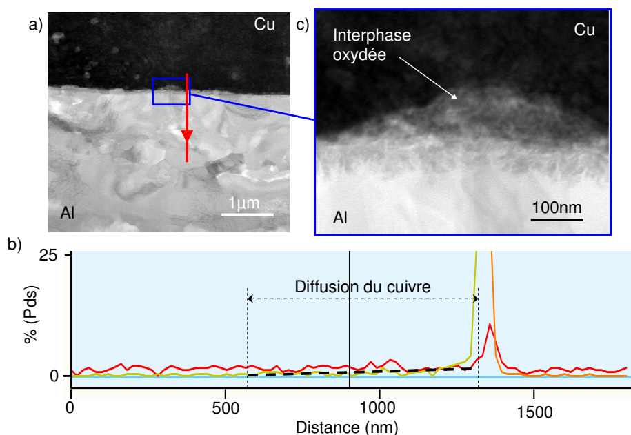
Figure V-18 : a) et c) Images STEM* en fond clair de la zone interfaciale, au fond de la particule projetée à 380\text{m.s}^{-1} et b) analyse par profil EDX* à travers l'interface b)
