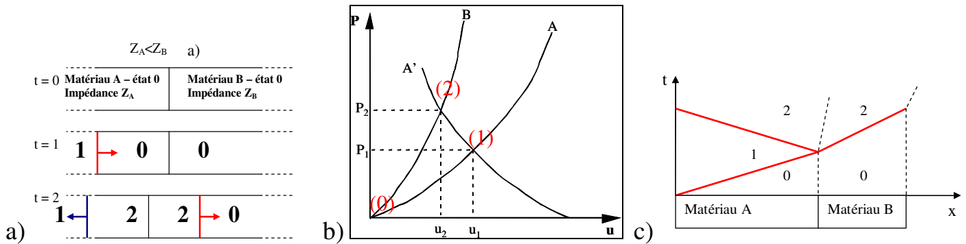
Figure I-6 : a) et c) Schéma de la propagation des ondes aux interfaces, b) polaires de choc
