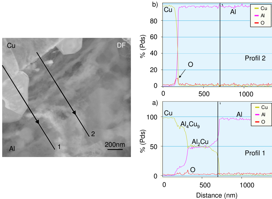
Figure V-10 : Image STEM en fond noir de la zone interfaciale, dans la zone intermédiaire, d'une particule projetée à 380\text{m.s}^{-1} avec a) et b) analyses chimiques par profil EDX*
