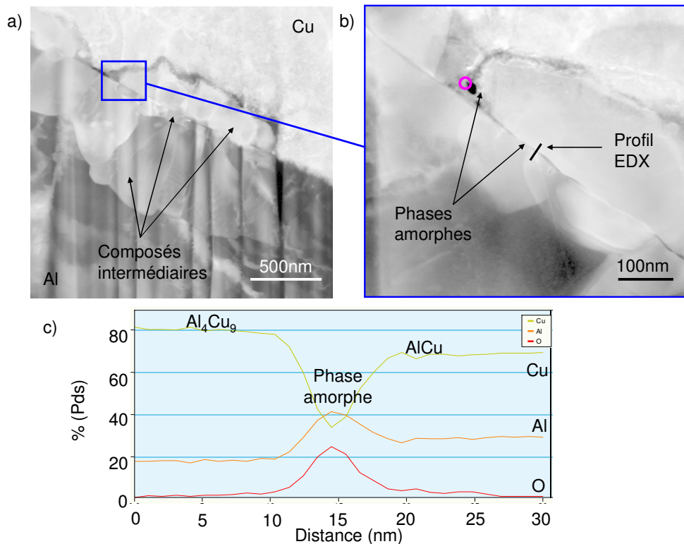
Figure V-12 : a) et b) Images STEM* en fond clair de la zone interfaciale, dans la zone intermédiaire, d'une particule ayant impacté à 480m.s -1 avec c) analyse chimique par profil EDX* de l'interphase centrale
