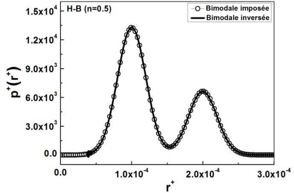
Figure 3.30. : Comparaison entre la DTP initiale et celle calculée pour une distribution bimodale avec m_2 = 2m_1 et le même \sigma pour un fluide de Herschel-Bulkley ( n = 0,5 ).
