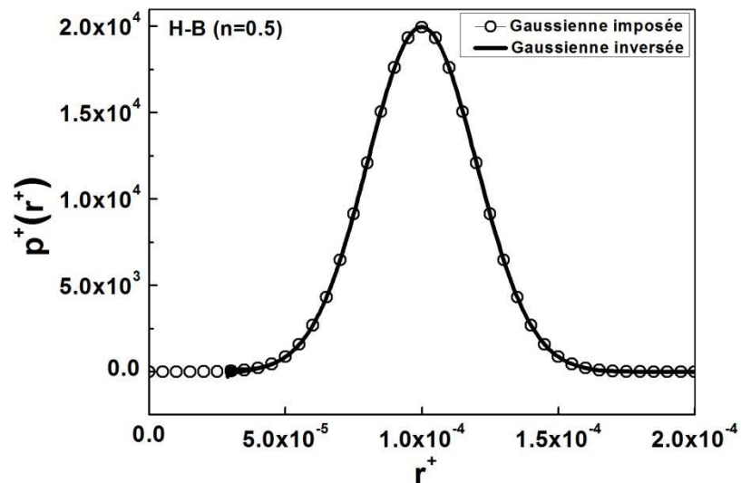
Figure 3.26. : Comparaison entre la DTP initiale et celle calculée pour une distribution gaussienne en utilisant un fluide de Herschel-Bulkley pour ( n=0,5 ).
