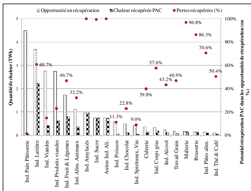
Fig. 64 : Potentiel de récupération des PACs dans les sous secteurs de l'industrie agroalimentaire à l'horizon 2020.
