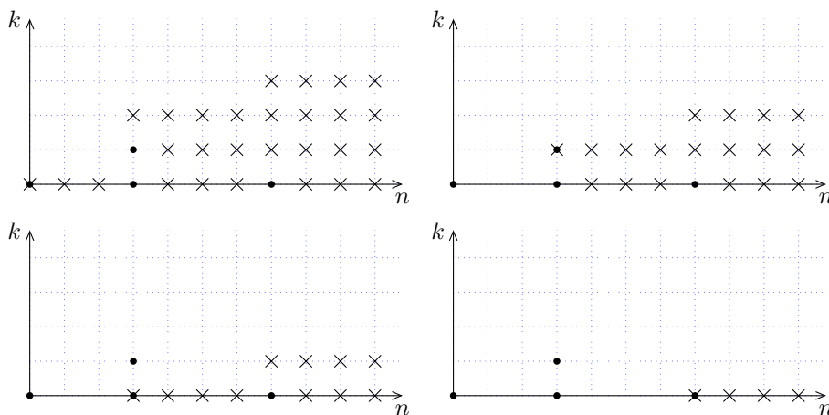
Figure 4.2. Support des solutions de la base canonique, pour une équation différentielle générique de polynôme indicial n(n-3)^2(n-7) . Les croix représentent les coefficients non nuls (sauf pour certaines équations exceptionnelles) ; les points, les coefficients arbitraires où se placent les conditions initiales.
